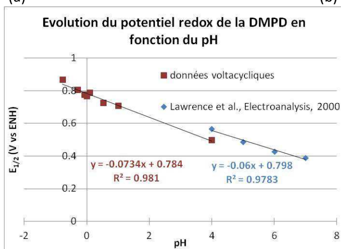
Figure 45 : Relation entre le pH est le potentiel redox de la DMPD. (a) Voltampérométrie obtenus pour la DMPD à différentes concentrations d'HCl ; (b) Détermination du potentiel redox de la DMPD à partir des voltampérométries de (a) ;(c) Comparaison de la relation potentiel – pH de la DMPD issue de la littérature [180] avec celle obtenue à partir des valeurs expérimentales de voltampérométrie cyclique.
