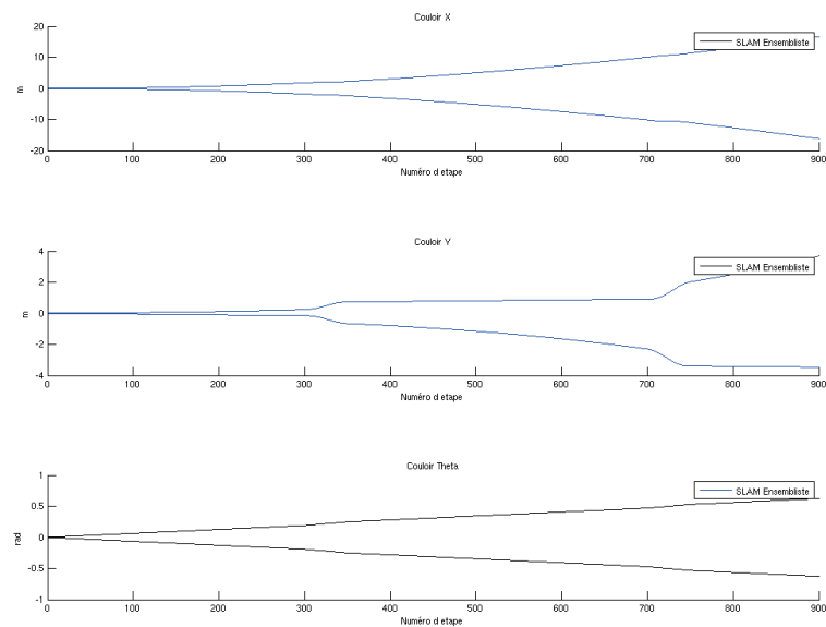
(b) Couloir d'incertitude incluant des incertitudes sur les constantes
