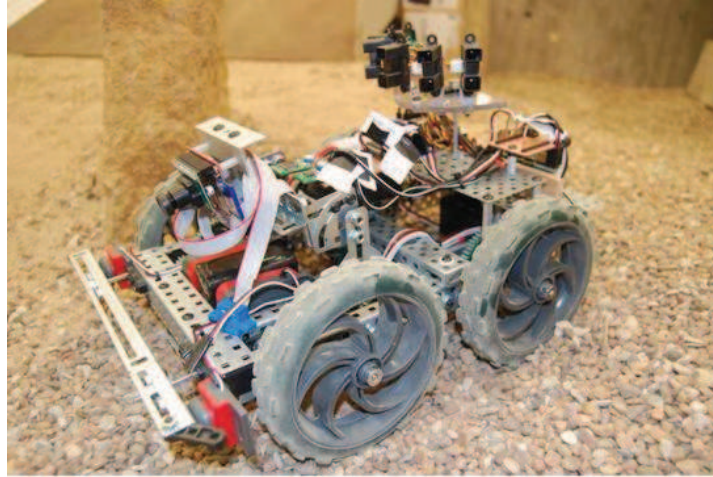
FIGURE 1.5: Robot d'exploration conçu par Gifford et al. [5]
