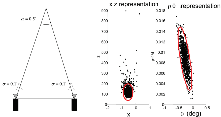
FIGURE 1.2: Comparaison entre une paramétrisation classique et par inverse de profondeur par Montiel et al. [2]
