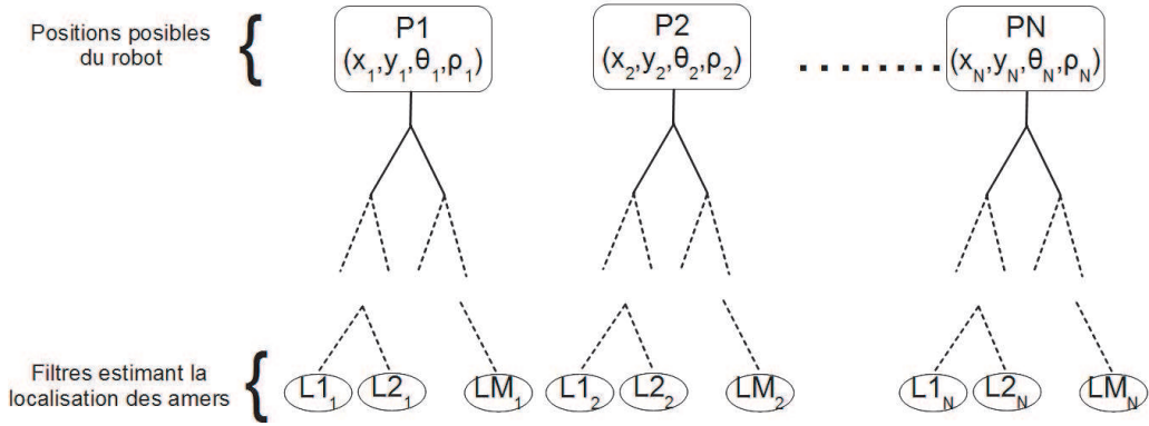
FIGURE 4.1: Représentation du FastSLAM
