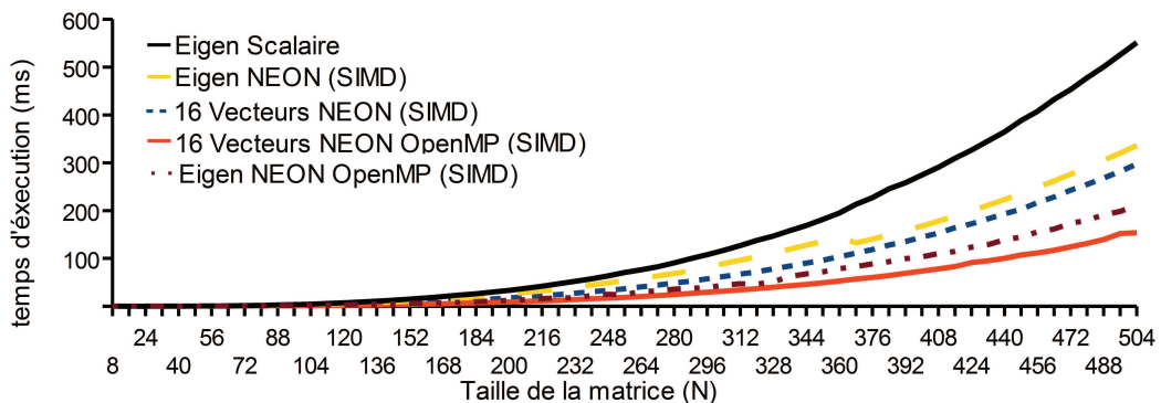
Figure 3.9: Temps d'exécution de la multiplication matricielle sur les deux cœurs de l'OMAP4430
