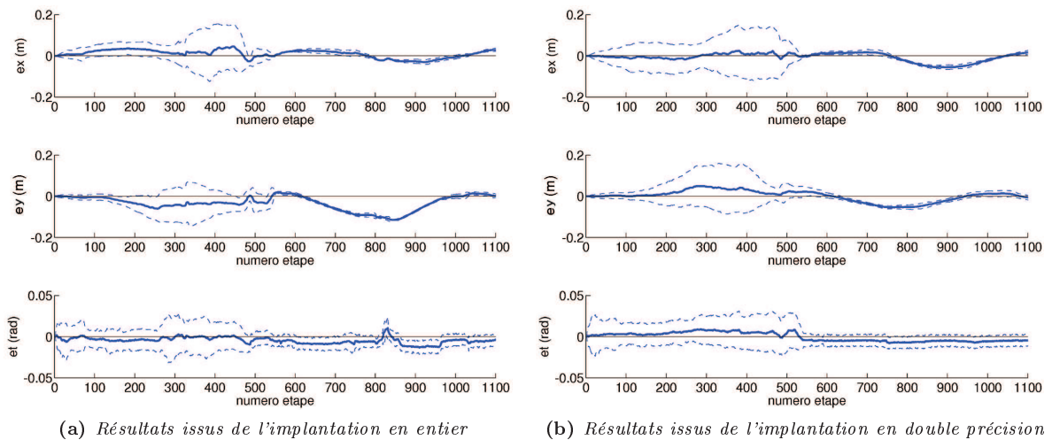
FIGURE 4.26: Couloir d'incertitude sur la position du mobile - Comparaison avec l'implantation en double précision
