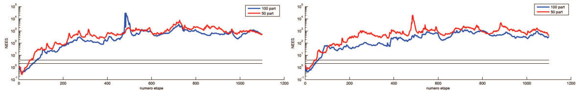
(e) NEES de la position x , y , \theta pour l'environnement 2 rempli de 100 amers
