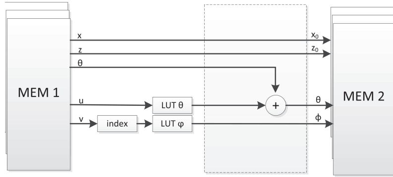
FIGURE 4.16: Architecture du bloc fonctionnel "Initialisation d'un amer"
