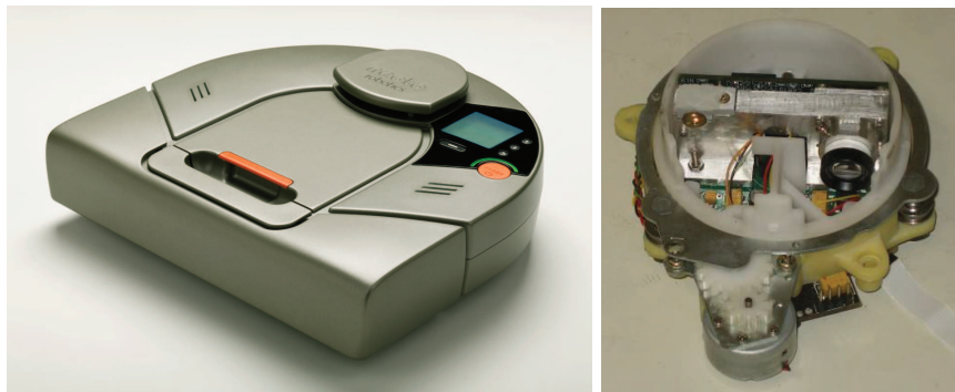
FIGURE 1: Aspirateur autonome développé par Neato, et son laser low-cost
