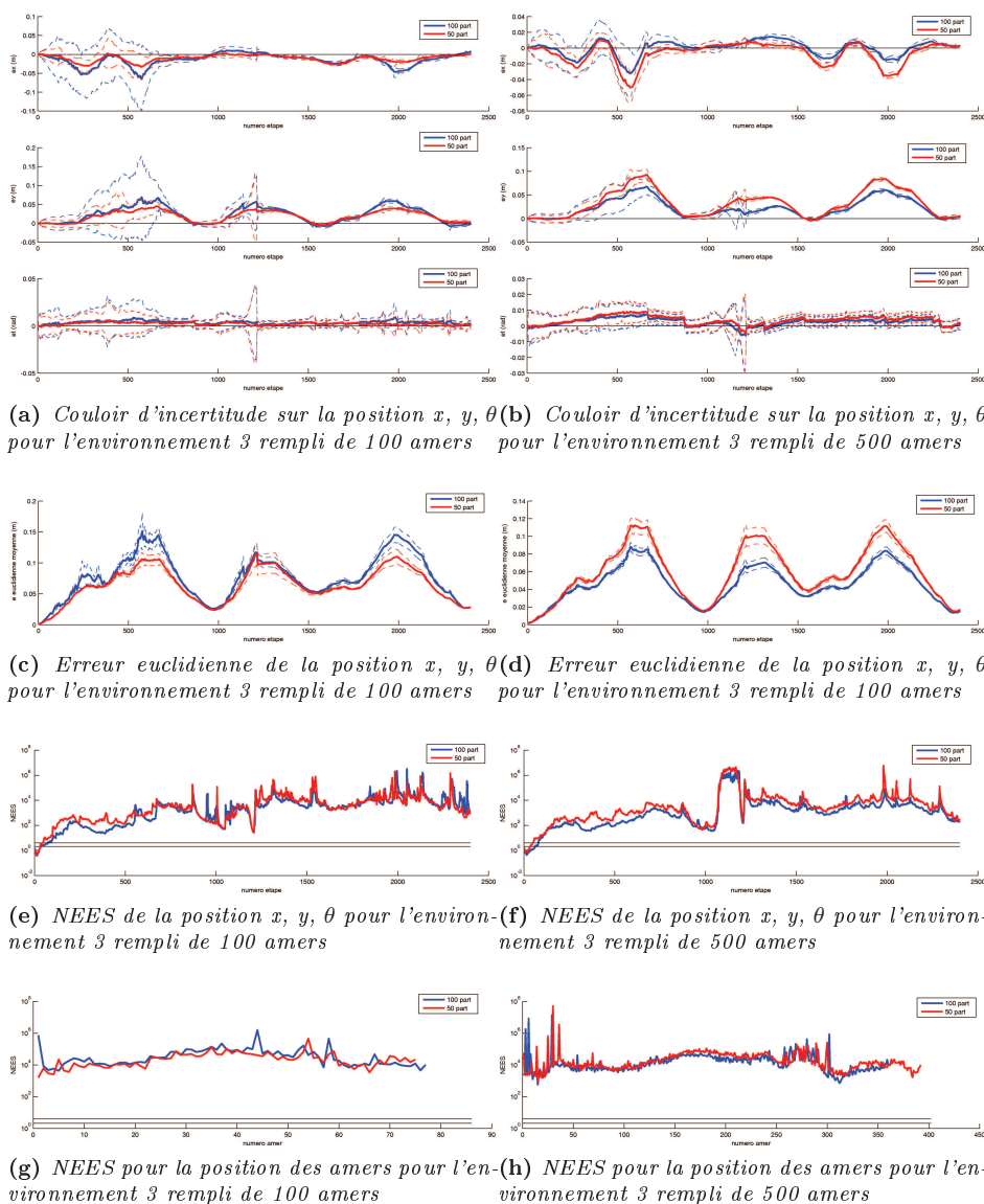
FIGURE 6.4: Résultats du FastSLAM pour l'environnement 3
