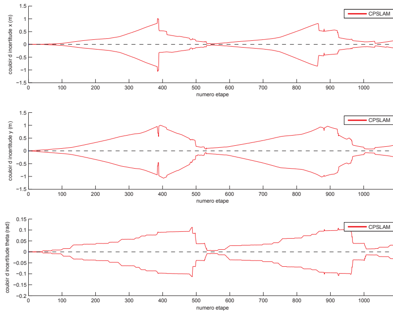
Figure 5.13: Couloir d'incertitude du SLAM ensembliste
