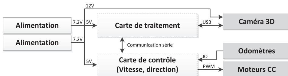
FIGURE 2.2: L'architecture du système embarqué par MiniB
