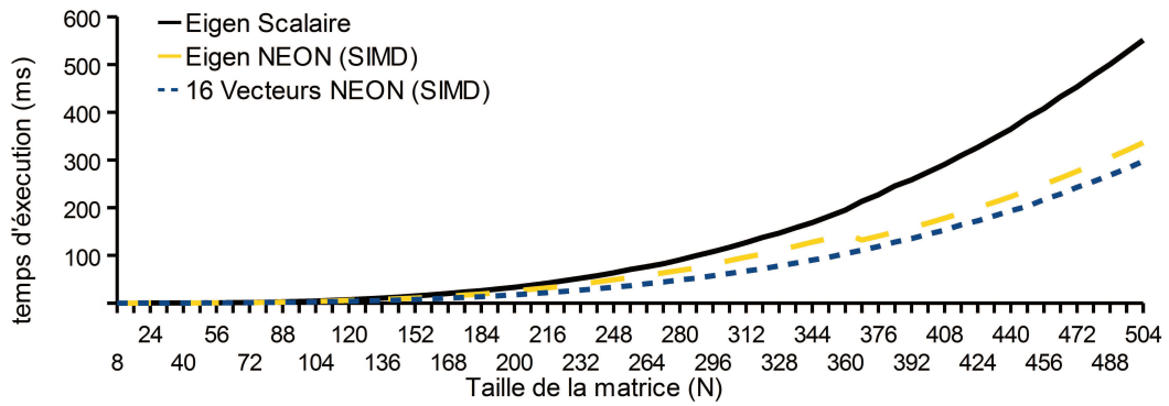
Figure 3.8: Temps d'exécution de la multiplication matricielle sur le processeur Cortex A9 et le coprocesseur NEON
