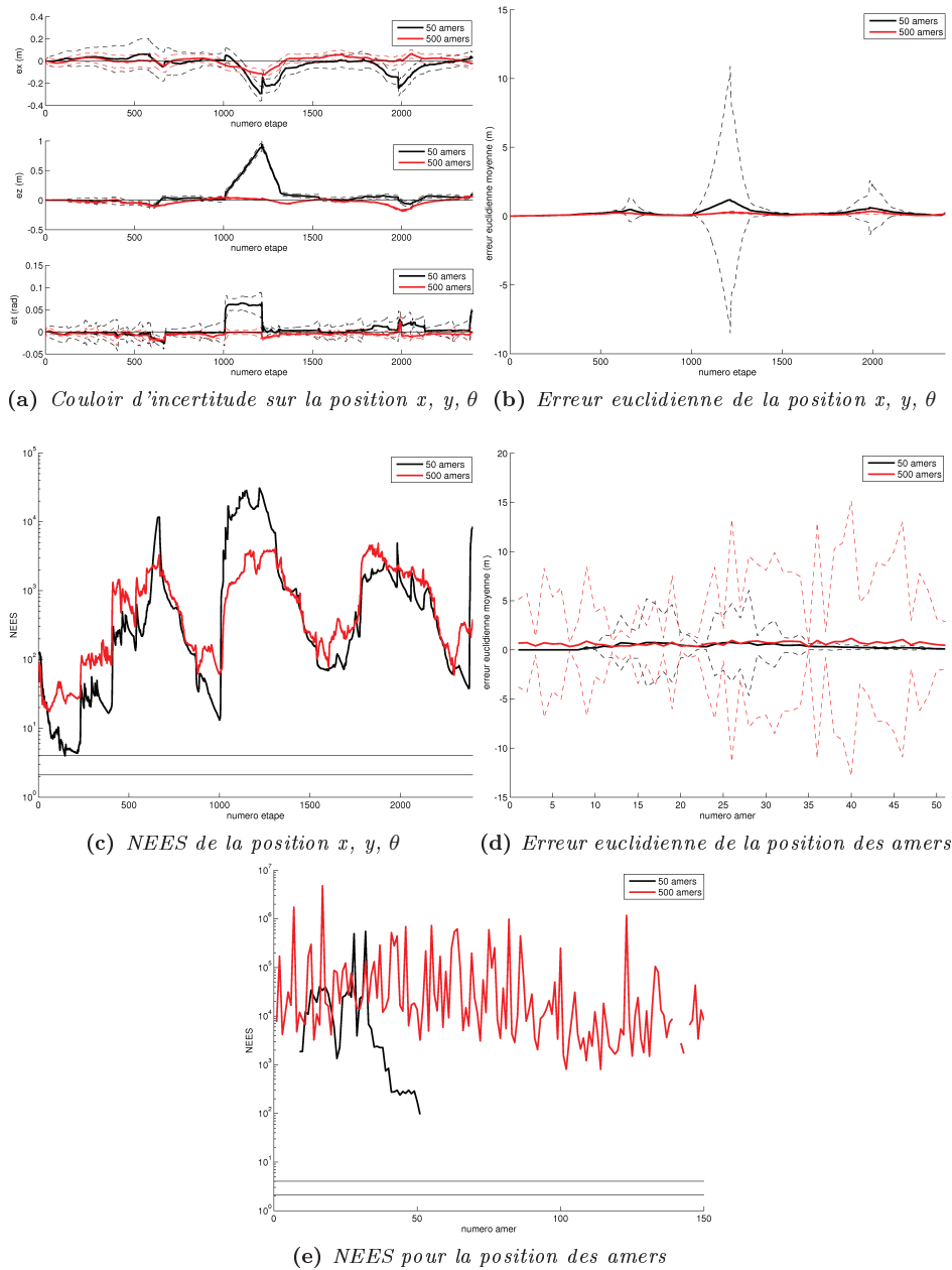
FIGURE 6.2: Résultats de l'EKF-SLAM pour l'environnement 3
