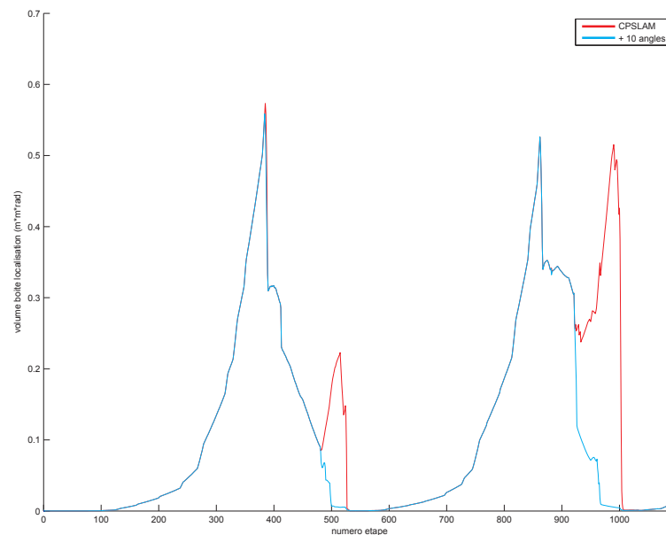
Figure 5.17: Comparaison entre le volume de la boîte de localisation avec et sans inclinaison de repère
