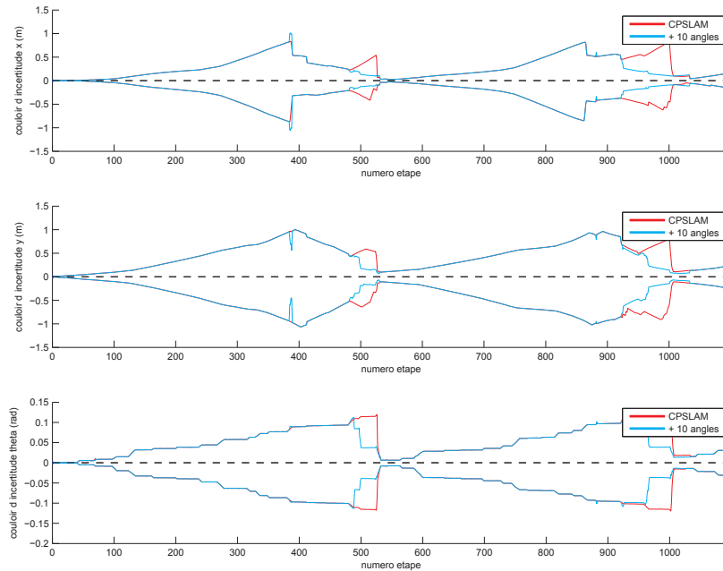
Figure 5.16: Comparaison entre les couloirs d'incertitudes avec et sans inclinaison de repère
