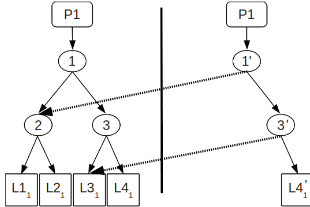
FIGURE 4.4: Mise à jour de l'amer 4 pour la particule 1
