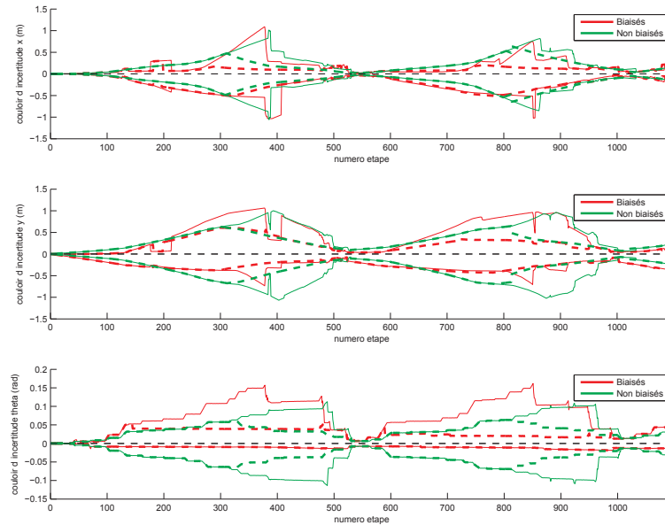
Figure 5.22: Couloir d'incertitude en incluant un biais sur les paramètres du modèle de déplacement
