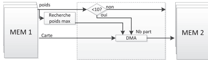
FIGURE 4.20: Architecture du bloc fonctionnel “Rééchantillonnage”
