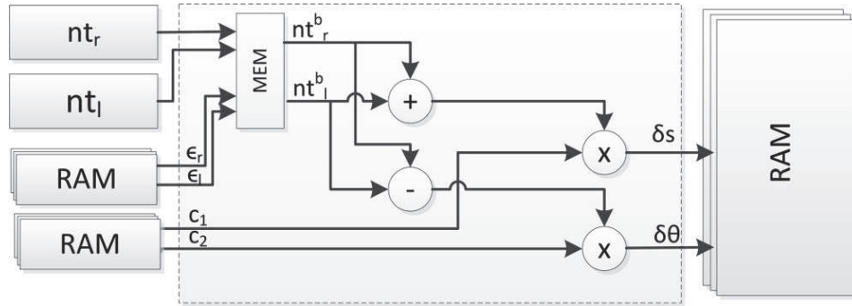
FIGURE 4.14: Architecture du bloc fonctionnel "Calcul déplacement"
