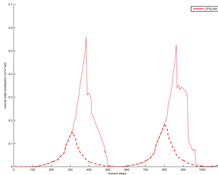
Figure 5.19: Volume de la boîte de localisation et post localisation pour l'environnement 2
