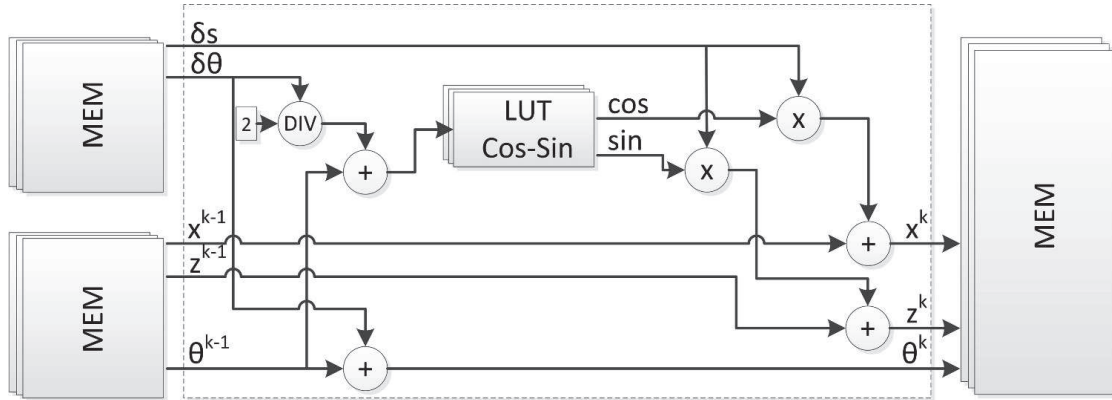
FIGURE 4.15: Architecture du bloc fonctionnel "Modèle déplacement"
