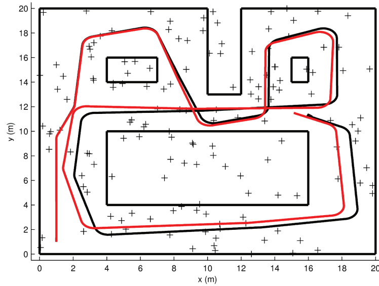
Figure 2.12: Trajectoire odométrique bruitée
