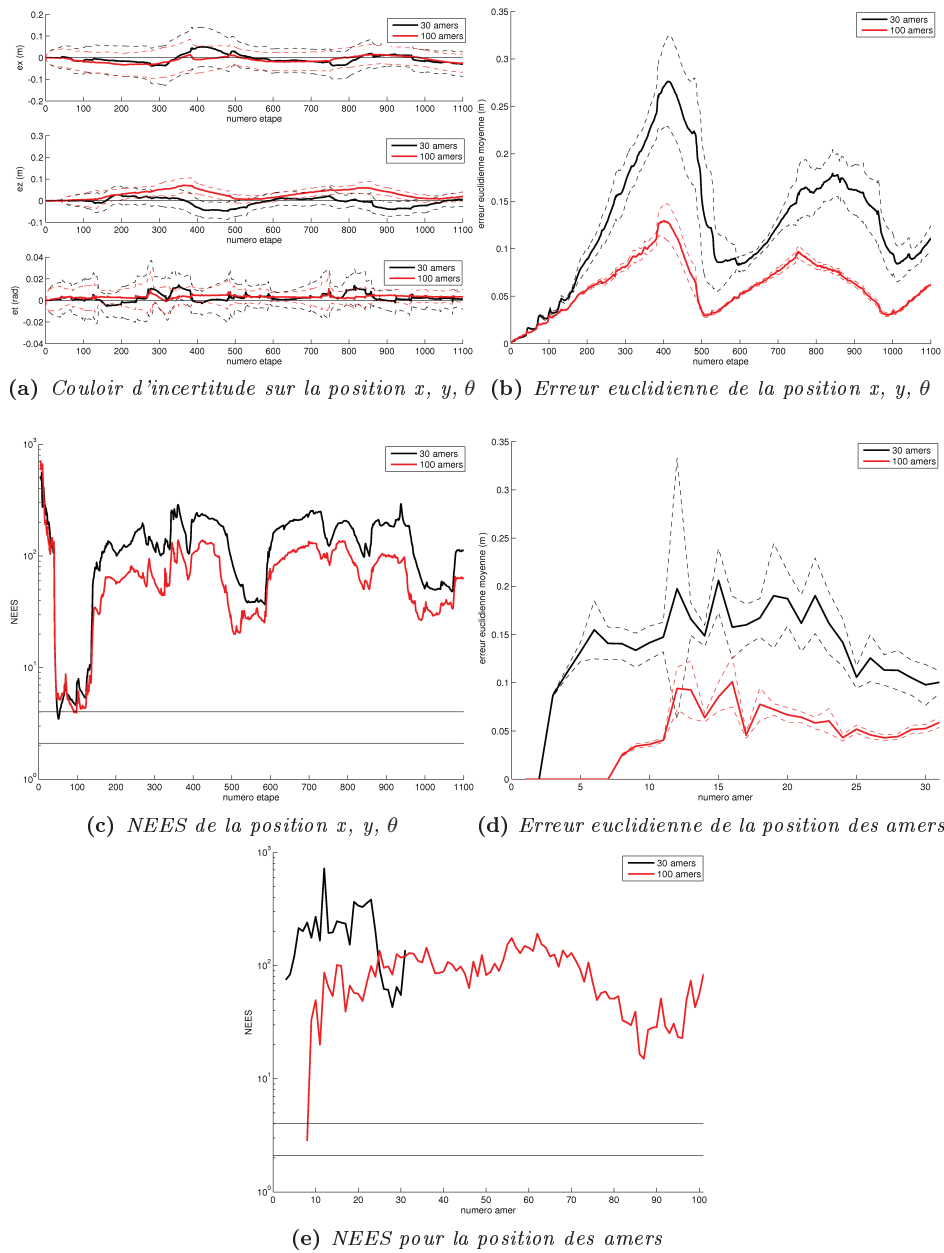
FIGURE 6.1: Résultats de l'EKF-SLAM pour l'environnement 2
