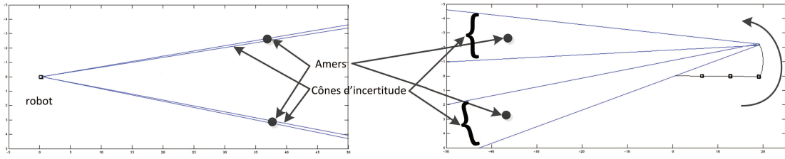
Figure 5.9: Initialisation d'amers avec et sans incertitude d'orientation du mobile
