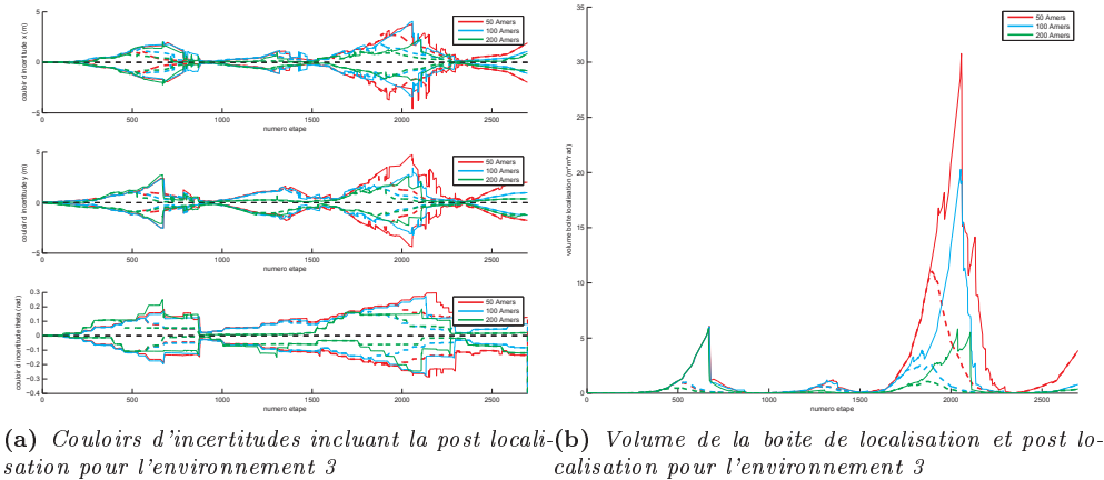
Figure 6.6: Résultats expérimentaux du SLAM ensembliste pour l'environnement 3
