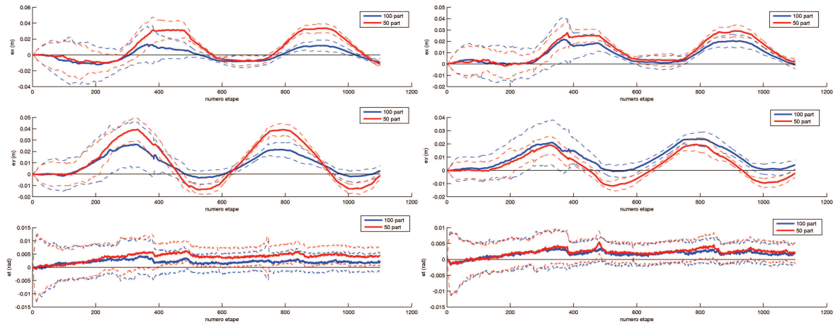
(a) Couloir d'incertitude sur la position x , y , \theta pour l'environnement 2 rempli de 100 amers
