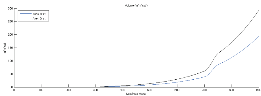
Figure 5.5: Volume de la boîte de localisation
