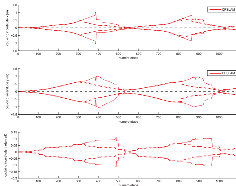
Figure 5.18: Couloirs d'incertitudes incluant la post localisation pour l'environnement 2
