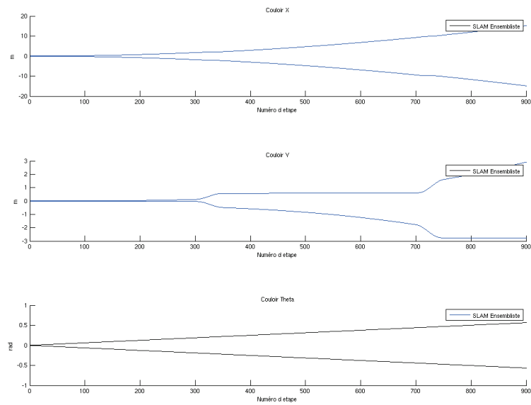
(a) Couloir d'incertitude sans incertitude sur les constantes
