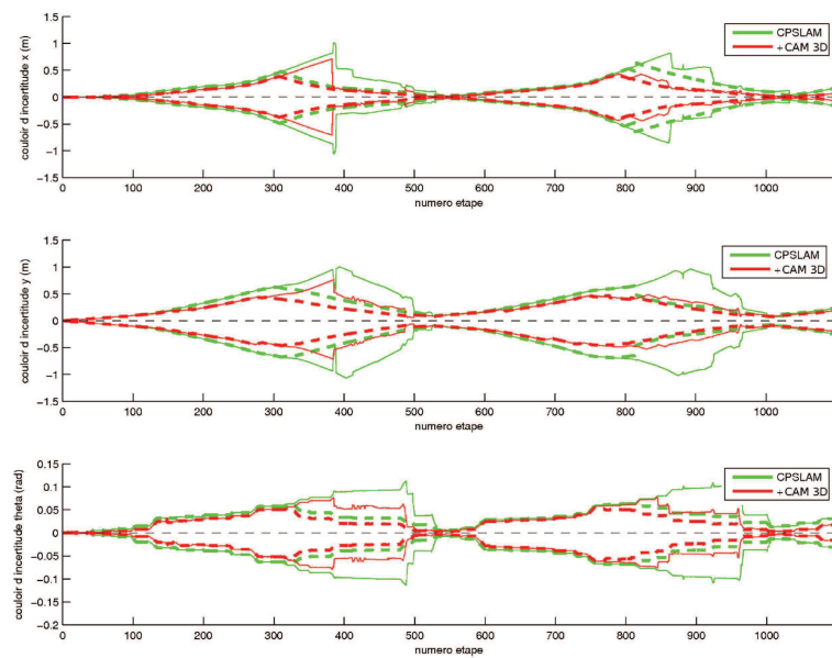
Figure 5.26: Couloir d'incertitude en utilisant un caméra 3D
