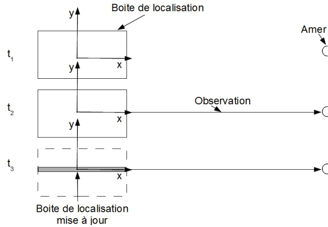
Figure 5.11: Correction de la boîte de localisation dans le cas 2D
