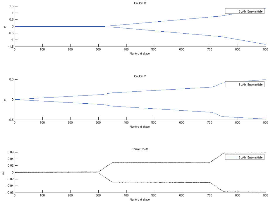
Figure 5.7: Couloir d'incertitude avec des incertitudes sur les constantes
