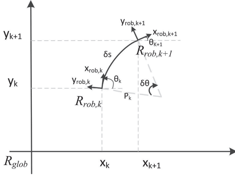
FIGURE 2.6: Définition de \delta s et \delta \theta
