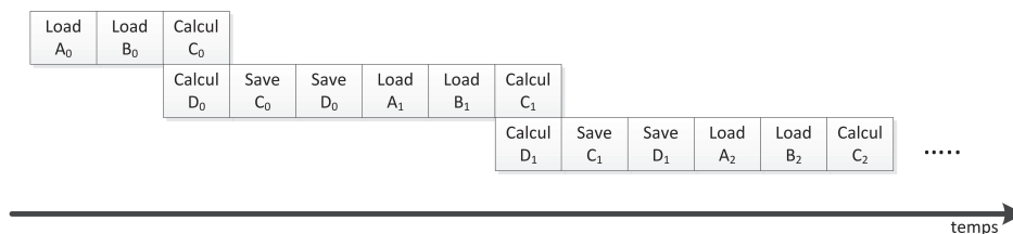
FIGURE 4.12: Diagramme temporel de l'exécution avec calculs parallèles
