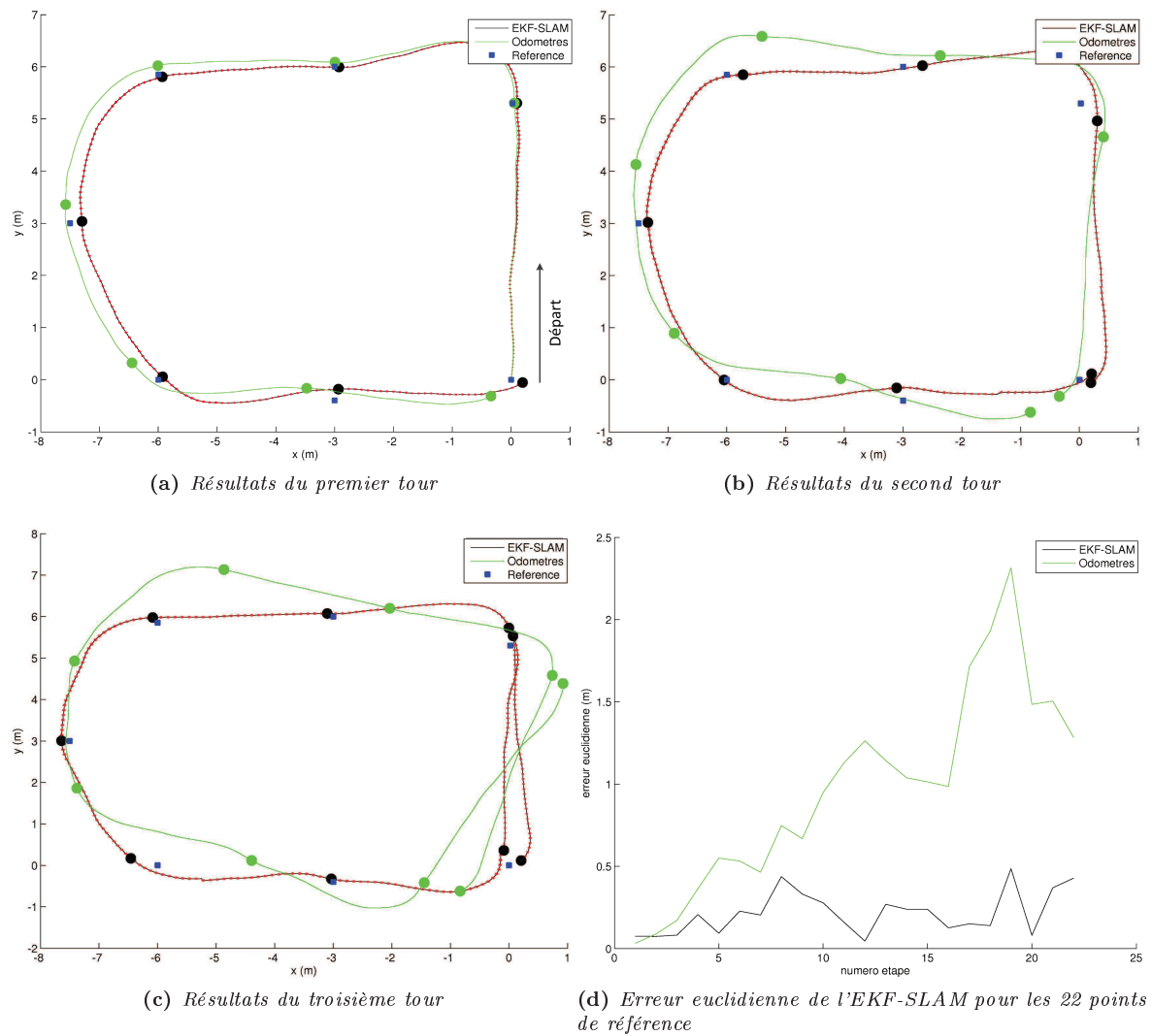
FIGURE 3.4: Résultats expérimentaux de l'EKF-SLAM
