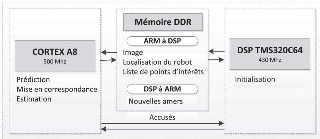
Figure 3.10: ARM-DSP mémoire partagée
