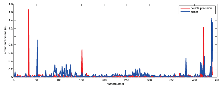
FIGURE 4.24: Erreur euclidienne sur la position des amers - Comparaison avec l'implantation en double précision
