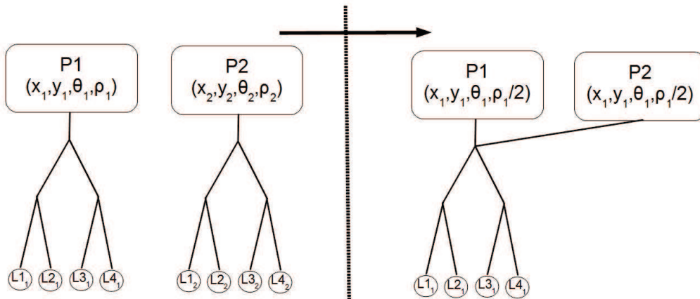
FIGURE 4.5: Réchantillonnage de la Particule 2 à partir de la Particule 1
