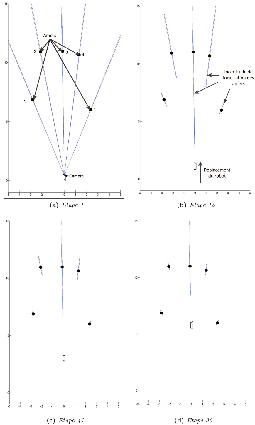
Figure 5.12: Evolution de la carte de l'environnement
