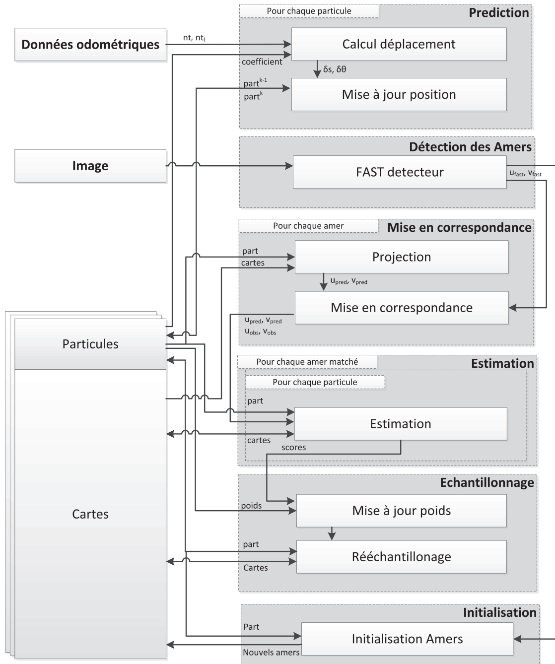
FIGURE 4.6: Algorithme FastSLAM sous forme de bloc fonctionnel
