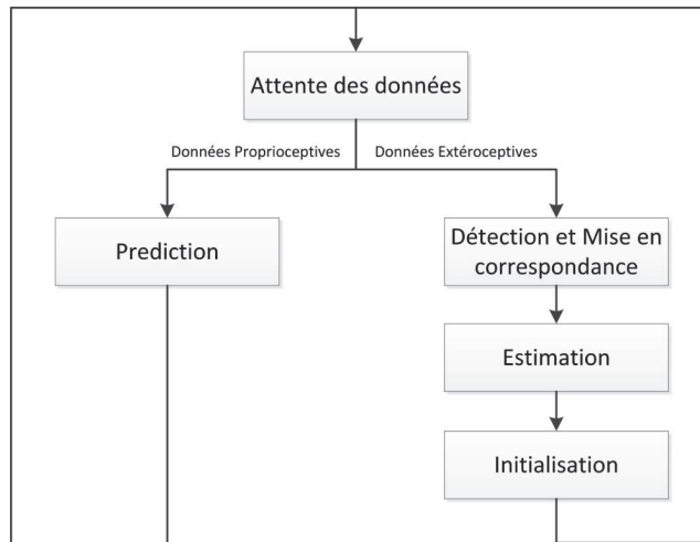
FIGURE 3.1: Algorithme SLAM Générique
