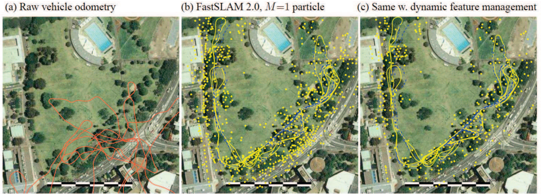
FIGURE 1.3: Résultats du FastSLAM de Montemerlo et al. [3] pour le jeu de données de Victoria Park
