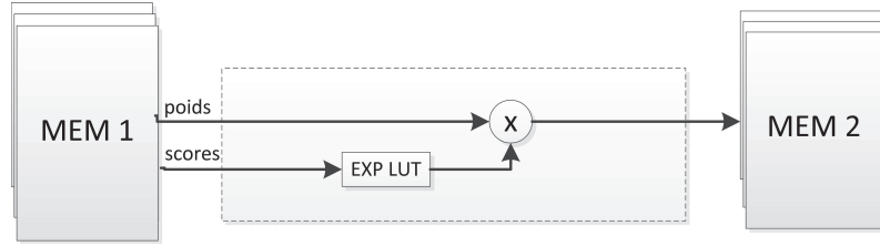
FIGURE 4.19: Architecture du bloc fonctionnel "Mise à jour des poids"
