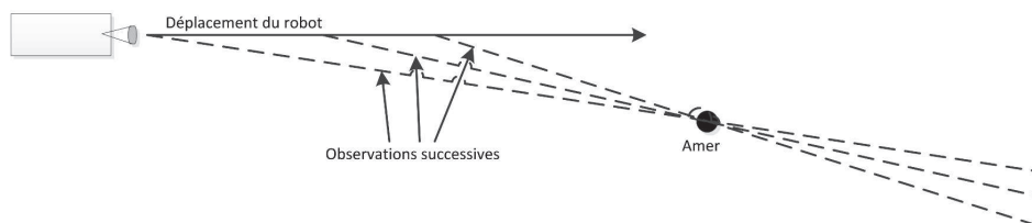
FIGURE 3.2: Initialisation des amers par la méthode de Davison.
