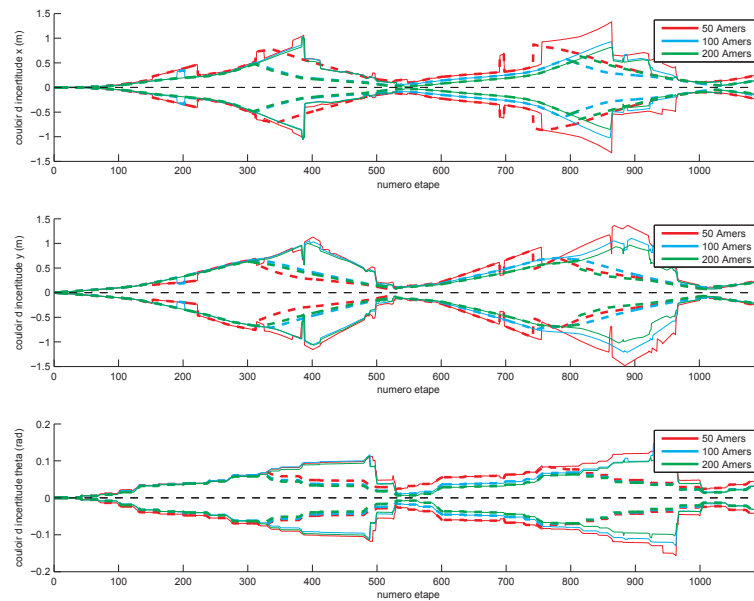
Figure 5.20: Couloirs d'incertitudes incluant la post localisation pour l'environnement 2 en fonction du nombre d'amers
