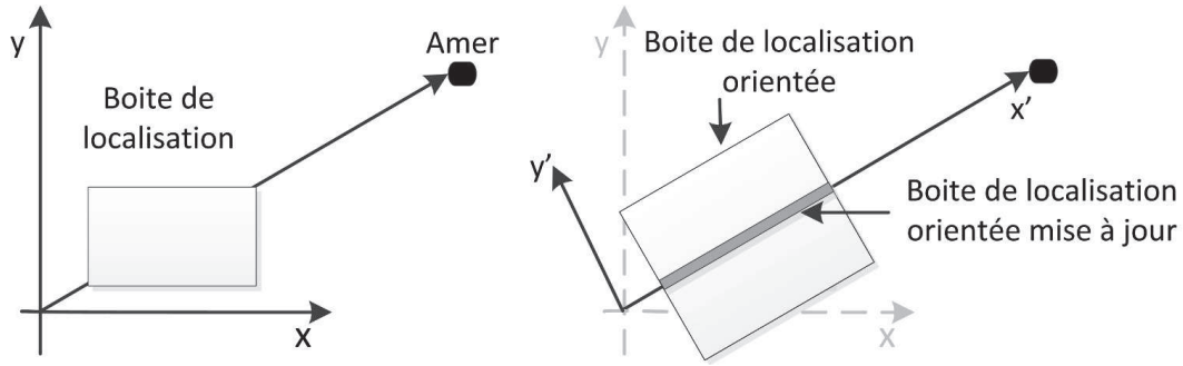
Figure 5.15: Correction de la boîte de localisation en utilisant un repère orienté
