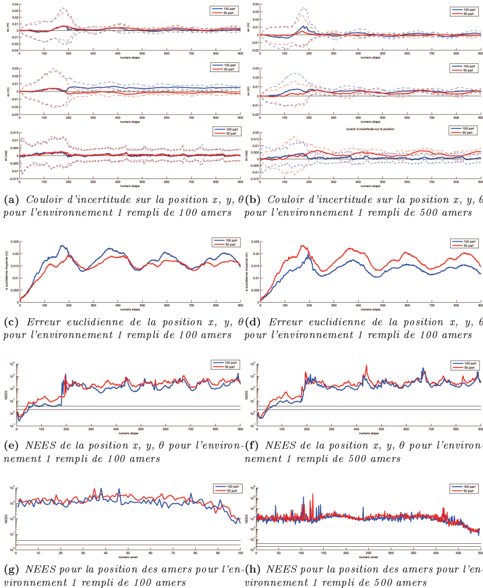
FIGURE 6.3: Résultats du FastSLAM pour l'environnement 1
