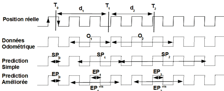
Figure 5.6: Amélioration de la gestion des données odométriques
