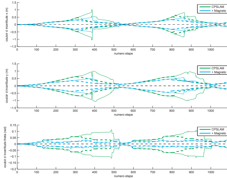
Figure 5.28: Couloir d'incertitude en utilisant un magnétomètre
