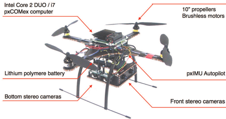
FIGURE 1.7: Drône quadrirotor conçu par Pixhawk [7]
