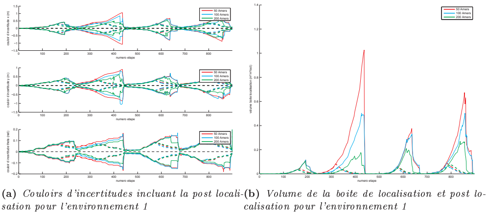
Figure 6.5: Résultats expérimentaux du SLAM ensembliste pour l'environnement 1
