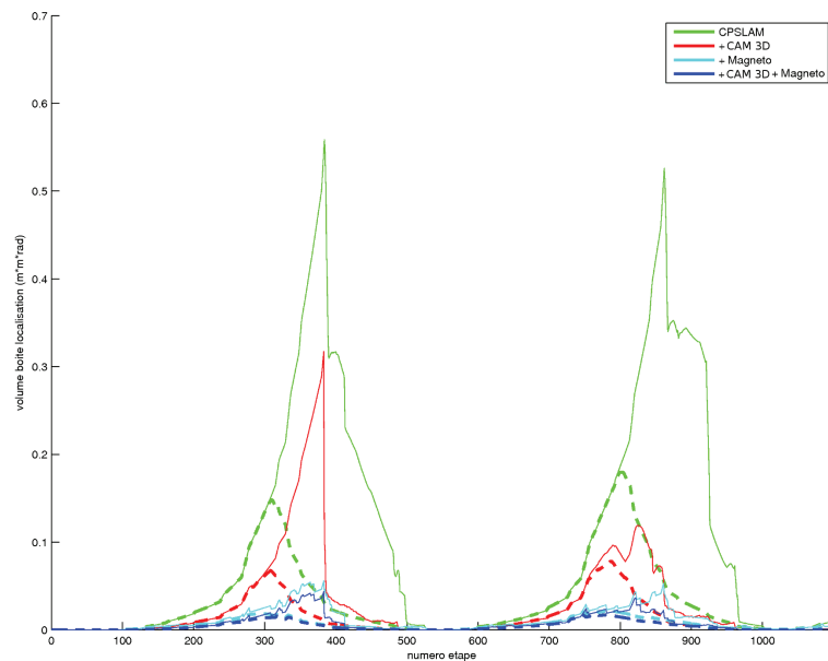
Figure 5.31: Volume de la boîte de localisation en utilisant l'ensemble des capteurs
