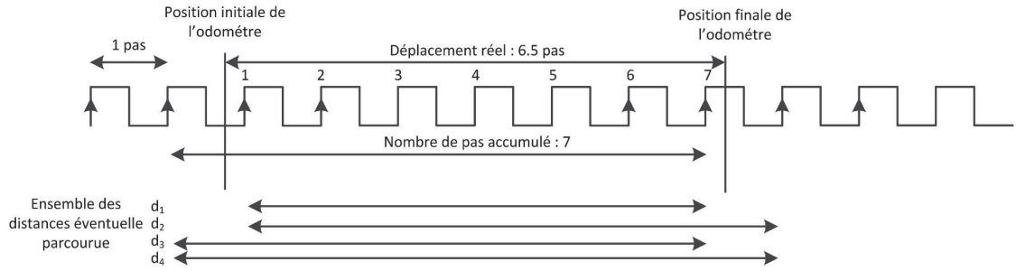
Figure 5.1: Utilisation des données odométriques
