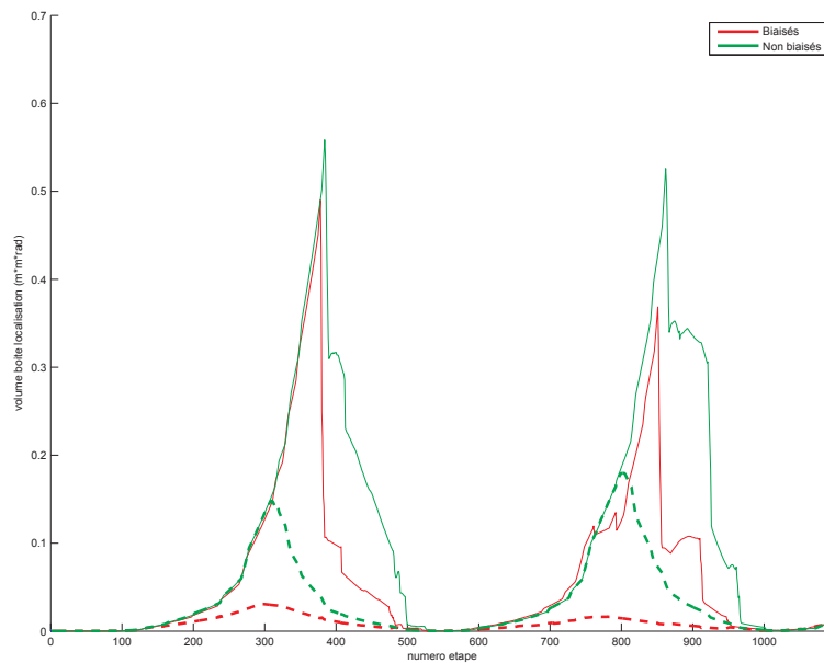
Figure 5.23: Volume de la boîte de localisation en incluant un biais sur les paramètres du modèle de déplacement
