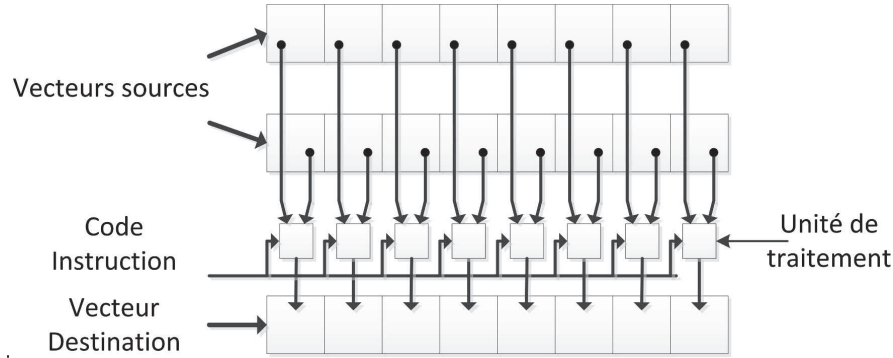
Figure 3.7: Traitement des données par le coprocesseur vectoriel NEON
