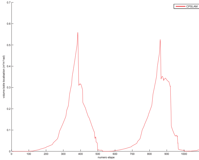
Figure 5.14: Volume de la boîte de localisation du SLAM ensembliste
