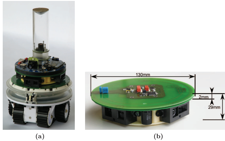
FIGURE 1.6: a) Robot conçu par Magnenat et al. [6], b) Capteur développé
