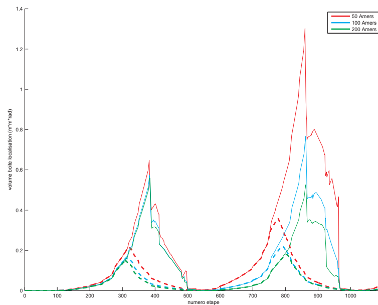
Figure 5.21: Volume de la boite de localisation et post localisation pour l'environnement 2 en fonction du nombre d'amers
