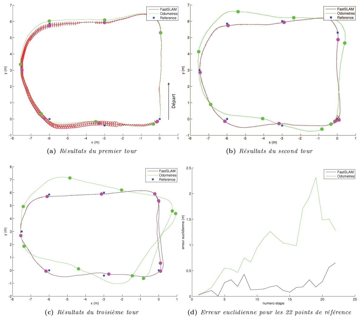
FIGURE 4.8: Résultats expérimentaux du FastSLAM
