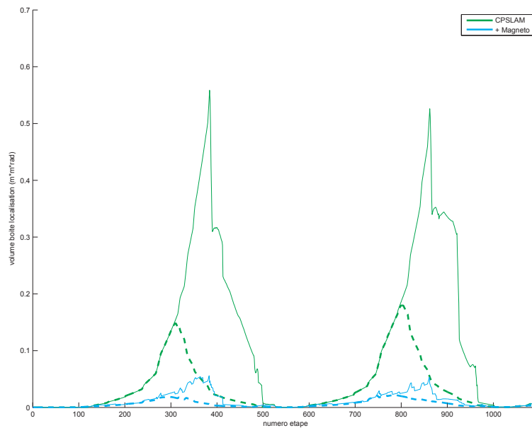
Figure 5.29: Volume de la boîte de localisation en utilisant un magnétomètre
