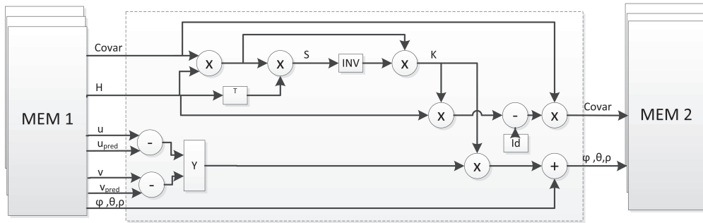
FIGURE 4.18: Architecture du bloc fonctionnel "Estimation de la localisation d'un amer"
