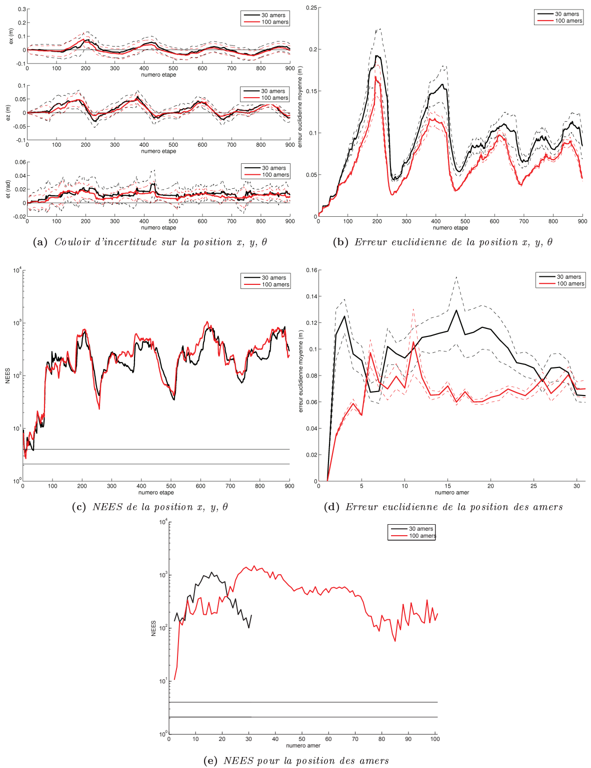
FIGURE 3.3: Résultats de l'EKF-SLAM pour l'environnement 1
