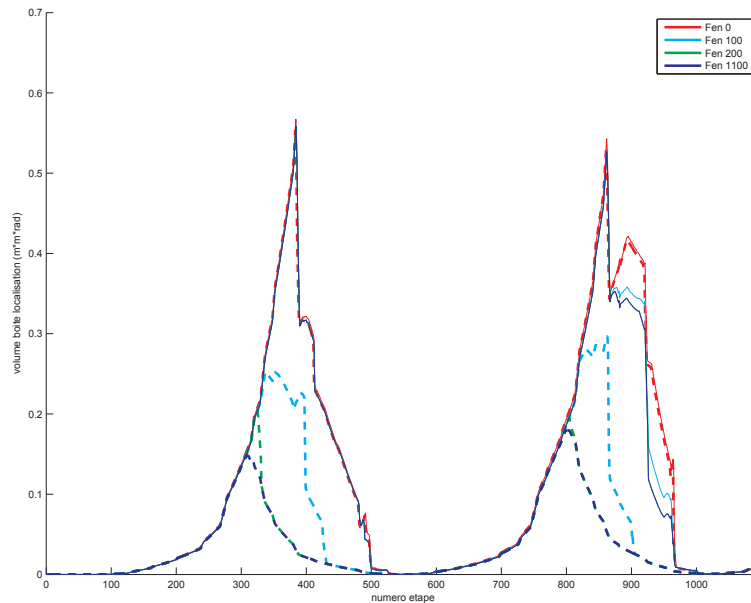
Figure 5.24: Comparaison entre le volume de la boîte de localisation en utilisant différentes tailles de fenêtre de propagation
