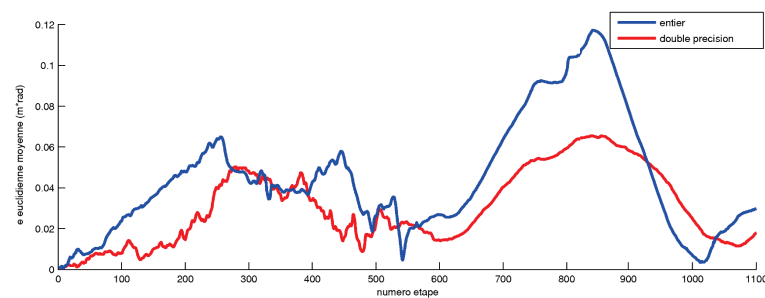
FIGURE 4.25: Erreur euclidienne sur la position du mobile - Comparaison avec l'implantation en double précision
