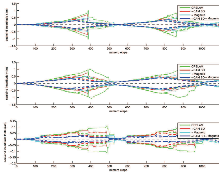
Figure 5.30: Couloir d'incertitude en utilisant l'ensemble des capteurs
