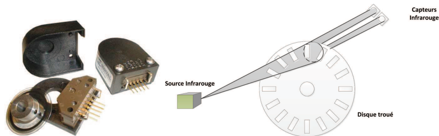
FIGURE 2.4: Fonctionnement d'un odomètre
