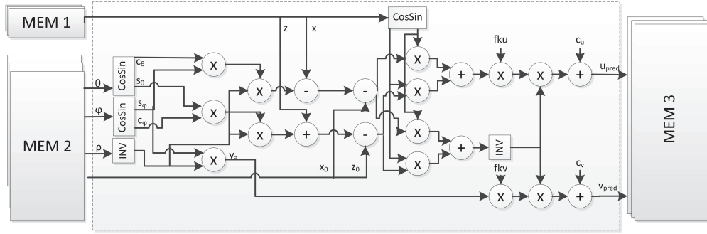
FIGURE 4.17: Architecture du bloc fonctionnel "Projection d'un amer"
