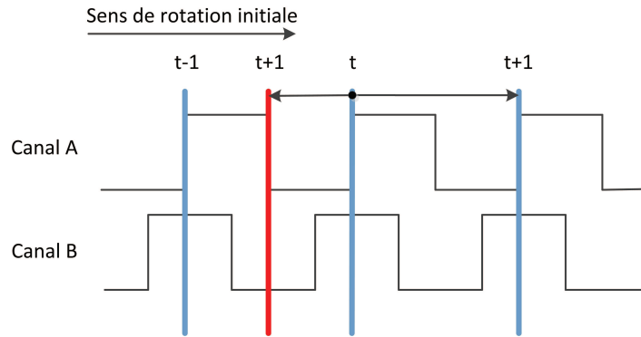
FIGURE 2.5: Signaux émis par un odomètre.
