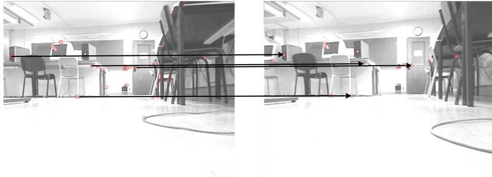
Figure 2.10: Résultats de la mise en correspondance des points d'intérêts
