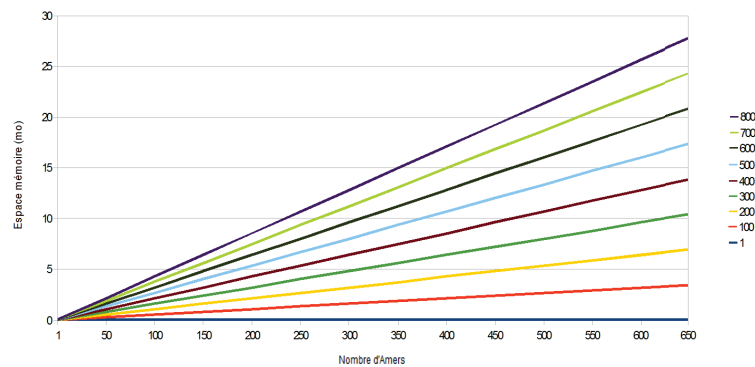
FIGURE 4.9: Espace mémoire nécessaire en fonction du nombre d'amers et du nombre de particules
