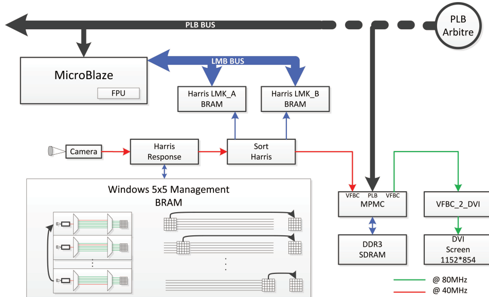
FIGURE 1.8: Architecture dédiée au SLAM par Botero et al. [8]
