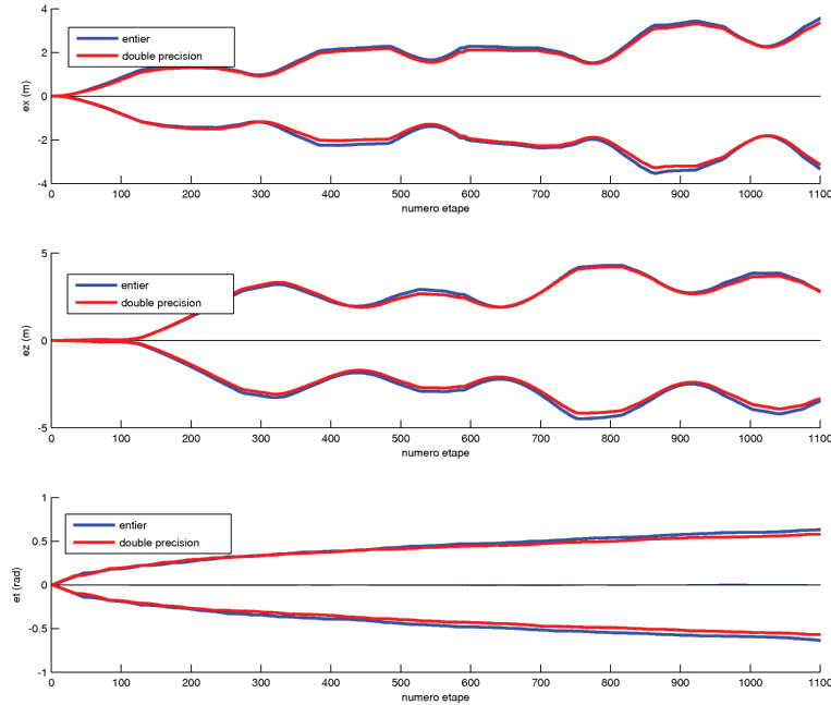
FIGURE 4.23: Couloir d'incertitudes issus de la phases de prédiction - Comparaison avec l'implantation en double précision
