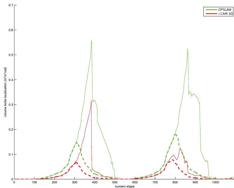
Figure 5.27: Volume de la boîte de localisation en utilisant un caméra 3D
