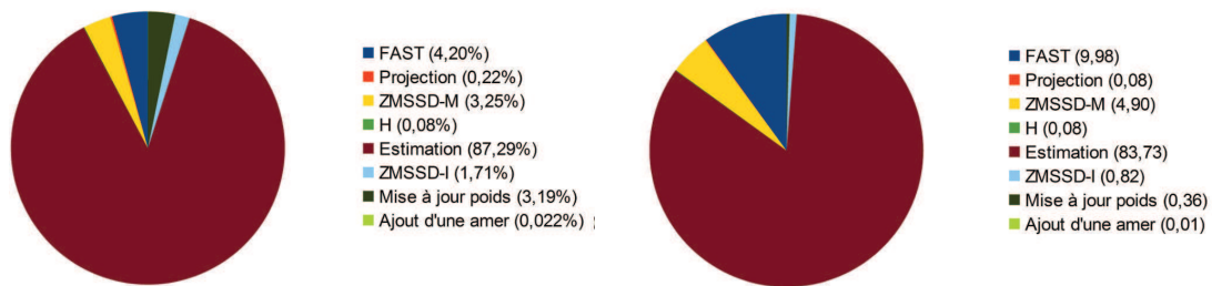
(a) Répartition des temps d'exécution pour le Cortex A8 (b) Répartition des temps d'exécution pour le Cortex A9
