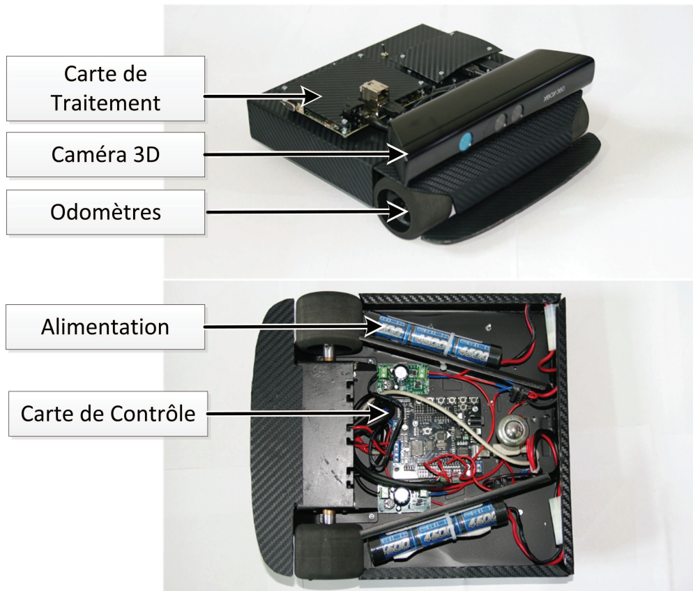
FIGURE 2.1: MiniB : Plateforme instrumentée
