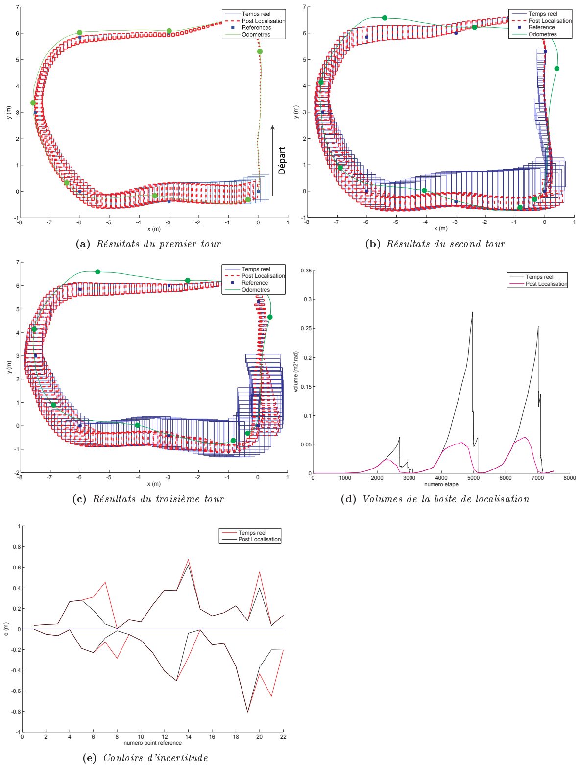
FIGURE 5.25: Résultats expérimentaux du CPSLAM
