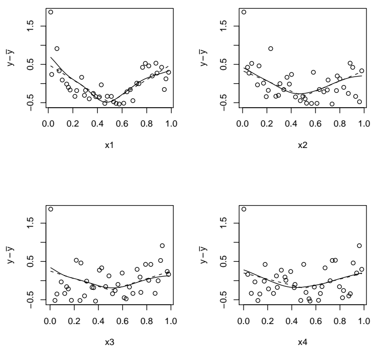
FIGURE 3.6 – Projection des observations sur chacun des axes (cercles) pour la fonction de Sobol en dimension 4. Les modèles univariés obtenus après 5 itérations RLM sont représentés en trait plein et les effets principaux analytiques sont en pointillé.
