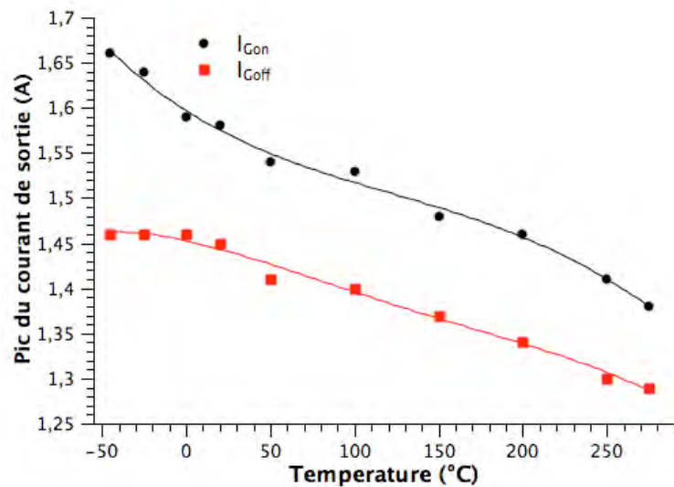
FIGURE 4.22 – Evolution du courant de sortie du driver Drv1
