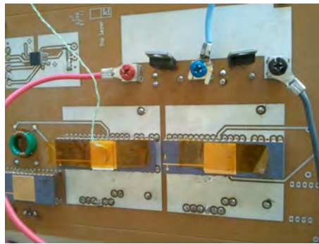
(b) Carte de test
