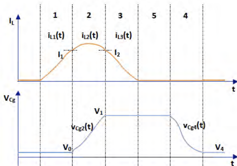
Figure A1.3 : Illustration d'un fonctionnement possible du driver schématisé de la figure A1.2
