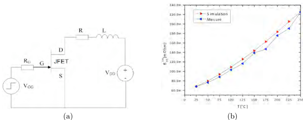
FIGURE 1.34 – Cellule de validation du modèle du JFET (a) et caractéristique statique R_{DS(on)} en fonction de la température (b) [HAM 11]
