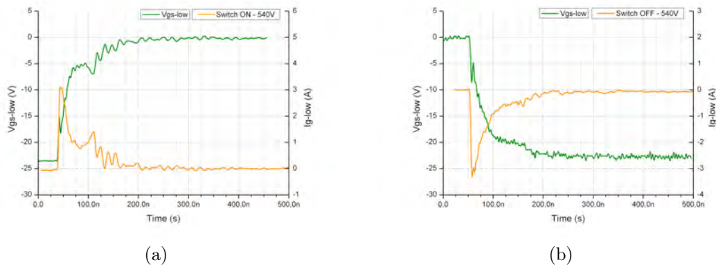
FIGURE 1.30 – Caractéristiques de grille du JFET bas de pont à la fermeture (a) et à l’ouverture (b) [ROB 11]
