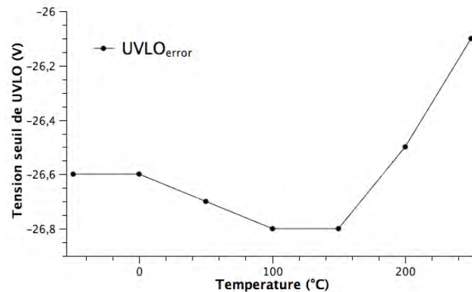
FIGURE 4.11 – Simulation de la tension de seuil UVLO avec la température ambiante
