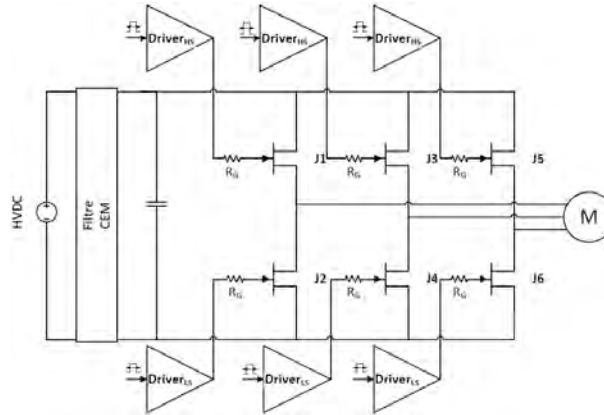
FIGURE 1.41 – Positionnement des drivers au sein de l'onduleur de tension
