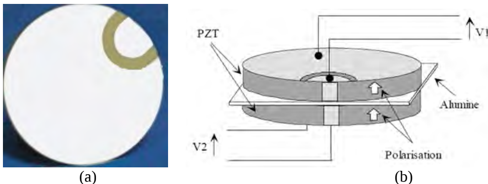
Figure A2.2 : (a) Échantillon de résonateur en céramique PZT, (b) Structure du transformateur multi-couche
