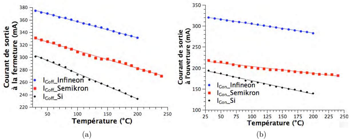
FIGURE 2.30 – Courant de sortie : (a) à la fermeture, (b) à l'ouverture
