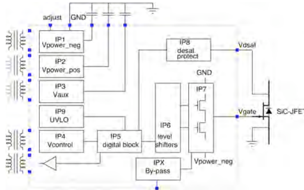
FIGURE 1.42 – Synoptique originel de la contribution du projet FNRAE COTECH au driver intégré SOI
