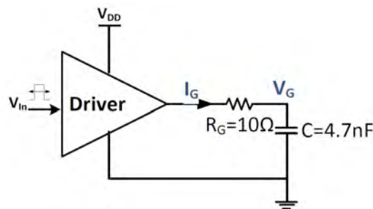
FIGURE 2.25 – Dispositif de test pour les drivers commerciaux
