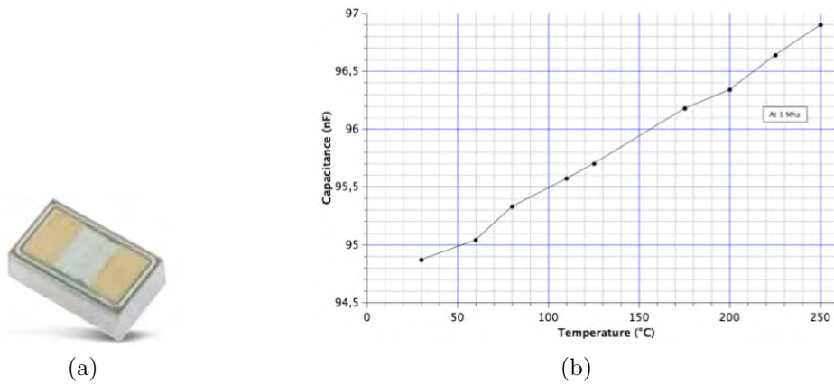
FIGURE 1.9 – Vue de la capacité HTSC424-100 (a). Evolution de la valeur de la capacité d’un produit HTSC424-100 (b) ( source Ipdia )
