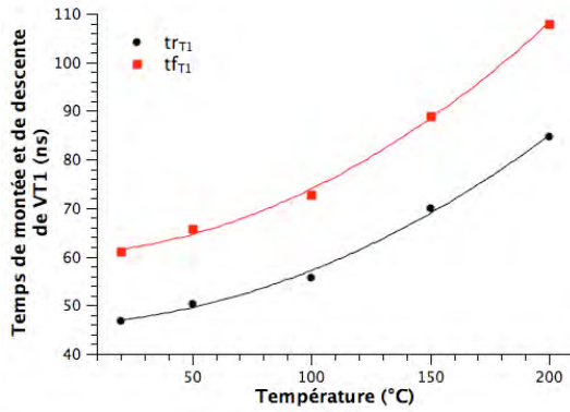
(a) JFET T1
