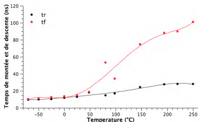
FIGURE 4.29 – Mesure des temps de montée et de descente du driver Drv3
