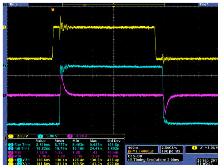
FIGURE 4.20 – Relevé des courbes à 275^{\circ}C
