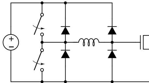
Figure A1.10 : Circuit semi-résonant à une phase de récupération d'énergie dans l'inductance
