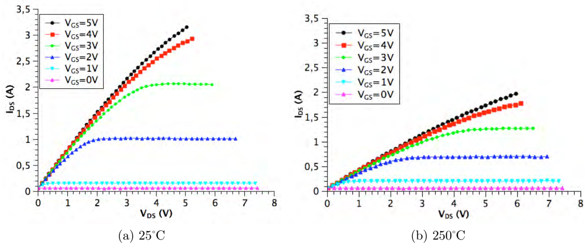
FIGURE 3.6 – Caractéristique statique du transistor NMOS 45V à température ambiante et à 250^{\circ}\text{C}
