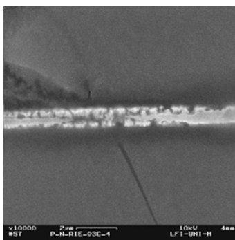
FIGURE 1.19 – Exemple de rupture de ligne due à l'électromigration ( source electromaniacs.com )
