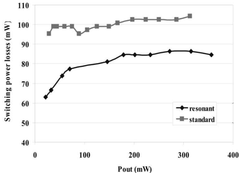
Figure A1.14 : Impact du driver résonant sur les pertes de commutation
