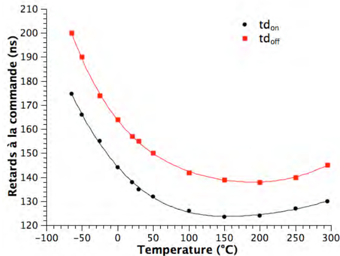
FIGURE 4.25 – Retards à la commande en fonction de la température
