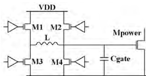
Figure A1.13 : Driver résonant en CMOS SOI 0.13μm [BAT 12]
