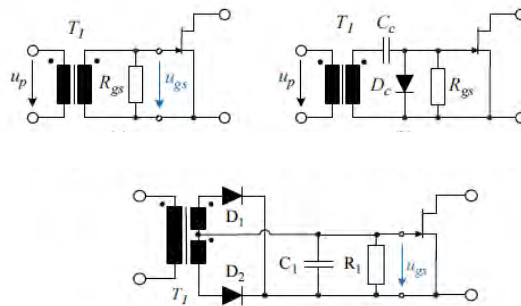
FIGURE 2.4 – Architecture de drivers sans étage de sortie [WAF 08]
