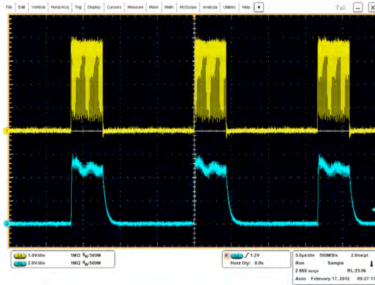
FIGURE 3.28 – Forme d'onde d'entrée et de sortie de la fonction d'isolation
