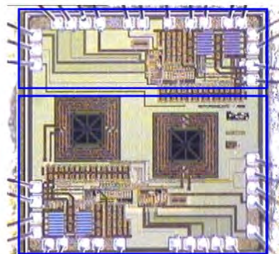
Figure A1.13 : Driver résonant en CMOS SOI 0.13μm [BAT 12]
