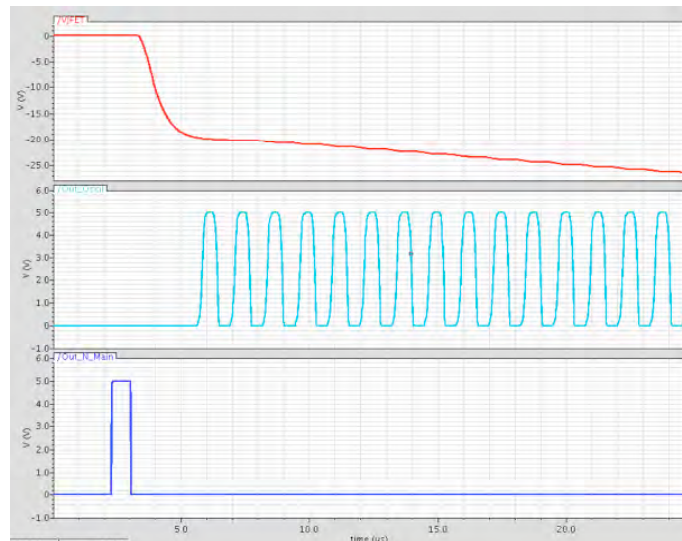
FIGURE 4.16 – Simulation des tensions caractéristiques de la fonction à 200°C
