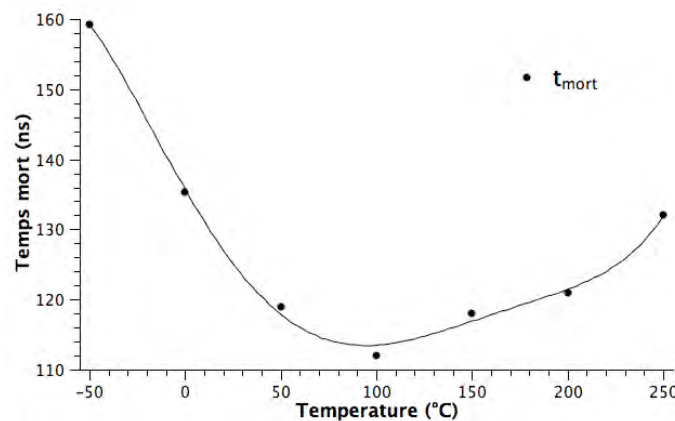
FIGURE 4.3 – Simulation de t_{mort} avec la température
