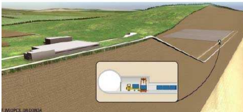
Figure 14 : L'option du « stockage sous couverture intacte » (SCI) [ANDRA, 2008]
