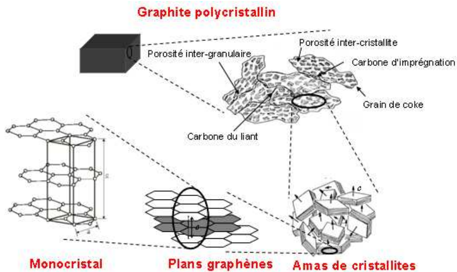
Figure 6 : Schéma multi-échelles de l'organisation structurale du graphite polycristallin [BONAL, 2007]
