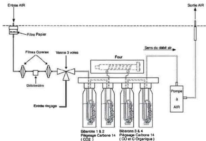
Figure 28 : Le barboteur HAG 7000 [SDEC]
