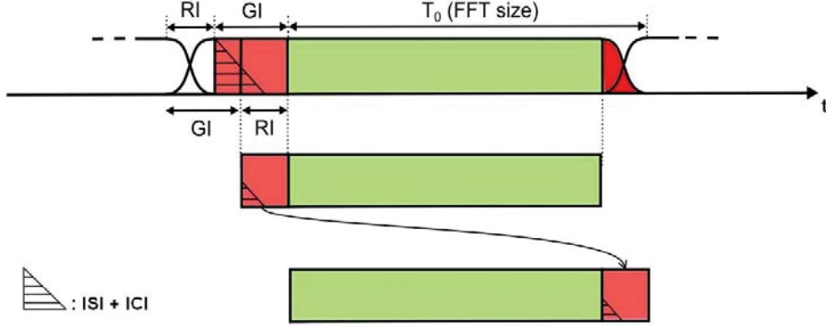
Figure D.2: Pré-traitement effectué au niveau de récepteur avant de démoduler le signal windowed OFDM.
