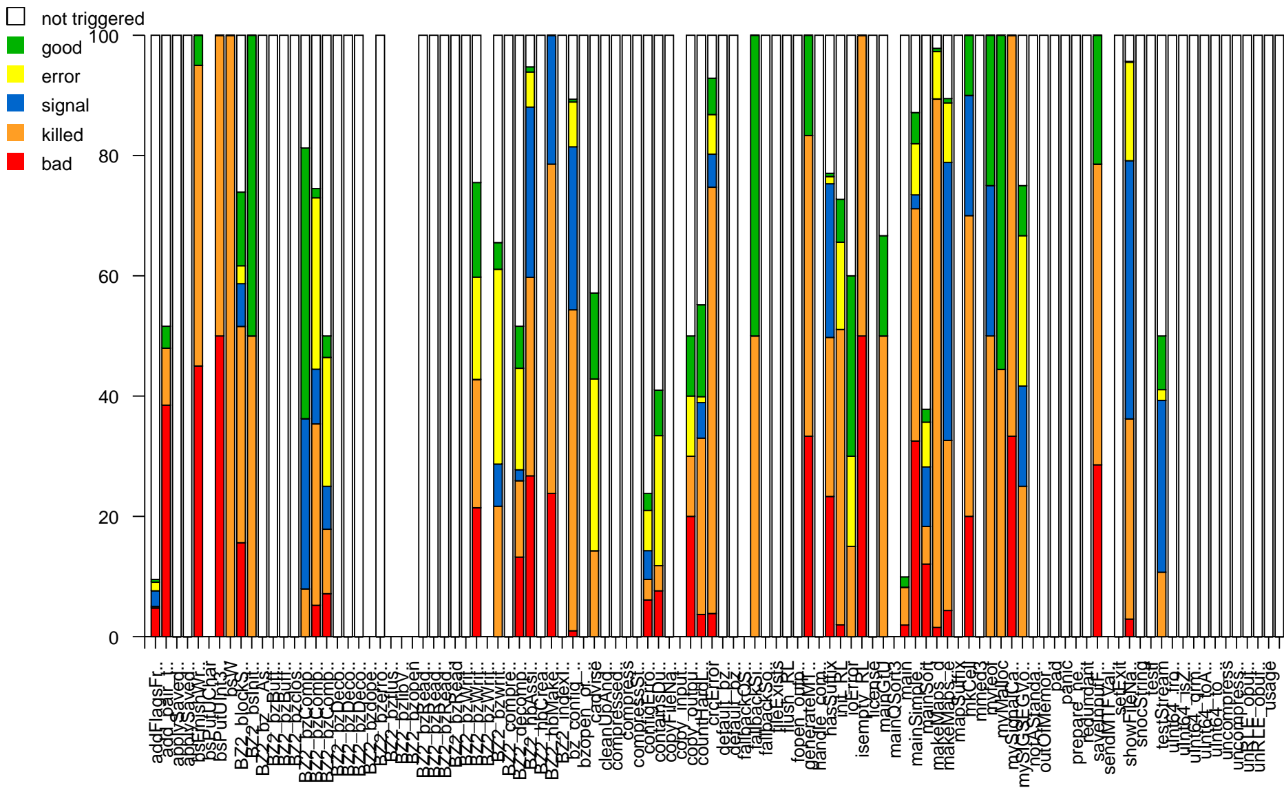
FIGURE 5.5 – Résultats d’attaques permanentes réalisées en C sur le code de BZIP2
