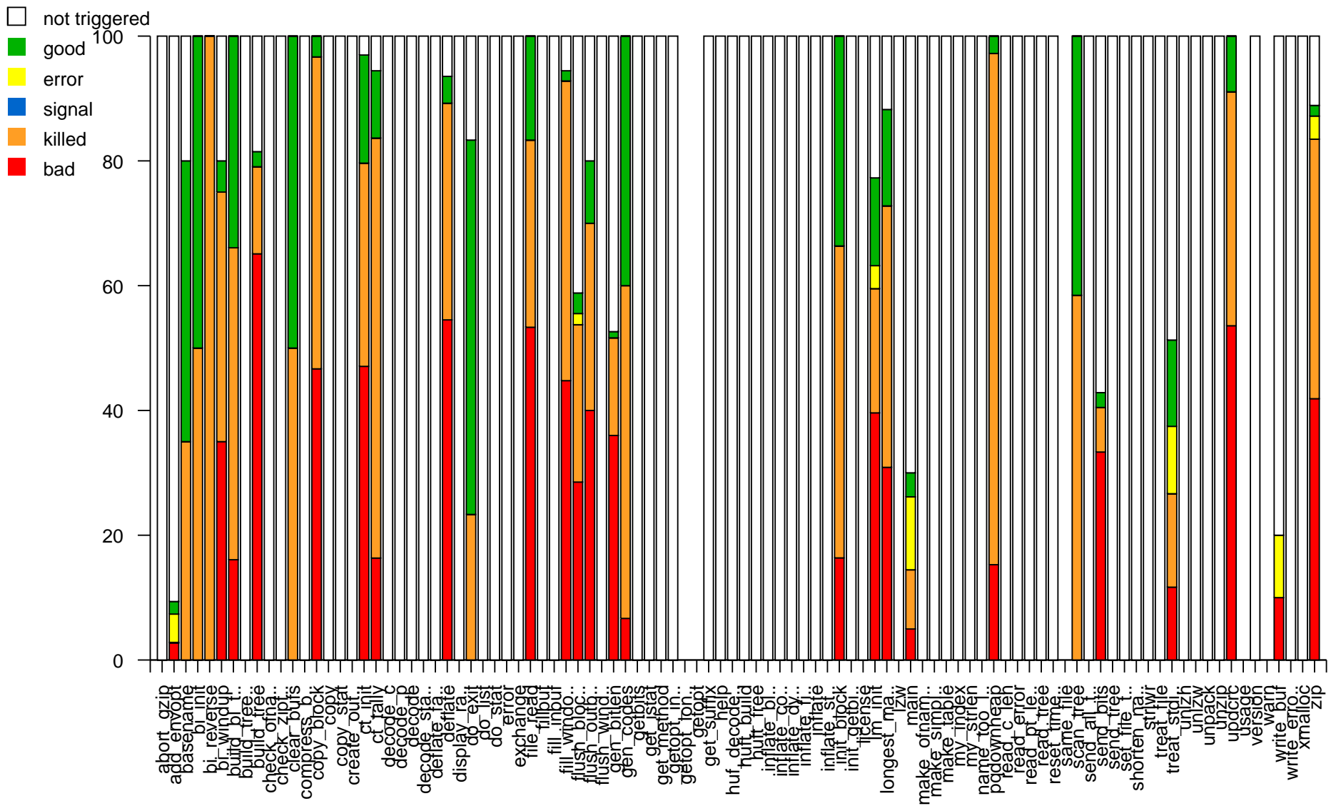
FIGURE 5.6 – Résultats d'attaques permanentes réalisées en C sur le code de GZIP
