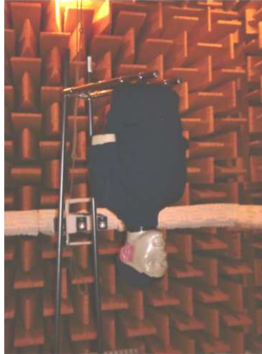
FIGURE 4.12 – Photo de l’installation du mannequin KEMAR à l’envers dans la chambre anéchoïque de l’IRCAM pour réaliser la mesure des HRTF comprises entre 0 et -90^\circ d’élévation.
