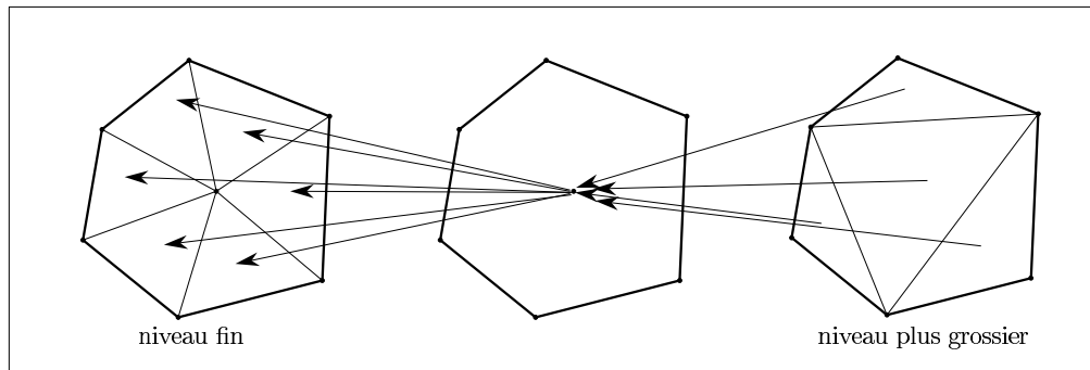
Figure 1.29 – un niveau intermédiaire pour construire une triangulation de Delaunay hiérarchique.
