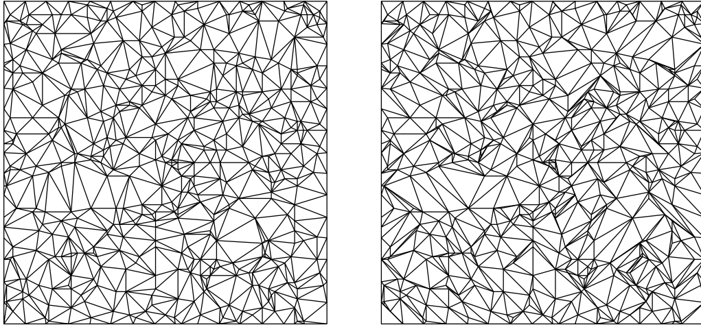
Figure 5.16 – bon exemple à 500 points : la triangulation obtenue par la méthode 13 (à droite) renvoie une erreur 28% plus petite que celle de Delaunay.
