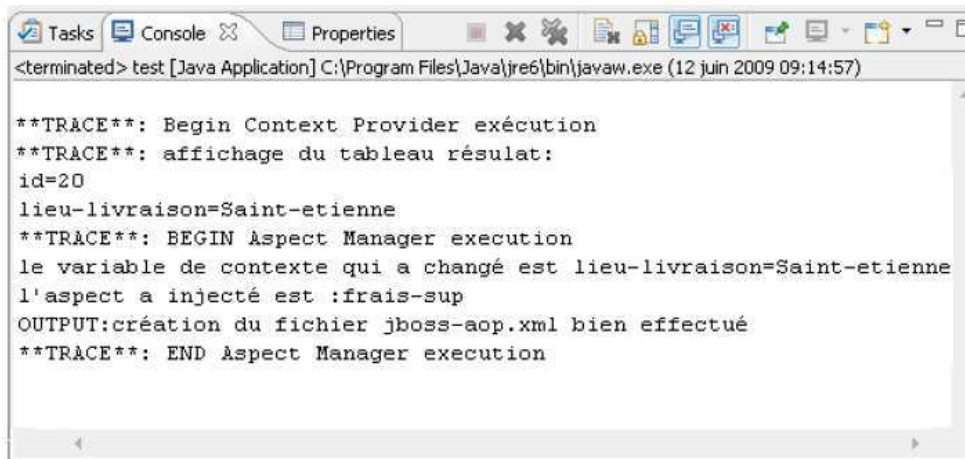
Figure C.7. Résultat d'exécution de la classe Test
