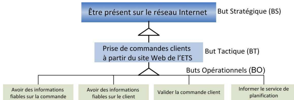
Figure A.6. Arbres de décomposition des buts du processus de prise de commande client
