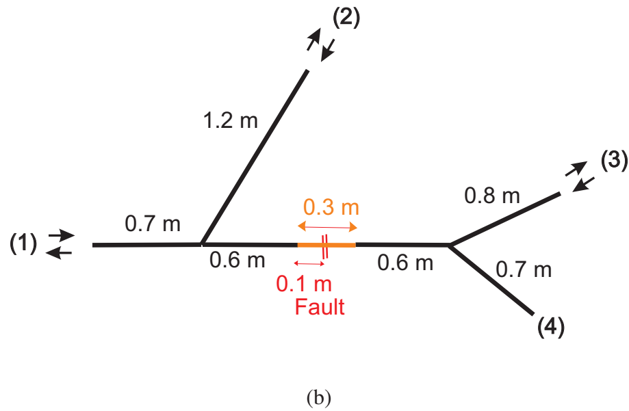
FIGURE I.11 : Réseau implémenté pour tester la méthode de localisation.
