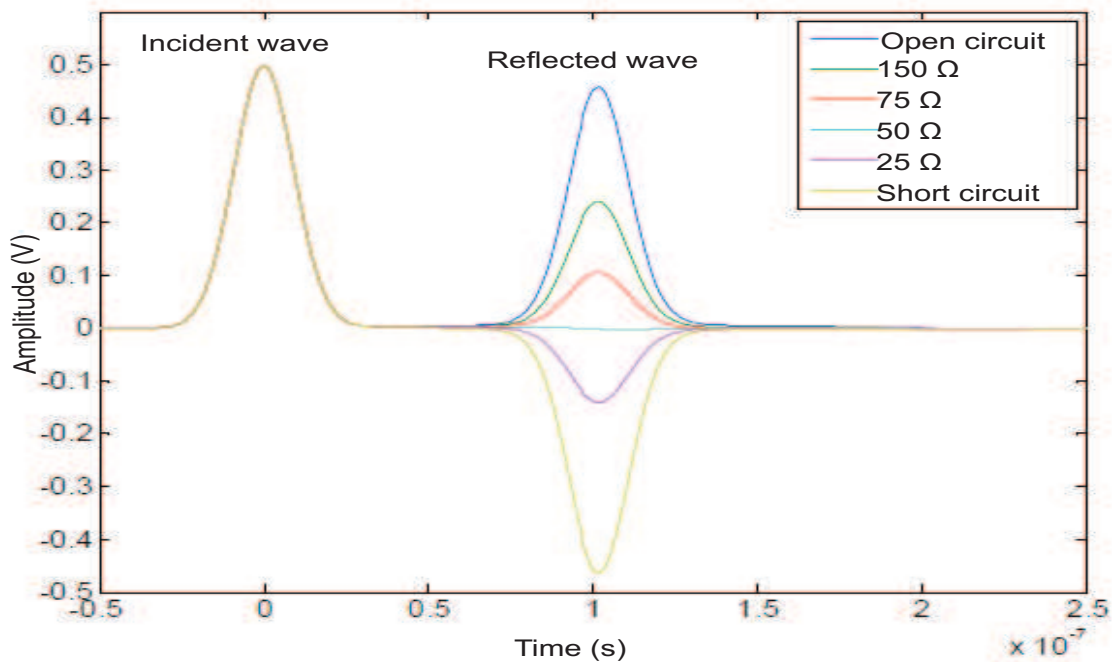
FIGURE I.4 : Exemple de la TDR standard appliquée à un câble coaxial 50 Ω, pour différentes valeurs de la charge à l'extrémité. Source : N. Ravot, Analyse et Diagnostic de Réseaux Filaires Complexes par Réflectométrie . Thèse de l'Université Paris-Sud 11, 2007.
