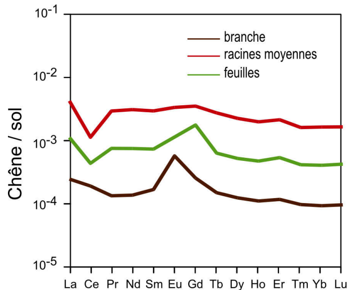
Figure 2.53 : Spectre des TR du chêne du site sur carbonatites ; normalisation par rapport au sol ; n=1 pour tous les échantillons.
