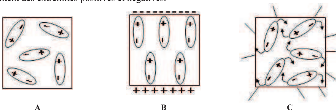
Figure II.16. Comportement de molécules dipolaires [69] A. agitation thermique; B. action de champ électrique; C. action de microondes
