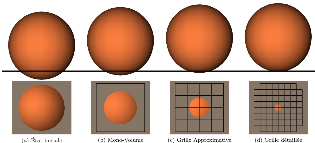
FIG. 4.20 – Intersection après la résolution des contraintes, pour différentes résolutions de la grille. Les figures du bas présentent un vue de dessus alors que les figures du haut présentent une vue de profil. En augmentant le nombre de multi-volumes, on obtient une solution plus précise.
