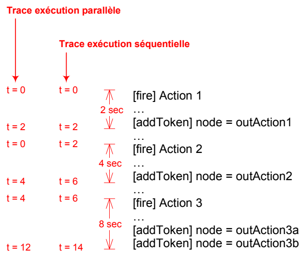
FIGURE 4.11 – Trace d’exécution contenant des informations temporelles
