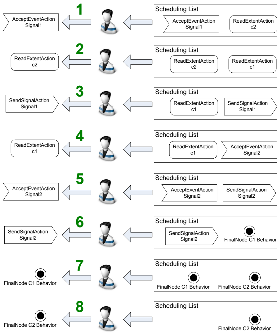
FIGURE 4.10 – L’ordre des actions sélectionnées par l’utilisateur
