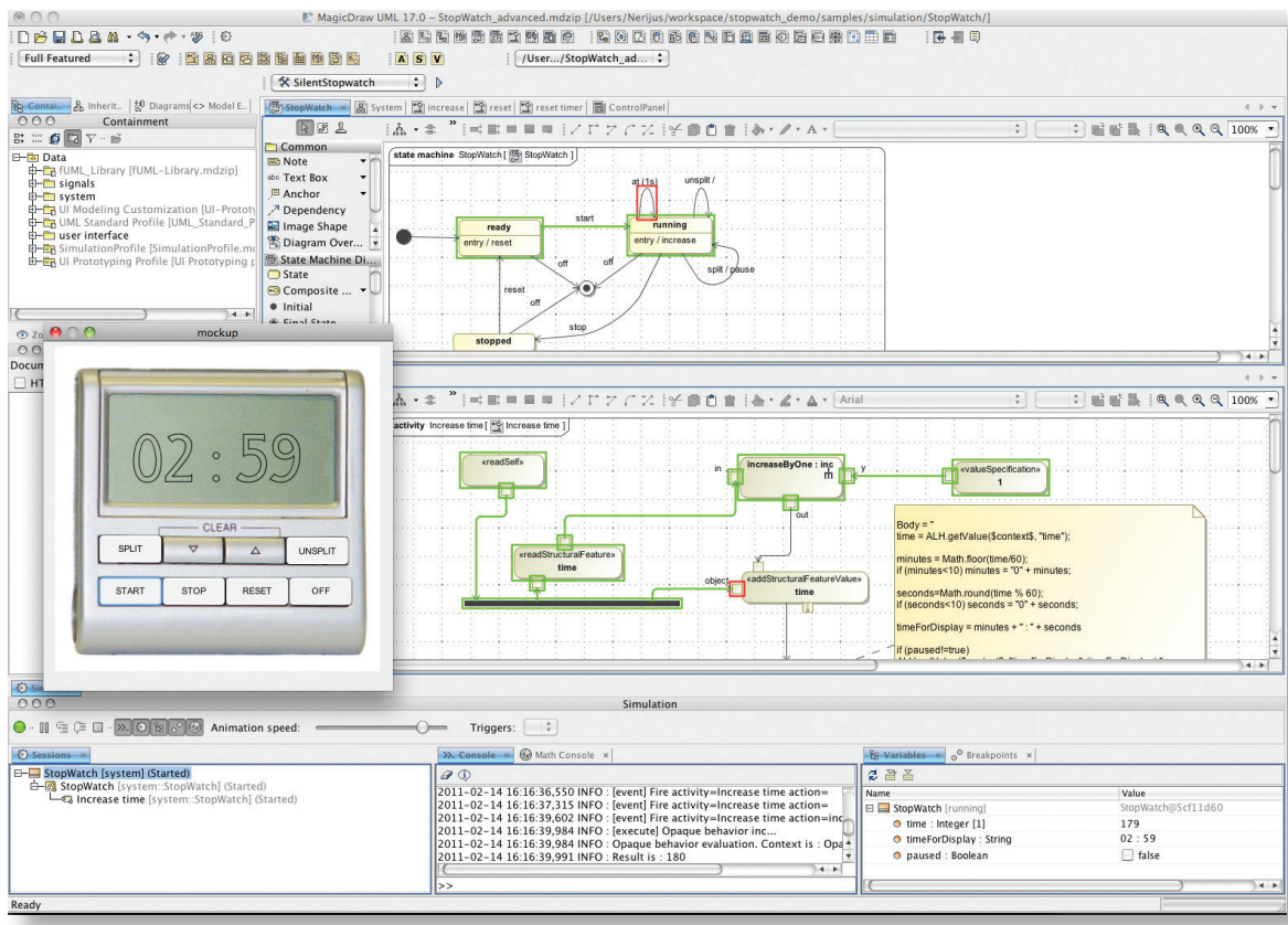
FIGURE 3.10 – Capture d'écran de l'environnement MagicDraw/Cameo
