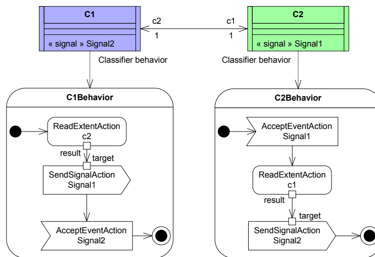
FIGURE 4.5 – Modèle fUML d'un système asynchrone simple
