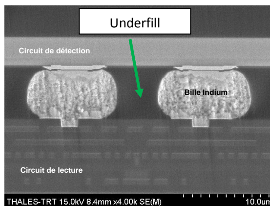
Figure 82 : Cliché MEB d'une micro-section d'un hybride Intense avec billes d'Indium au pas de 15µm.
