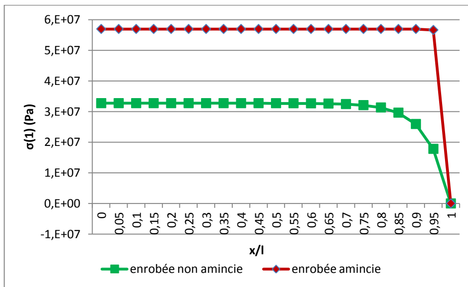
Figure 28 : Effet de l'amincissement sur la répartition des contraintes de traction dans le détecteur (GaAs) d'épaisseurs 650 \mu m et 400 \mu m avec \Delta T=223K et une taille de structure de 5mm de longueur.
