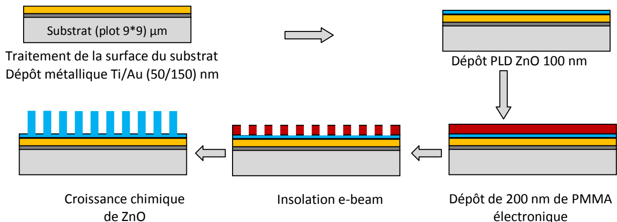
Figure 144 : Etapes technologiques nécessaires pour le dépôt des nano-fils ZnO Sur une surface d'un seul plot (UBM) de dimension (9*9) μm. Les plots sont disposés sur la surface du substrat avec une période de 15μm.
