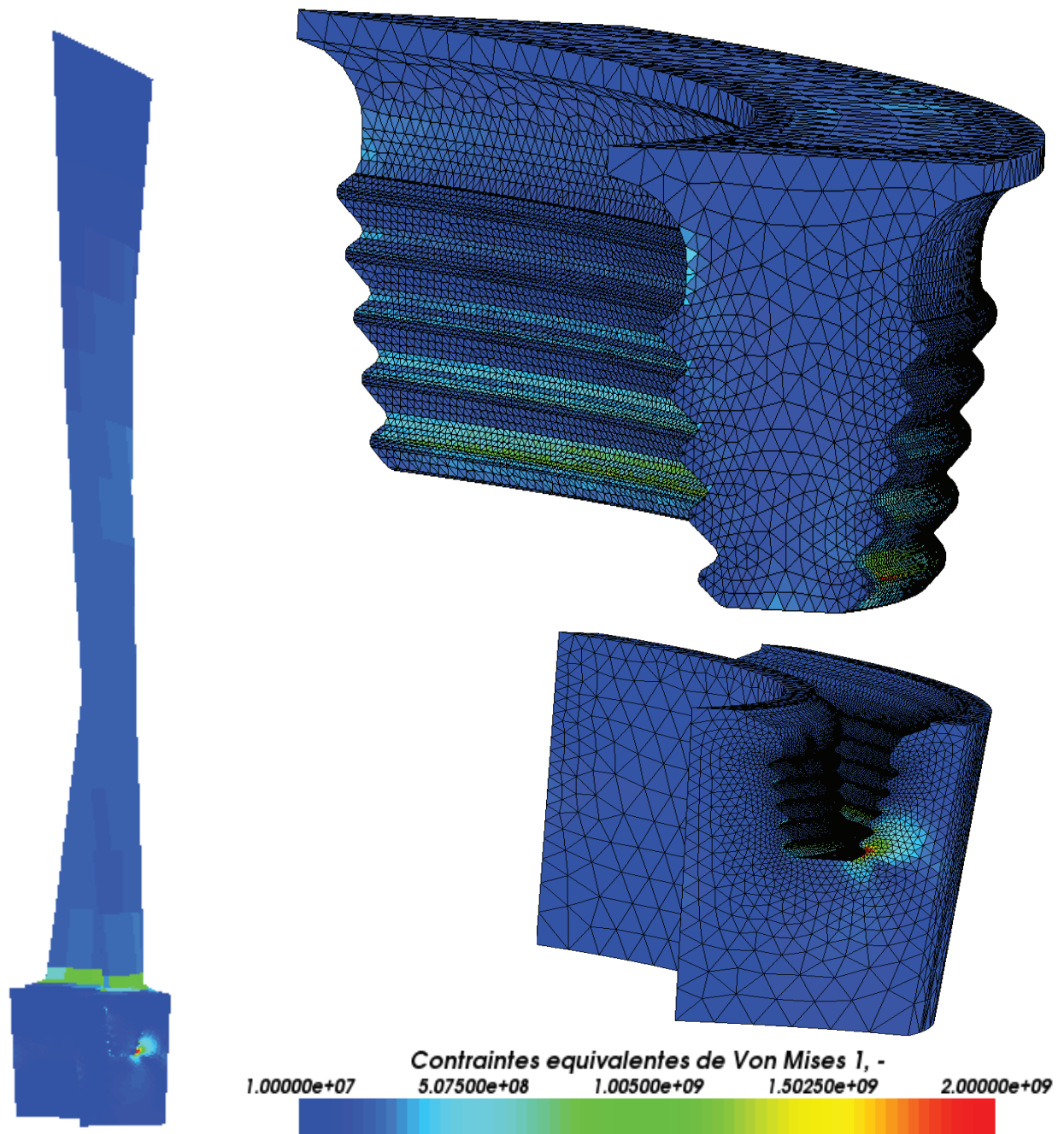
FIGURE 5.29 – Problème de contact-frottement sur les pieds d’ailettes : contraintes de Von Misès
