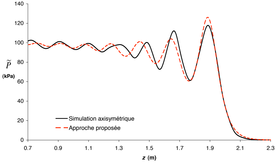
FIG. 3.18: Evolution spatiale de la pression macroscopique dans un liquide avec des clusters de bulles. Gaz : N_2 , liquide : huile silicone. Rayon de bulles a_0 = 4\text{mm} , rayon de cluster R_{10} = 3.48\text{cm} , fraction volumique d'air dans les clusters f_{c0} = 4\% , fraction moyenne de vide dans le mélange f_0 = 1.02\% , fraction volumique de clusters \alpha_0 = 25.4\% , P_0 = 109.3\text{kPa} , \Delta P = 101.2\text{kPa} , q = 6/\pi , q_1 = 3/2 , temps d'observation t = 15\text{ms} . 26 bulles dans chaque cluster. Coefficient de séparation d'échelles : \epsilon \sim 2.2 .
