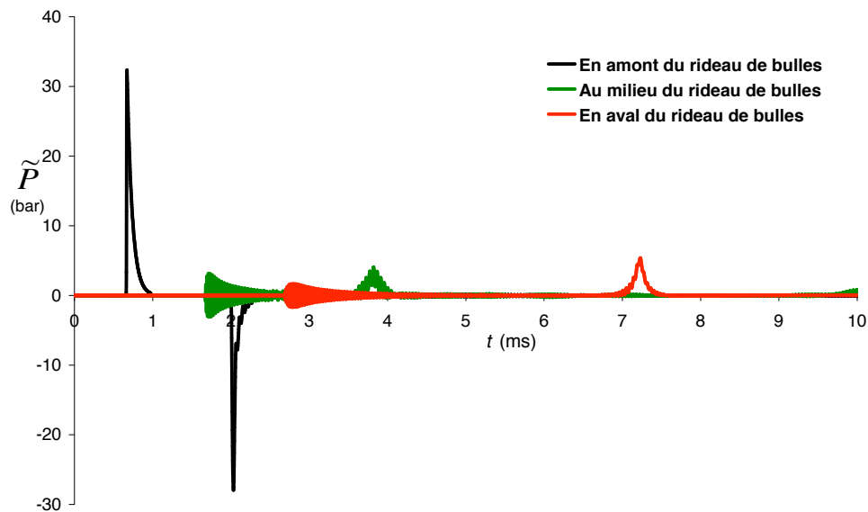
FIG. 5.4: Profils temporels de pression en amont, au milieu et en aval d'un rideau de bulles. Porosité uniforme au sein du rideau. f_0 = 1\% - a_0 = 2\text{mm} - P_m = 35\text{ bars} - \theta = 0,15\text{ ms} . Le liquide en amont est régi par l'équation d'état 2.39. Domaine de calcul : L_1 = L_2 = 2\text{ m} , L_R = 1\text{ m} .
