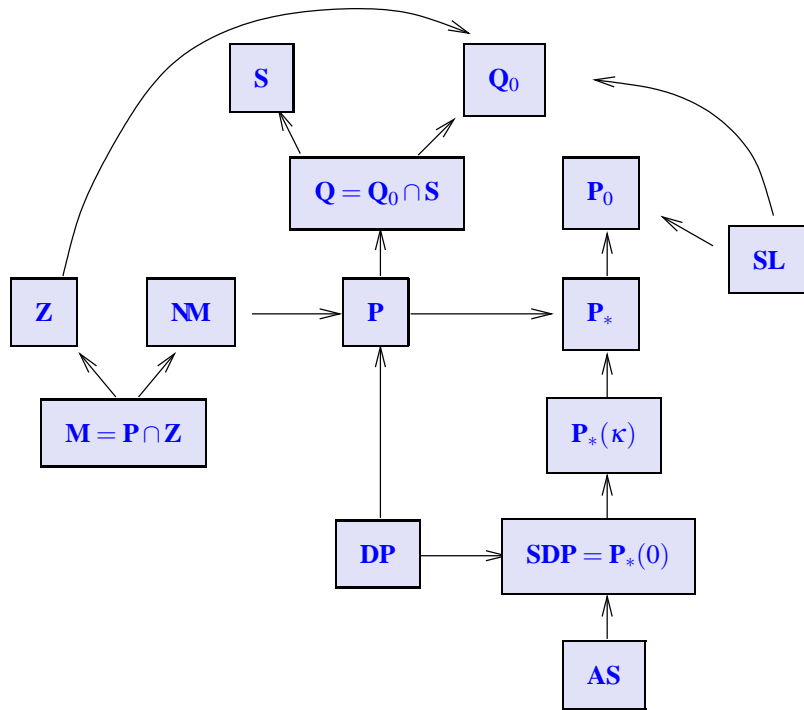
Figure 2.2.1 – Propriétés d’inclusion de quelques classes de matrices : la flèche A \rightarrow B indique que A \subset B (on peut cliquer sur la figure pour voir les propriétés de chaque classe de matrices)
