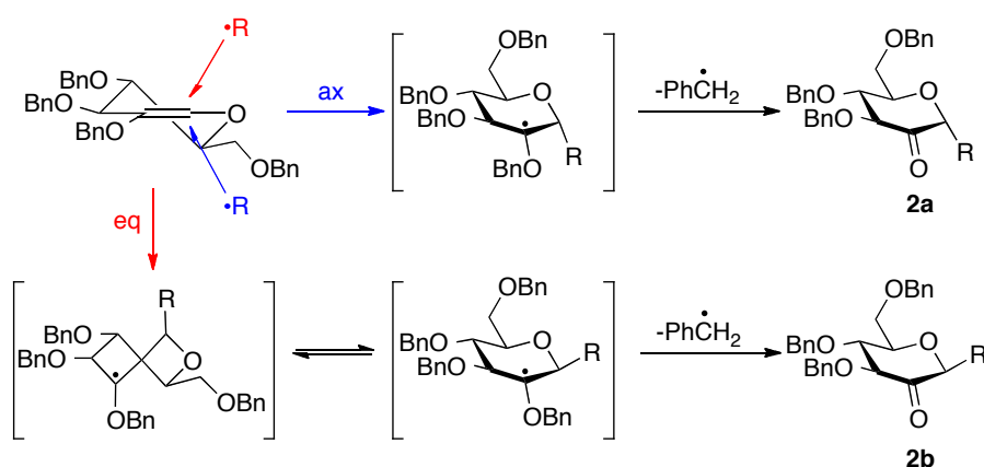
Schéma 36 : Diastéréosélectivité de l'addition radicalaire du 2-benzyloxy-D-glucal
