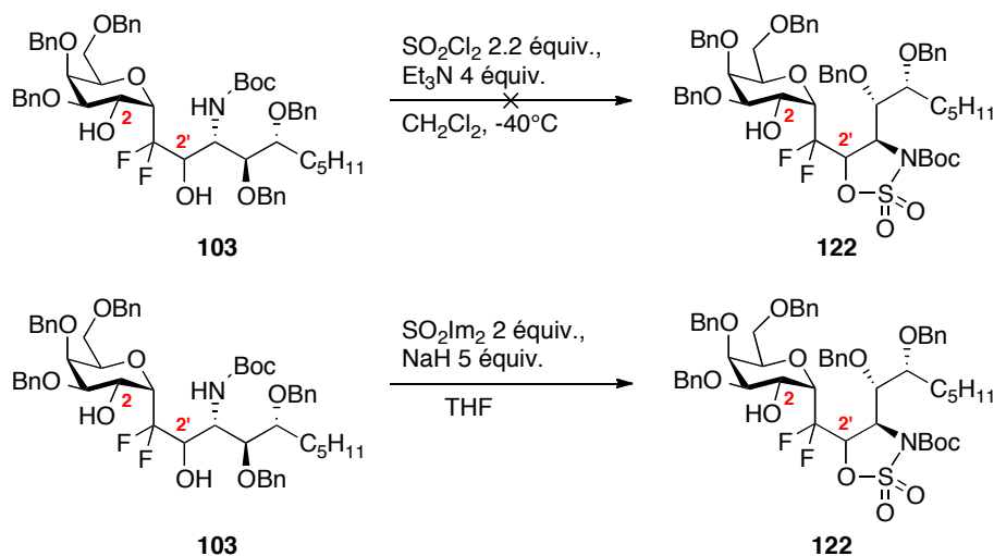
Sch\u00e9ma 84 : Essais de protection via un sulfamidate en O-2'
