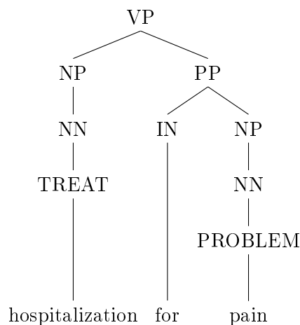
FIG. 4.7 – Exemple du sous-arbre minimal entre les deux entités de type traitement et problème
