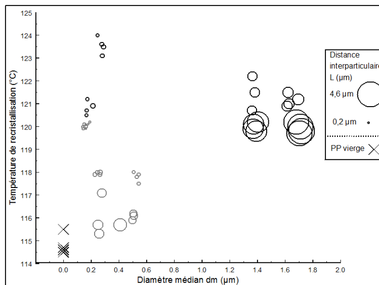
Figure 16 : température de recristallisation des différents mélanges polypropylène et CaCO 3 . La taille de chaque cercle est proportionnelle à la distance interparticulaire, les cercles noirs correspondent aux matériaux sans traitement, les cercles gris aux matériaux traités à l'acide stéarique.
