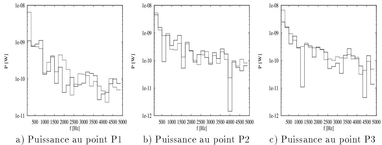
FIG. 5.13 - Puissances actives moyennes échangées (reçues par S_2 ) — calcul exact - - calcul EMMA
