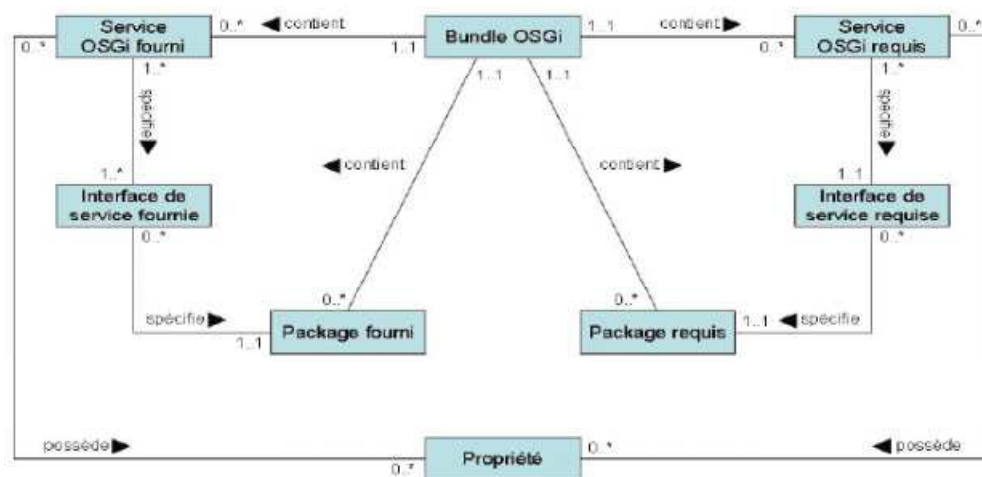
Figure 3.10. Méta-modèle des Bundles OSGi (du point de vue entité logicielle).
