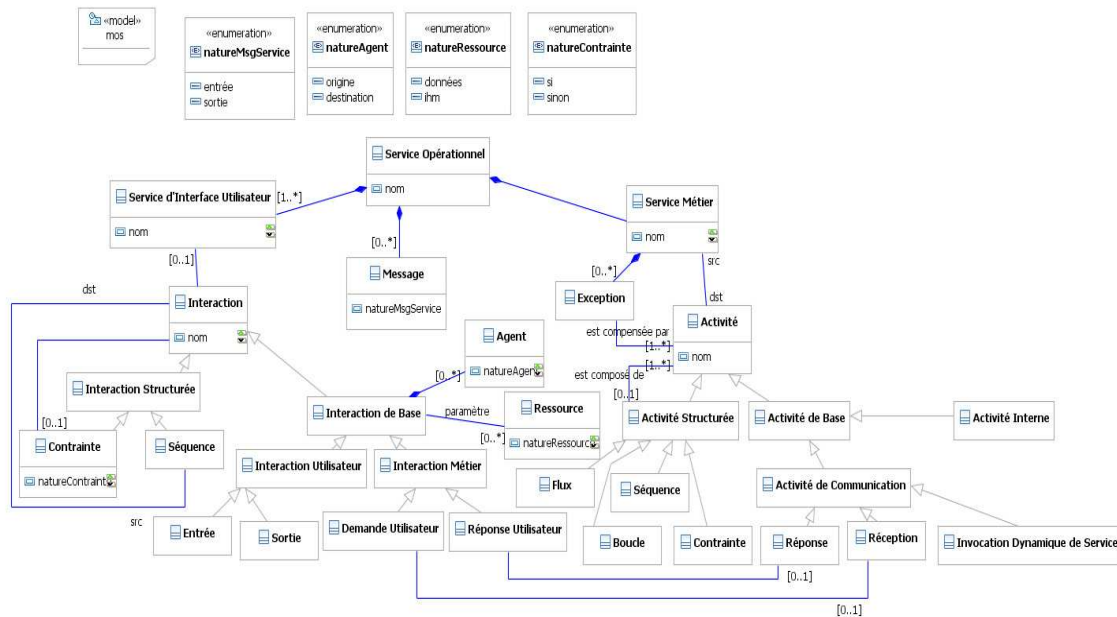
Figure 4.2. Le méta-modèle opérationnel du langage MOS
