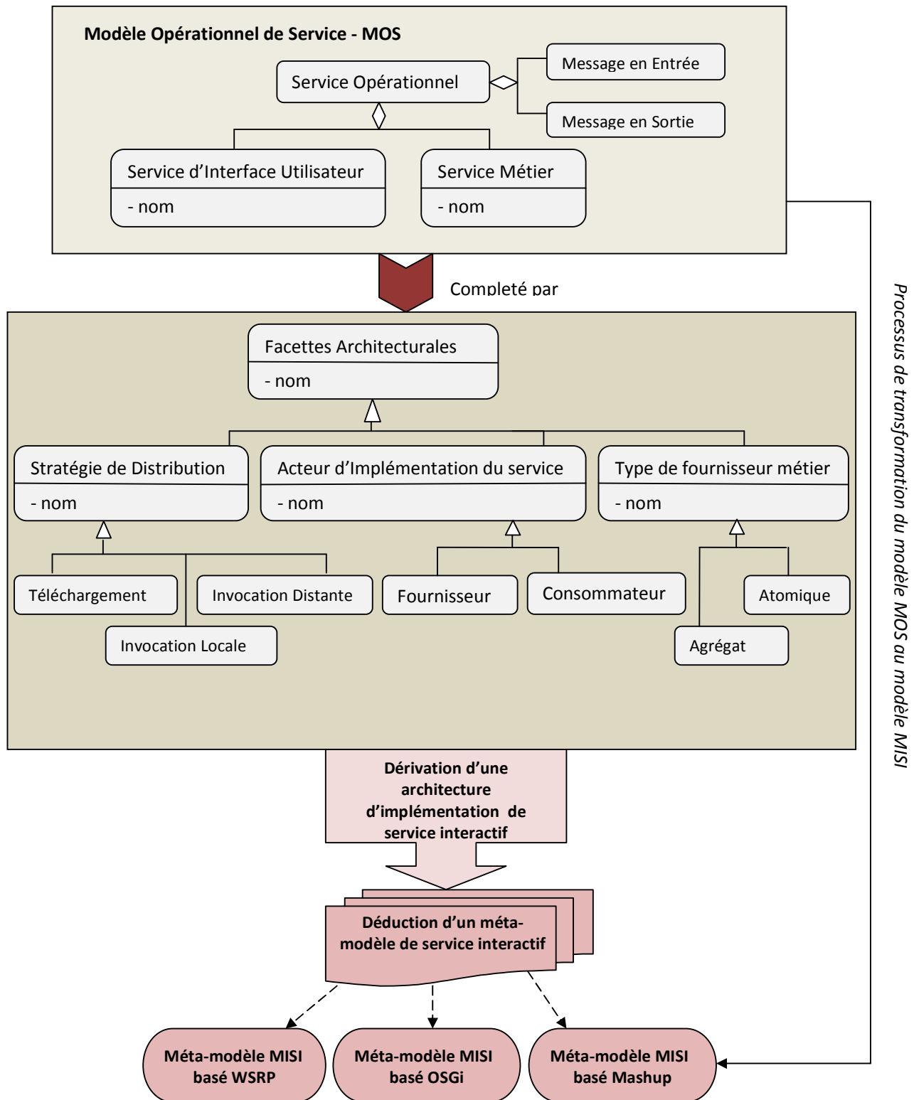
Figure 5.6. : Etape de sélection de l'architecture et plateforme d'implémentation
