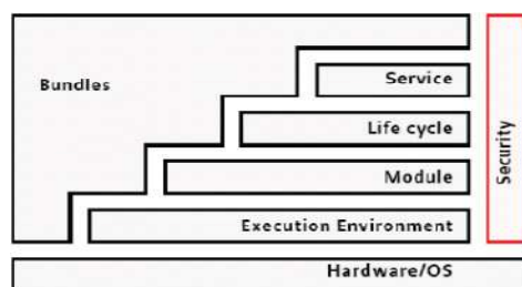
Figure 3.8. Les différentes couches de la plateforme OSGi [OSGi07].
