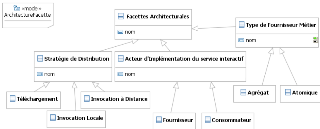
Figure 5.1. : Le méta-modèle de facettes architecturales
