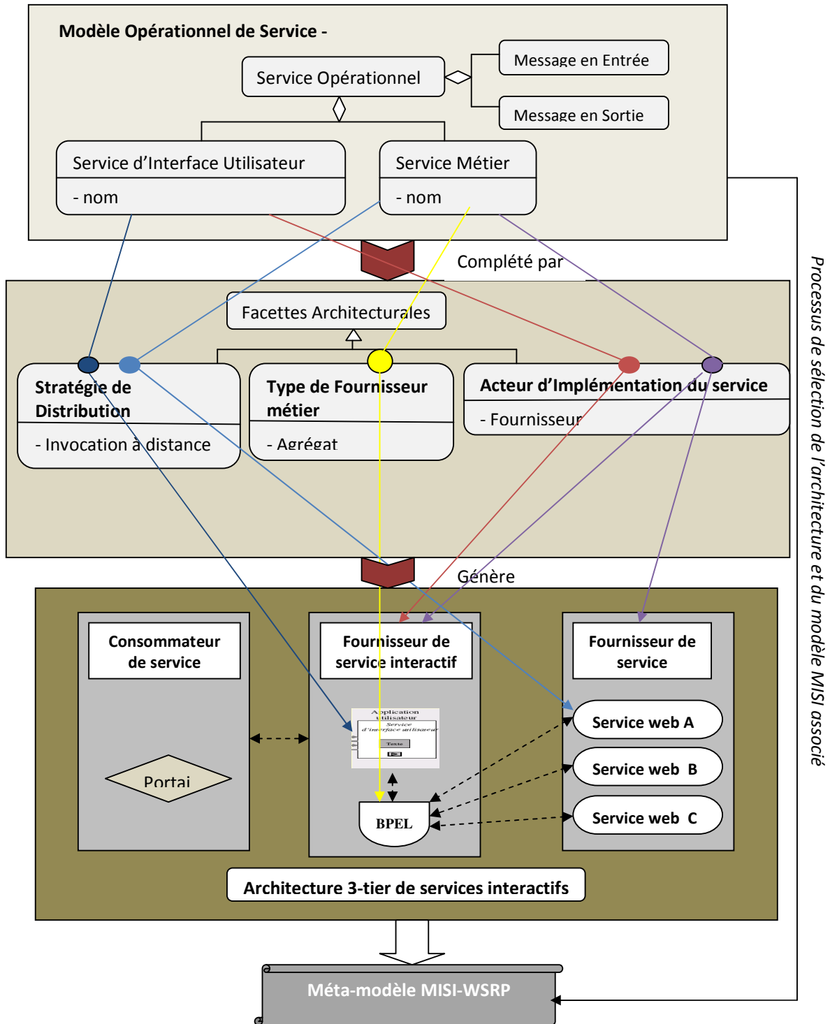
Figure 5.13. : Processus de sélection de l'architecture et du méta-modèle MISI basé
