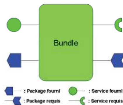
Figure 3.9. Schéma d'un bundle OSGi avec ses packages et services.
