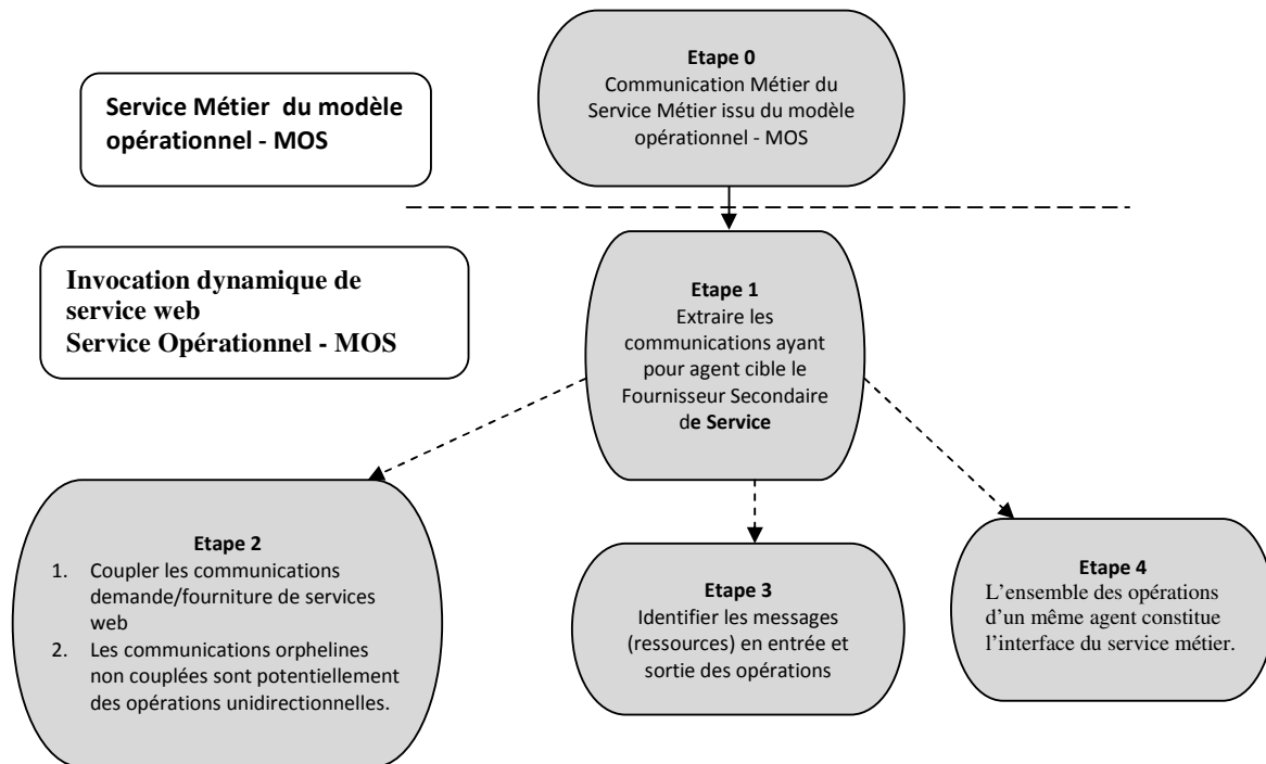
Figure 4.12. Le processus de découverte des opérations et des ressources permettant l'invocation dynamique du service web
