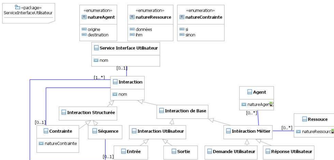
Figure 4.3. Le méta-modèle du Service d'Interface Utilisateur
