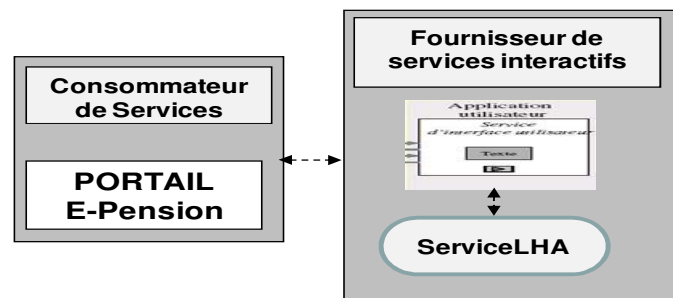
Figure 6.7. Architecture 2-tier de service interactif
