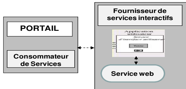
Figure 5.8. : Présentation d'une architecture 2-tier de service interactif
