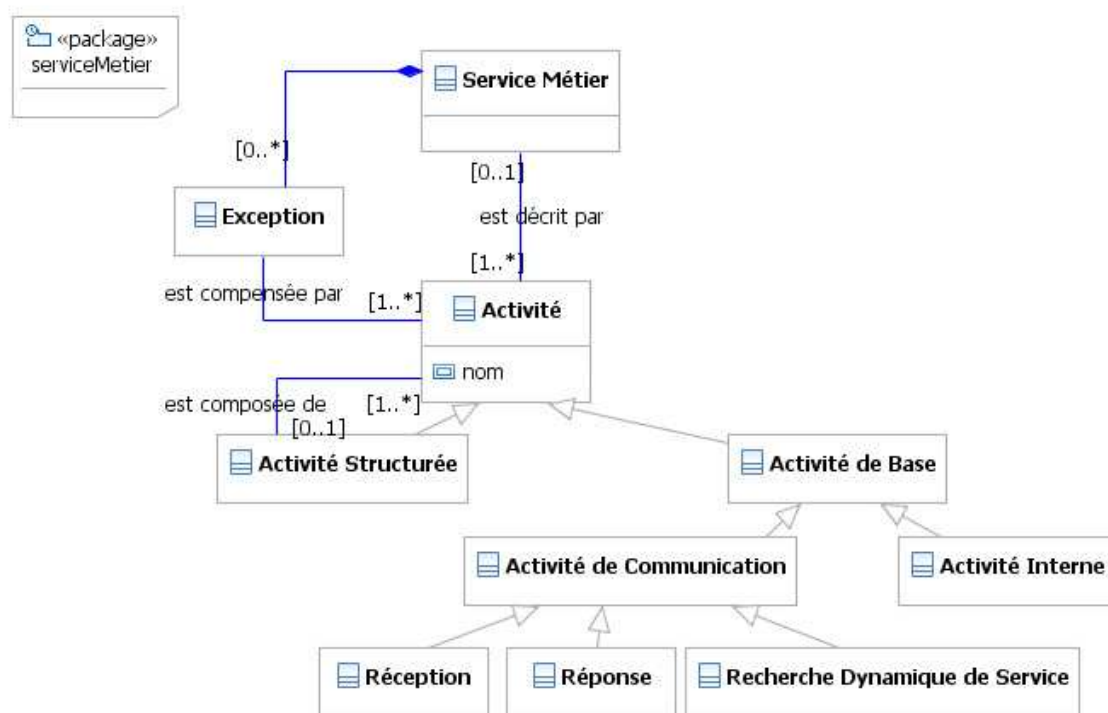
Figure 4.4. Le méta-modèle du Service Métier
