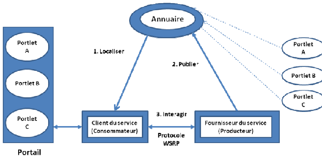
Figure 3.11. Architecture WSRP (paradigme localiser-publier-intégrer).
