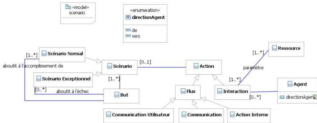
Figure 4.4. Le méta-modèle de Scénario
