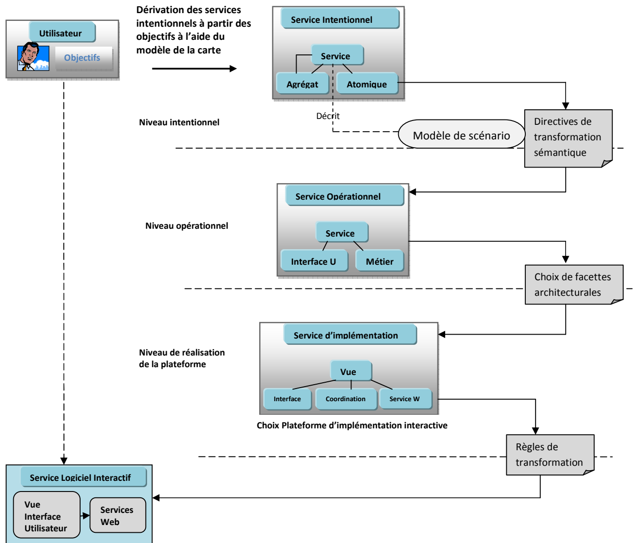
Figure 3.2. La démarche MeTSI
