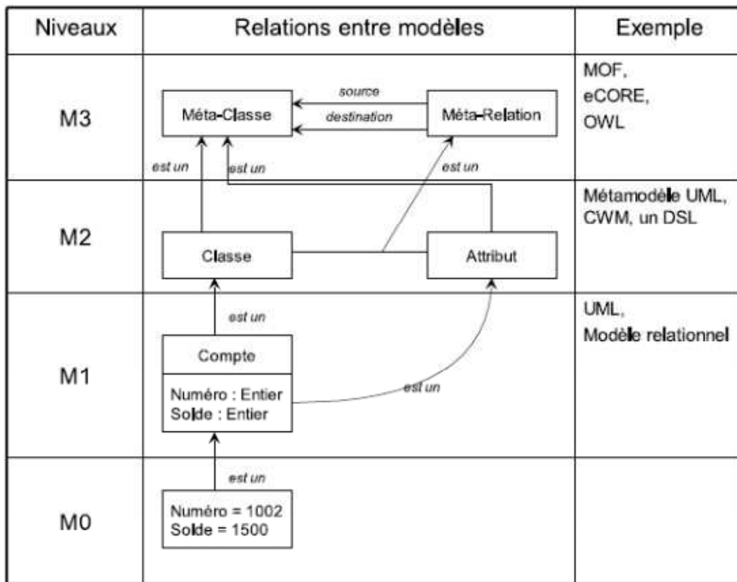
Figure 3.2. Les quatre niveau du MDA
