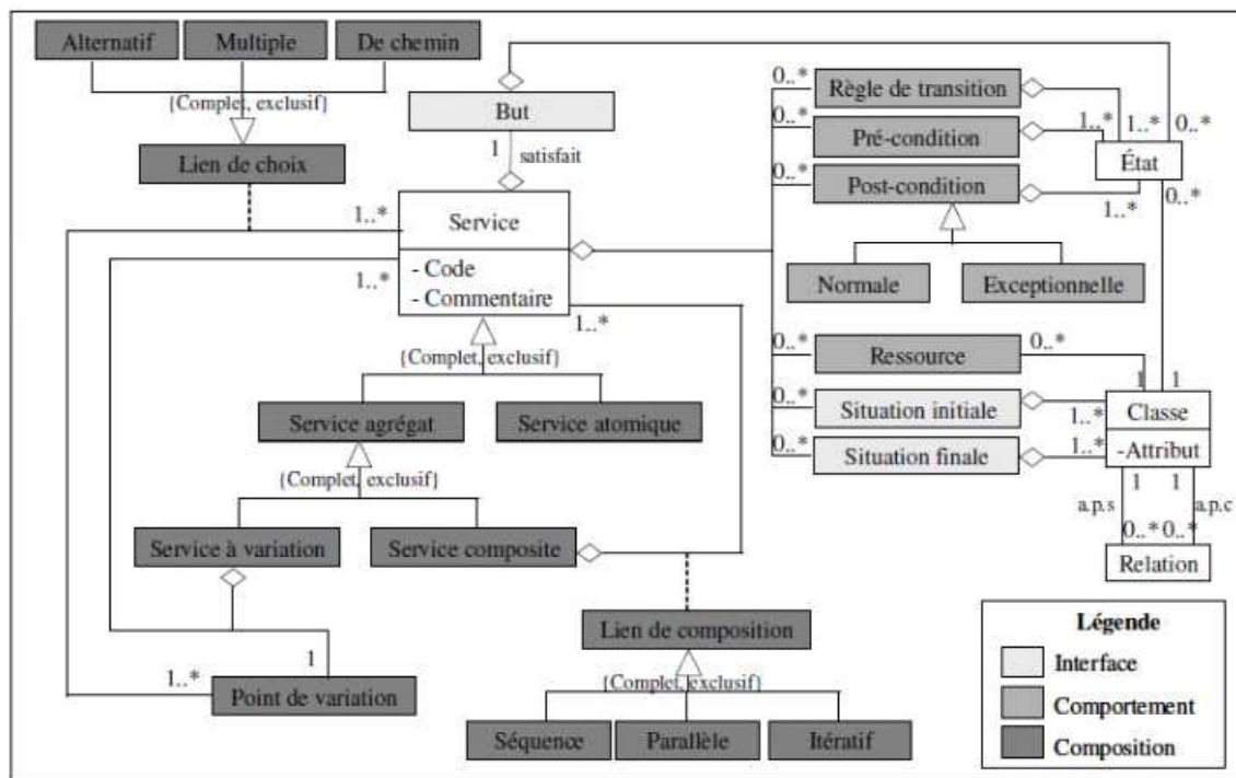
Figure 3.7. Le Modèle Intentionnel de Services (MIS) [Kaabi 2007]
