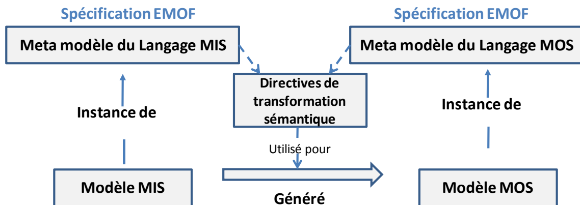
Figure 4.1. Schéma de liaison entre le modèle intentionnel et le modèle opérationnel.
