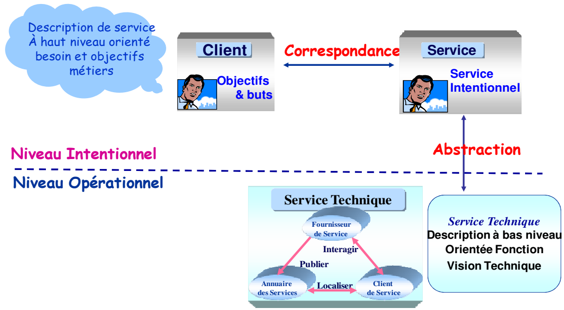
Figure 3.1. Approche orientée services intentionnels
