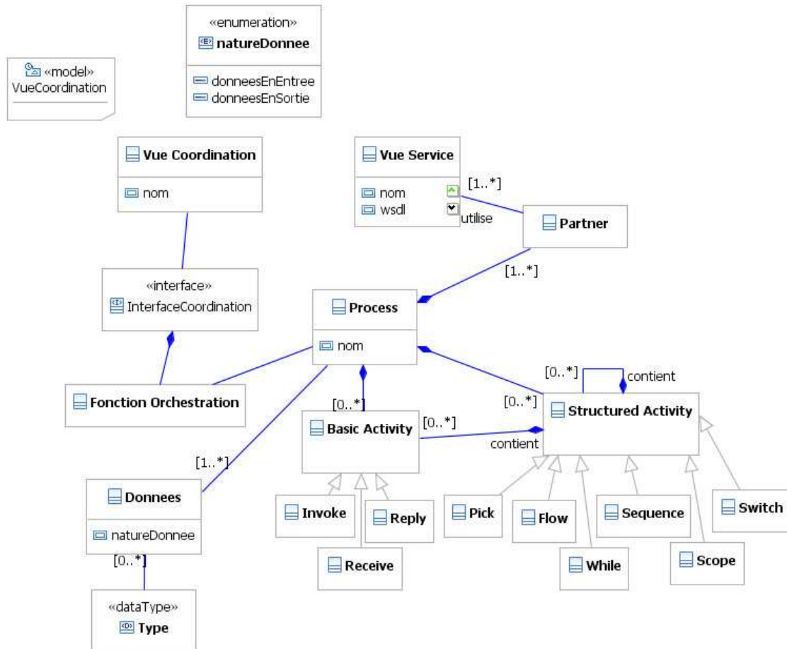
Figure 5.5. : Le méta-modèle de la vue coordination et service
