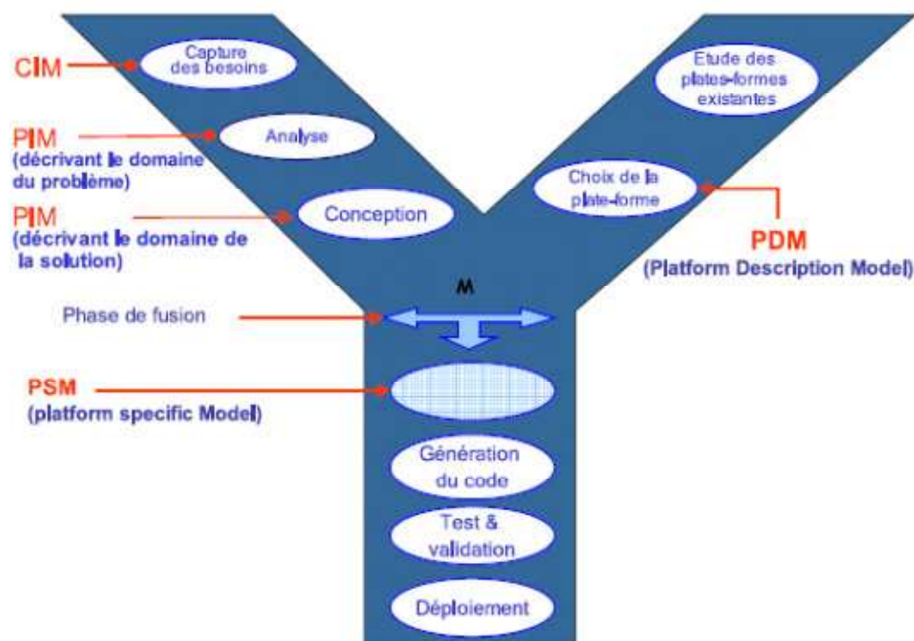
Figure 3.6. Le cycle de vie en Y
