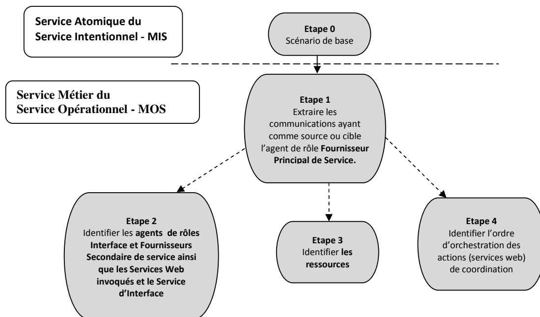
Figure 4.11. Le processus de découverte du Service Métier à partir du but du Service Atomique
