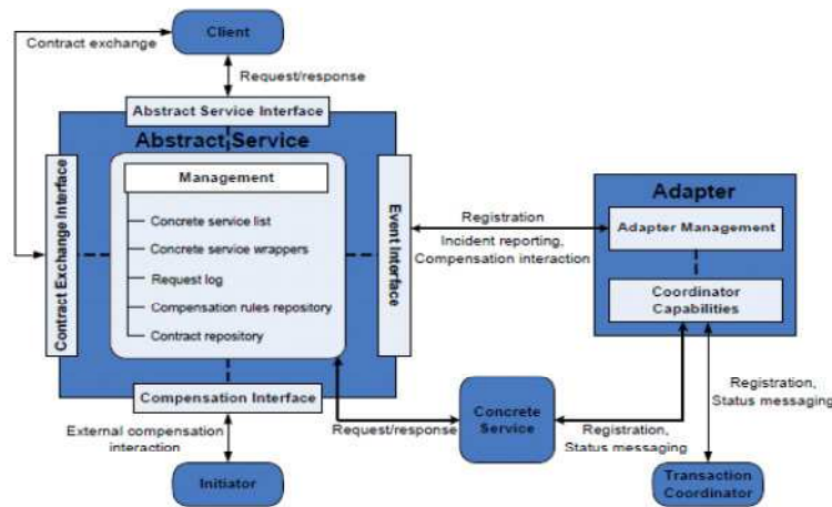
Figure 2.4. Le service abstrait et l'environnement de transaction adaptateur
