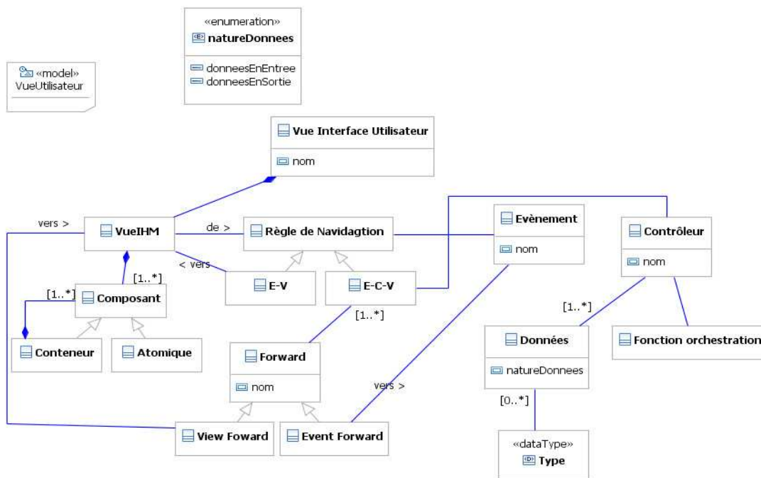
Figure 5.4. : Le méta-modèle de la vue Interface Utilisateur
