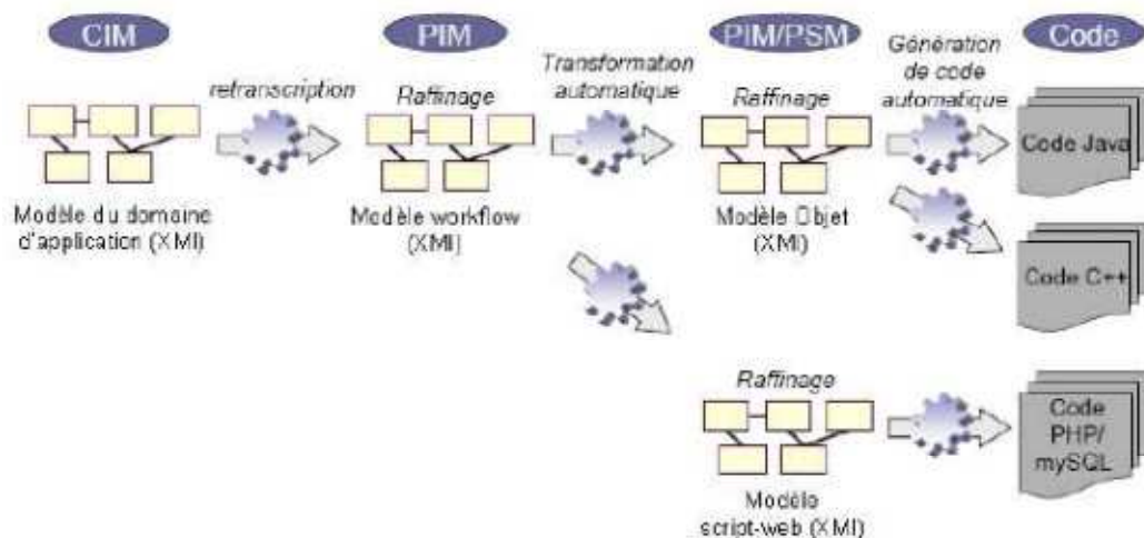
Figure 3.5. Le cycle de vie de MDA
