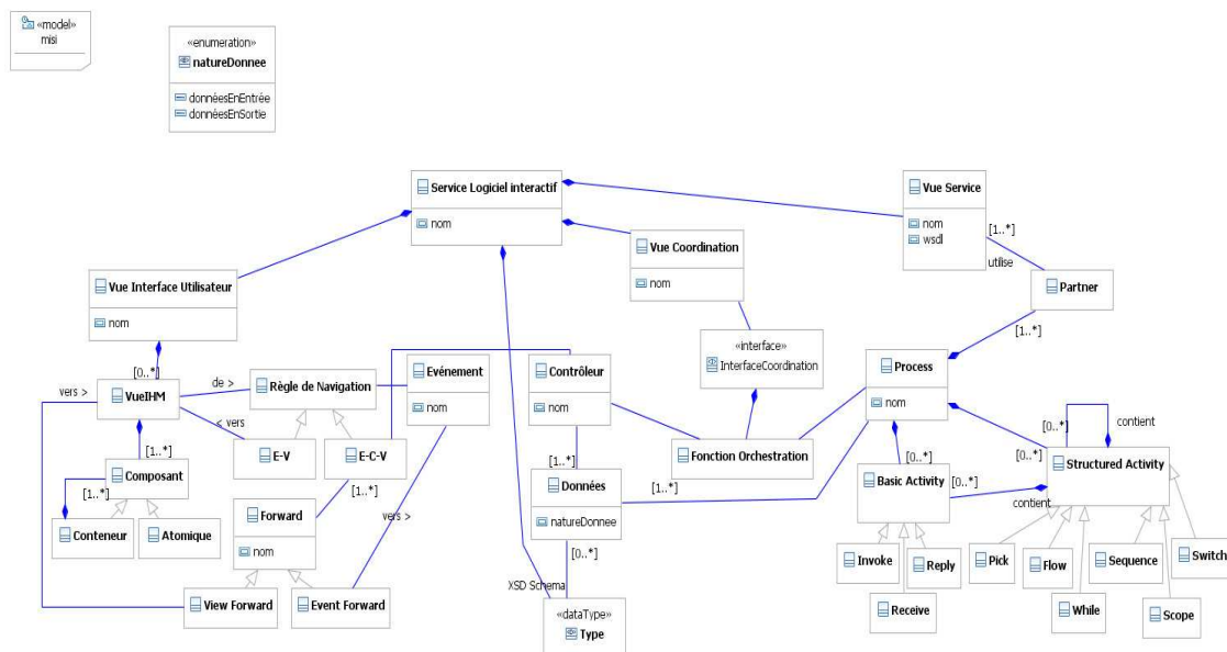
Figure 5.3. : Le méta-modèle du modèle MISI
