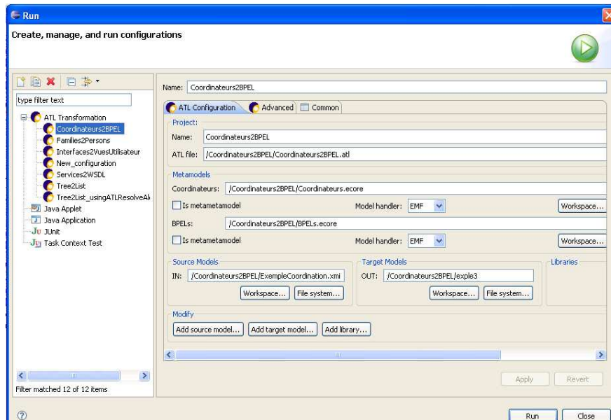
Figure 5.15. : Exécution d'une transformation avec ATL©
