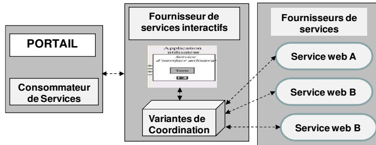
Figure 5.7. : Présentation d'une architecture 3-tier de service interactif
