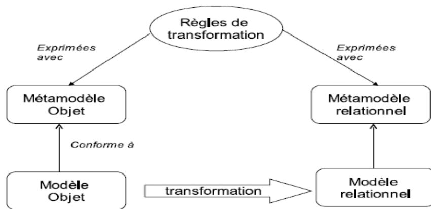
Figure. 3.4. Migration de modèle objet à un modèle relationnel
