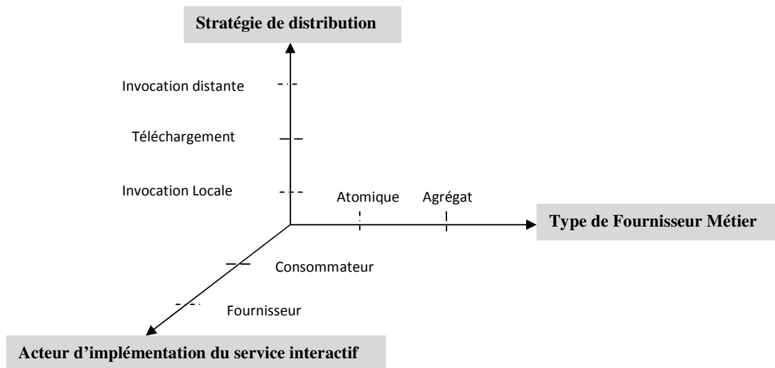
Figure 5.2. : Attributs des facettes architecturales
