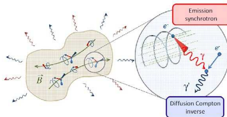
FIG. VI.13 – Illustration du processus de Synchrotron Self Compton.
