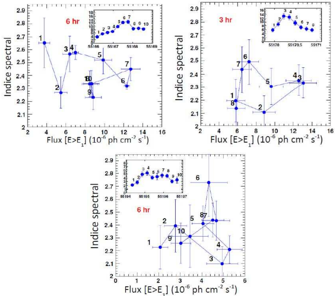
FIG. VII.17 – Indice spectral versus flux ( E > E_1 ) pour les éruptions MJD 55167, MJD 55170, et MJD 55195. Les numéros mettent en évidence l'évolution temporelle. Les courbes de lumière correspondantes sont affichées en encarts.
