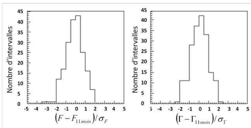
FIG. VIII.9 – Distribution normalisée en flux (gauche) et indice spectral (droite) pour une réalisation donnée de source constante avec \Gamma = 2.4 et F_{100}=5 .
