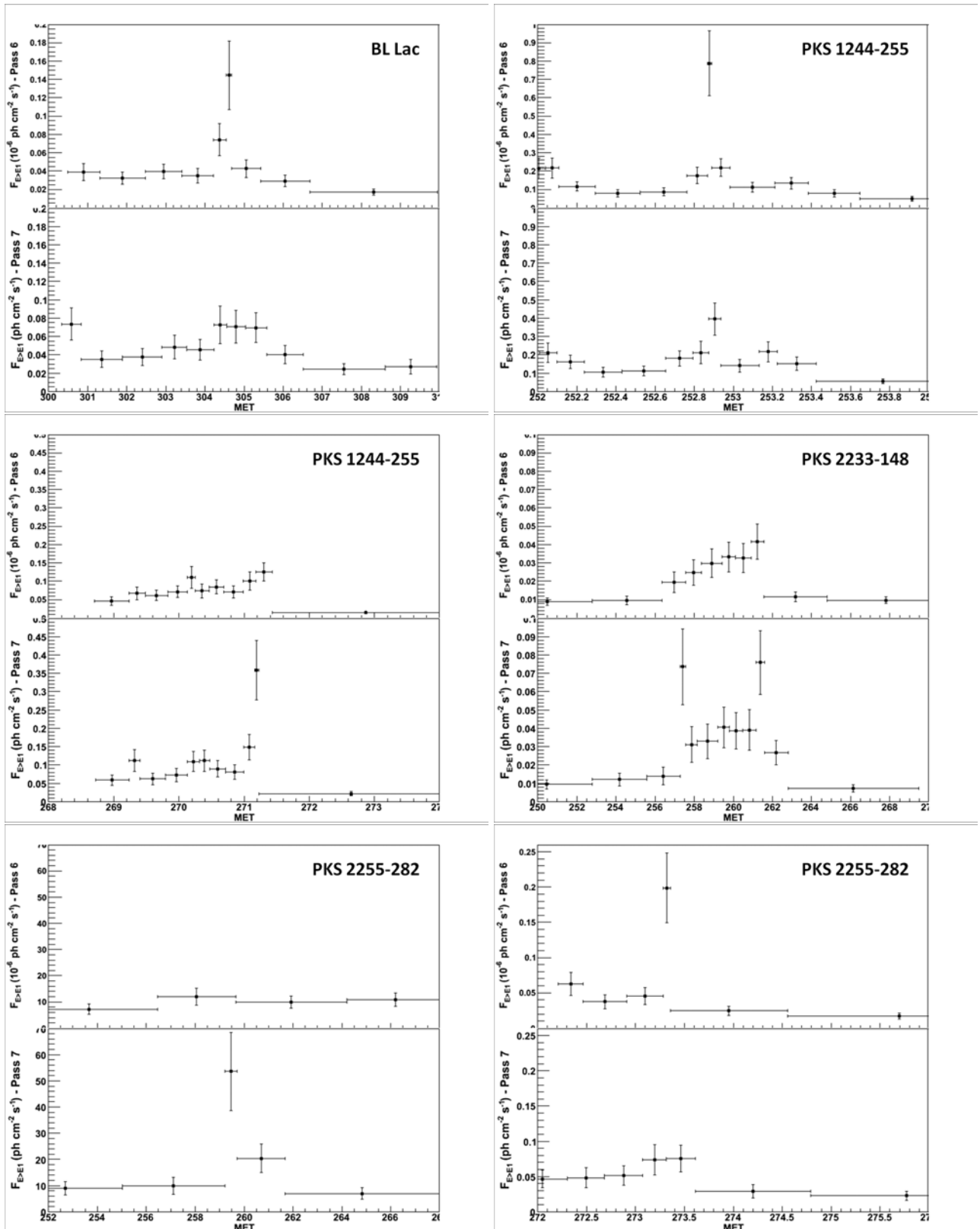
FIG. VIII.28 – Comparaison des LCs obtenues avec les données Pass 6 et Pass 7 à travers divers agrandissements réalisés sur les sources suivantes : BL LAC , PKS 1244-255 , PKS 2233-148 et PKS 2255-282 . Les flux représentés sont ceux issus de l'étape M2 .
