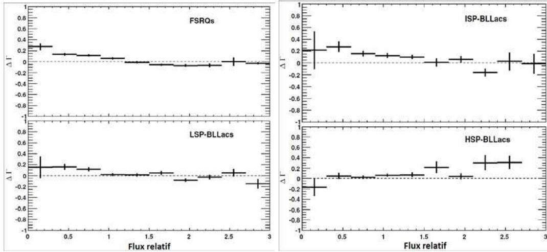
FIG. VI.18 – Variation moyenne de l'indice spectral \Gamma en fonction du flux relatif (normalisé au flux moyen) pour les différentes classes de blazars. De haut en bas et de gauche à droite : FSRQs, LSPs, ISPs, HSPs. Les données sont intégrées sur des périodes d'une semaine. Les 8 sources les plus brillantes de chaque catégorie, contenues dans LBAS, ont été considérées pour l'analyse. Figure extraite de Abdo et al. (2009f).
