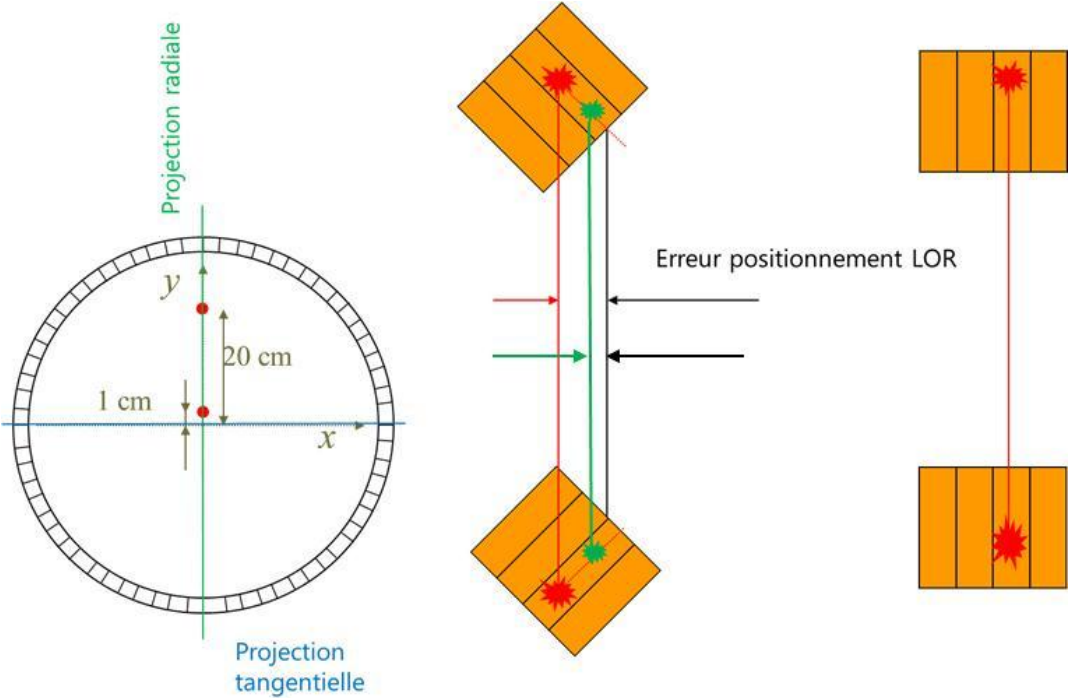
Figure 28 : La résolution spatiale : composante radiale et tangentielle.
