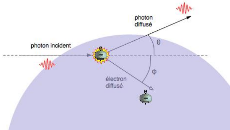
Figure 6 : La diffusion Compton 7 .
