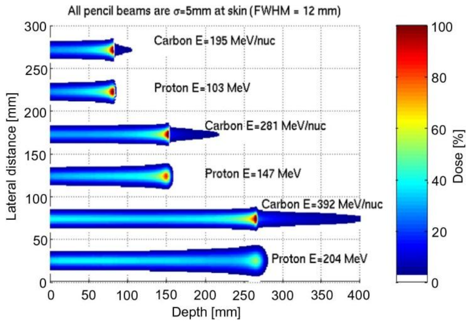
Figure 12 : La dose déposée par les protons et ions carbone dans l'eau (Suit et al. , 2010).
