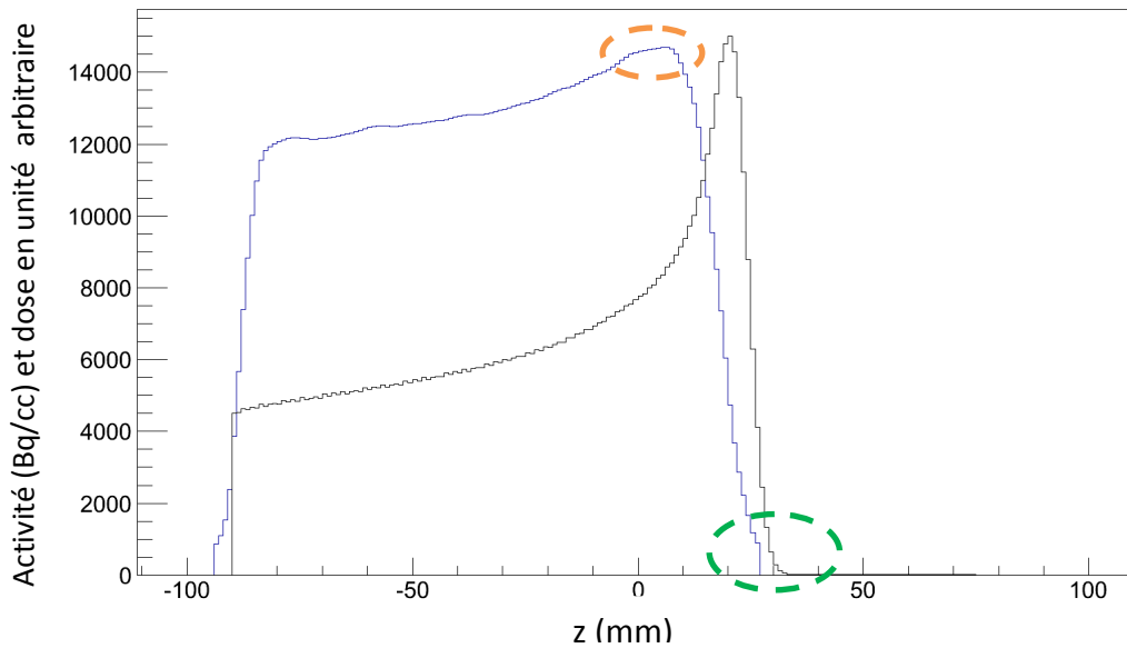
Figure 80 : Le profil TEP avec un seuil de 5 % de l'activité maximale, les pointillés oranges désignent la position où la section efficace est maximale et les pointillés verts désignent la pénombre distale de la dose déposée.
