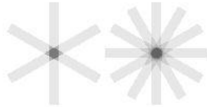
Figure 25 : Le principe de rétroprojection de la distribution d'activité à partir de ces projections, à gauche la reconstruction se fait à partir de 6 projections et à droite à partir de 12 projections.
