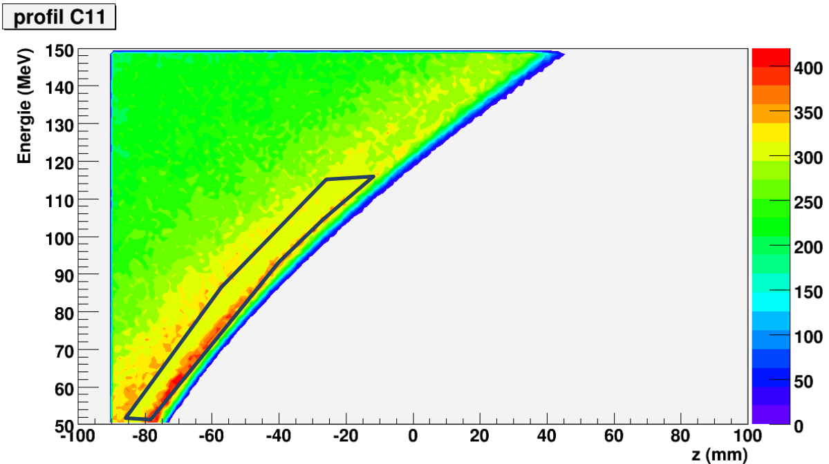
Figure 48 : Les intensités des profils de productions de ^{11}\text{C} de 50 à 150 MeV sans modification du modèle de cascade binaire. L'échelle de couleur correspond au nombre de ^{11}\text{C} formés pour 10 millions de protons simulés par pas 1 MeV entre 50 et 150 MeV.
