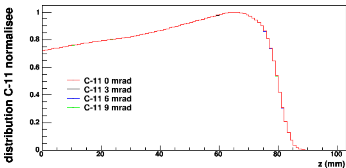
Figure 43: Les profils de C-11 normalisés en profondeur pour 4 dispersions angulaires différentes.
