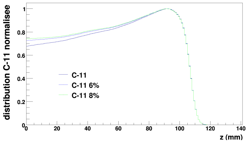
Figure 39 : Le profil non normalisé et normalisé des 11 C dans du PMMA à 134,7 MeV.
