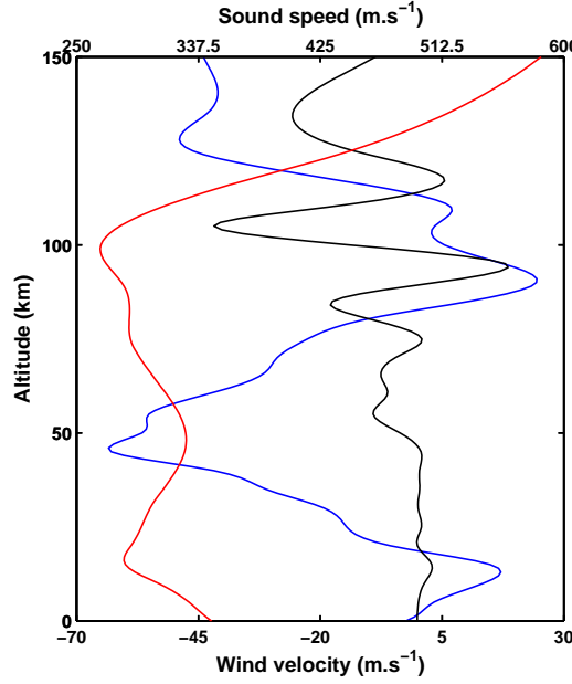
FIGURE 3.4 – Modèle atmosphérique HWM07 utilisé pour les tests de validation numérique. La courbe rouge représente la vitesse du son, la courbe bleue le vent zonal et la courbe noire le vent méridien.
