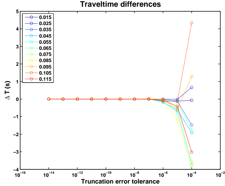
FIGURE 3.6 – Influence de la tolérance sur l’erreur de troncature et de la valeur du paramètre d’intégration (traits colorés) sur le calcul du temps de trajet pour un rayon d’angle d’incidence fixé à 65^\circ et d’azimut 70^\circ .
