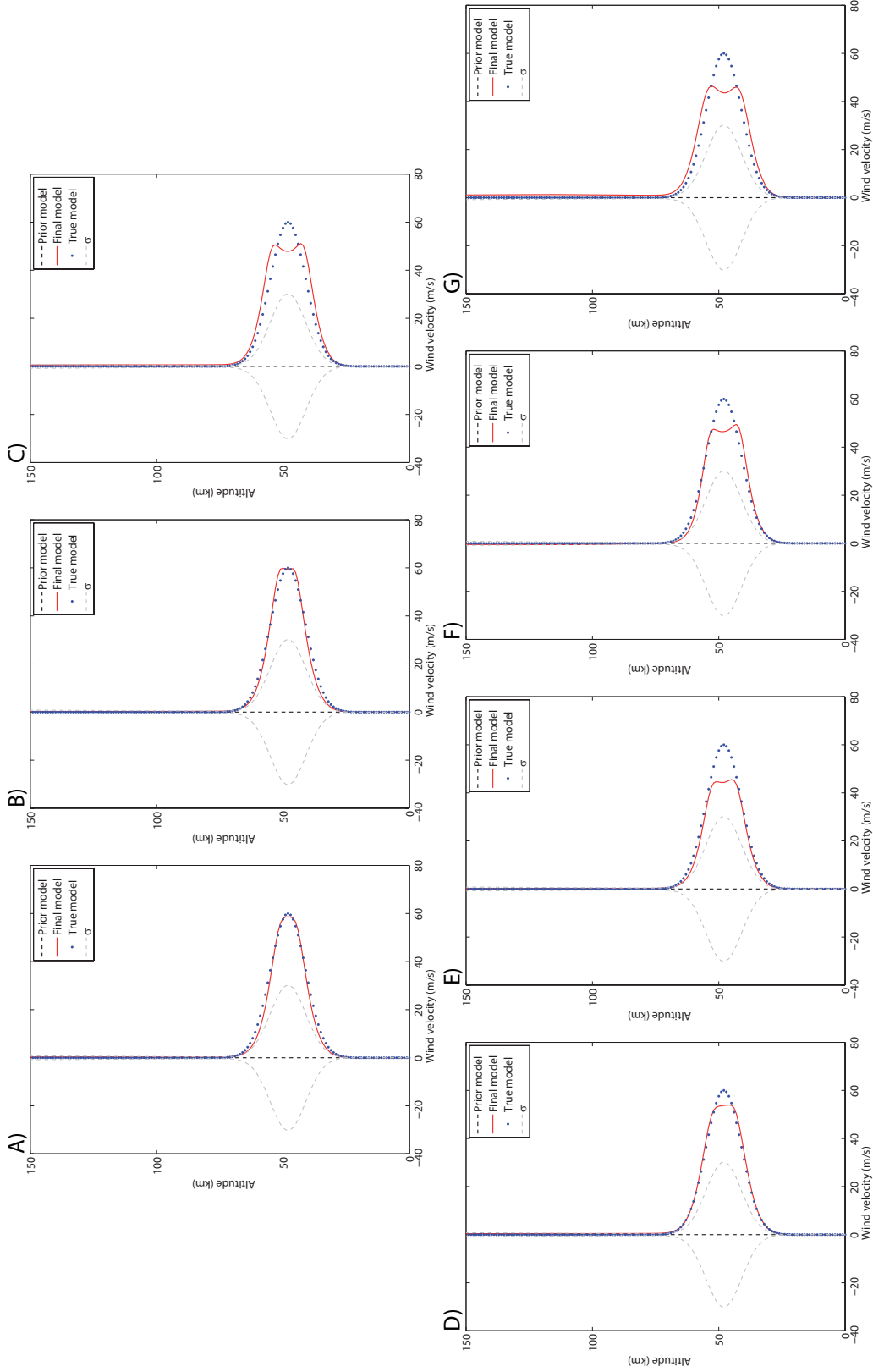
FIGURE C.1 – Inversion de données dégradées par un bruit gaussien sur la vitesse de passage et l'azimut avec \sigma_{v_t} = 2 m/s et \sigma_\phi = 1^\circ (A), \sigma_{v_t} = 3 m/s et \sigma_\phi = 2^\circ (B), \sigma_{v_t} = 4 m/s et \sigma_\phi = 3^\circ (C), \sigma_{v_t} = 5 m/s et \sigma_\phi = 3^\circ (D), \sigma_{v_t} = 6 m/s et \sigma_\phi = 3^\circ (E), \sigma_{v_t} = 8 m/s et \sigma_\phi = 3^\circ (F), \sigma_{v_t} = 10 m/s et \sigma_\phi = 3^\circ (G).
