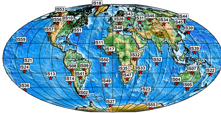
FIGURE 2.18 – Répartition des stations microbarométriques du réseau IMS.
