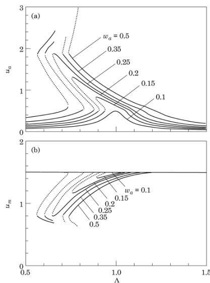
Figure 1.5. : Effet de la fluctuation de raideur w_a sur la partie fluctuante (a) et la valeur moyenne (b) de la résonance paramétrique principale du système. (—) Solutions stables. (....) Solutions instables. (Blankenship 1995 [33]).
