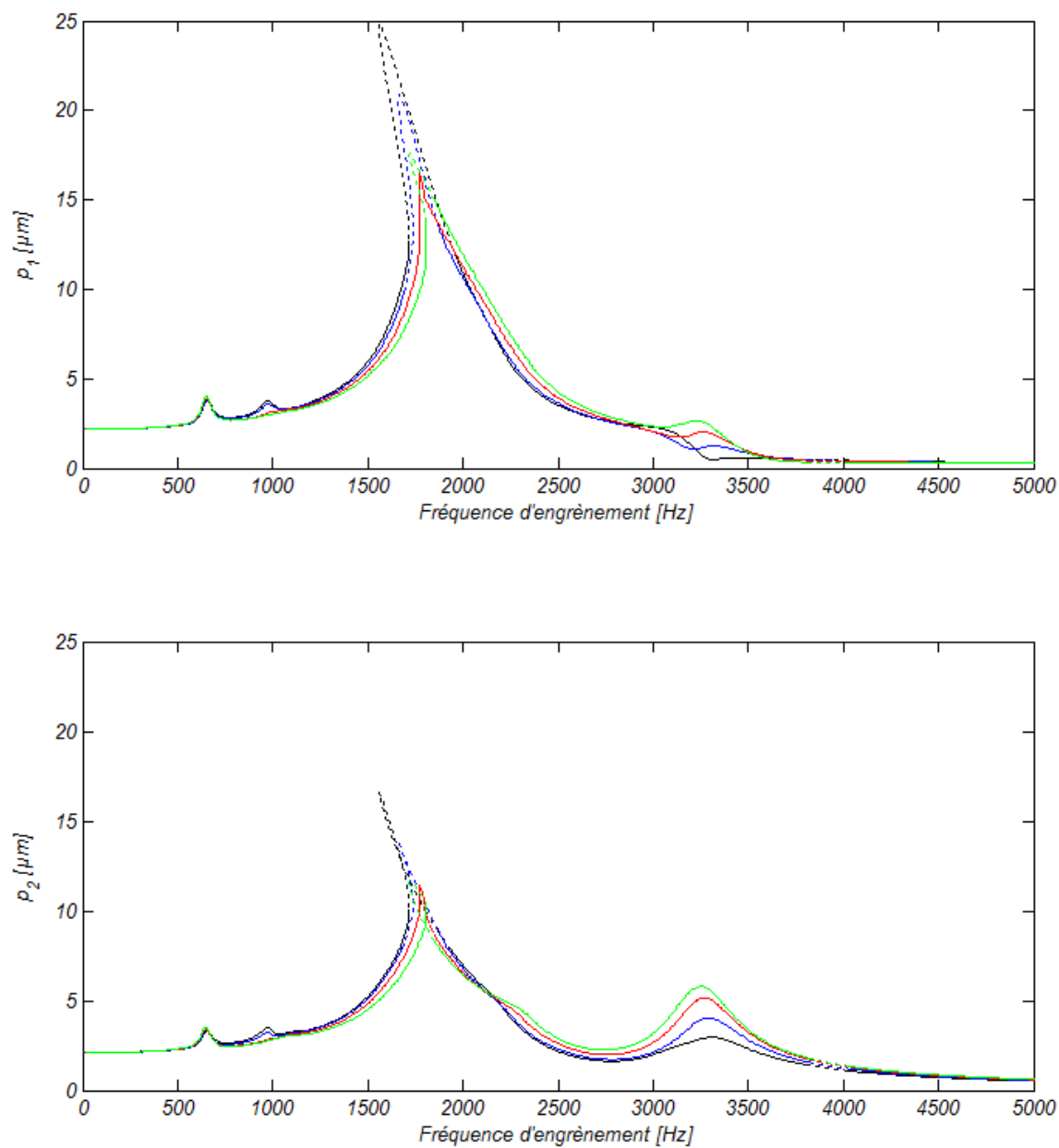
Figure 4.28. : Valeurs RMS des solutions 1-T périodique de la cascade 84-73-56 pour différentes valeurs de déphasage.
