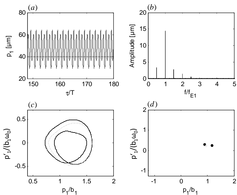
Figure 4.18. : Solution 2-T périodique avec 2 impacts par période, à f_{E1} = 1830 \text{ Hz} .
