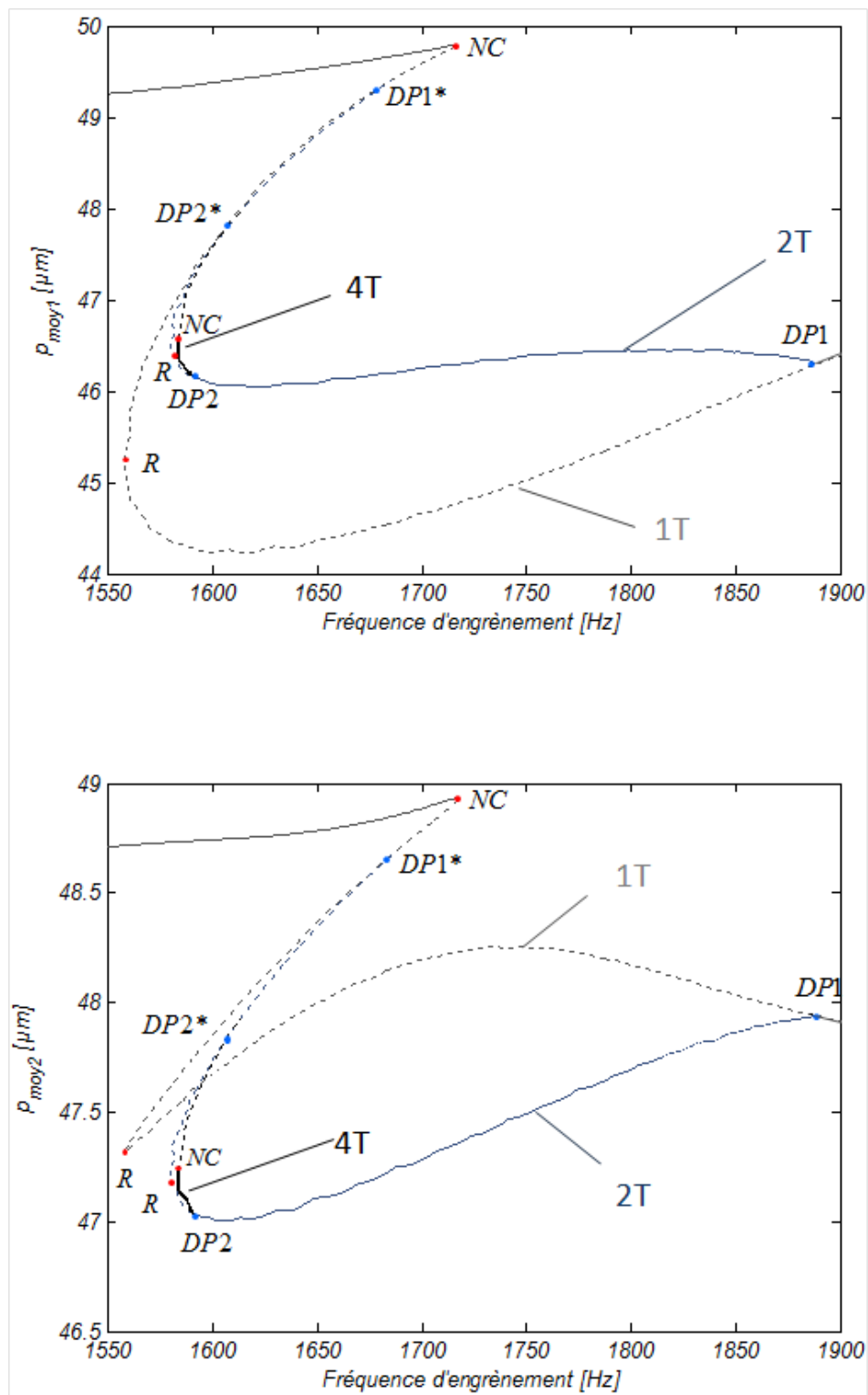
Figure 4.17. : Valeurs moyennes des réponses n-T périodiques des deux engrènements de la cascade 84-73-56 autour de la résonance principale.
