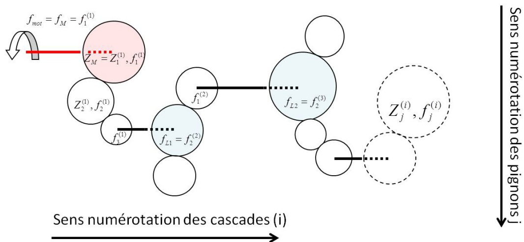
Figure 3.3. : Schéma général d'une transmission par engrenages.
