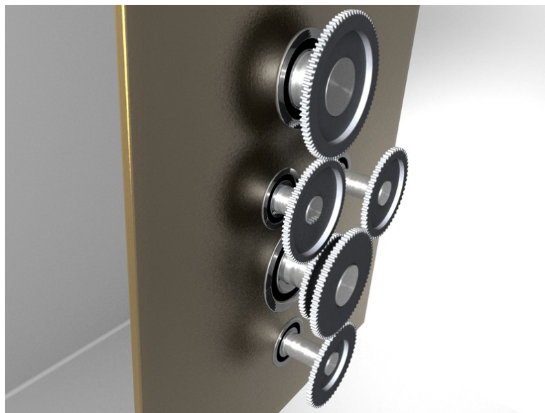
Figure 3.22. : Schéma de la cascade de dentures : arbres, pignons, roulements et plaque support.
