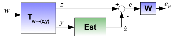
Figure 2.1 – Forme standard du problème d'estimation nominale
