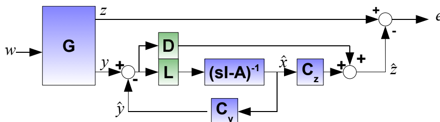
Figure 2.19 – Forme standard du problème de synthèse d'EGN sans pondération
