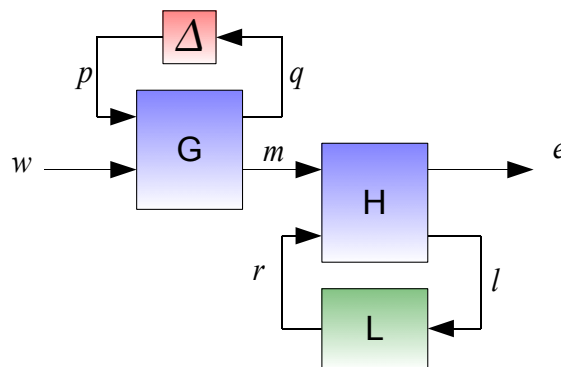
Figure 4.4 – Forme standard du problème de synthèse général d'estimateur robuste
