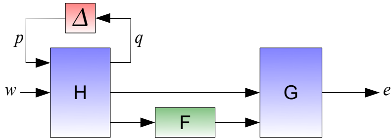
Figure 5.8 – Forme standard du problème de contrôle en boucle-ouverte (cas SEI)
