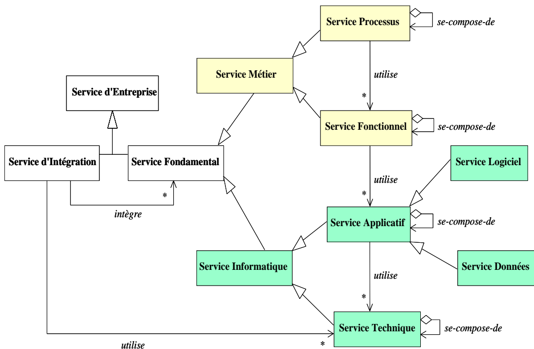
Figure VI.6. Typologie des services d'entreprise selon la nature
