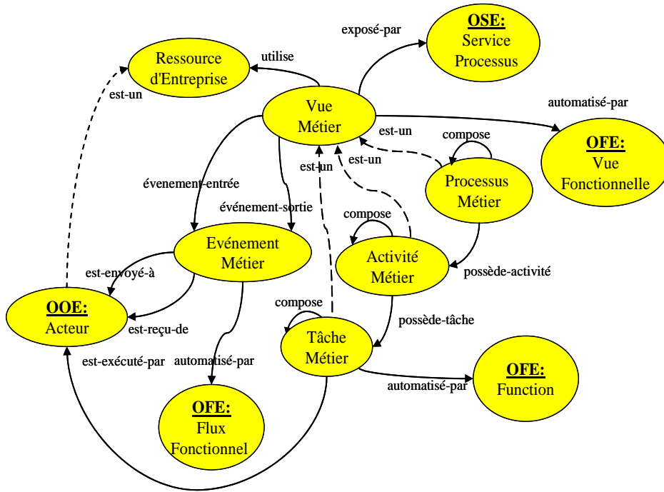
Figure VII.21. Ontologie métier d'entreprise (OME)
