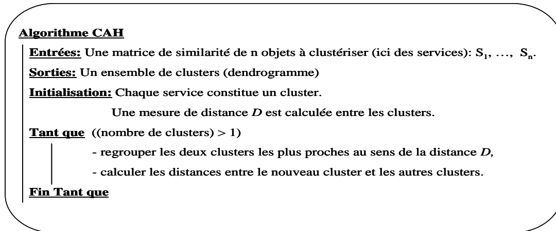
Figure VI.20. Principe de la classification ascendante hiérarchique
