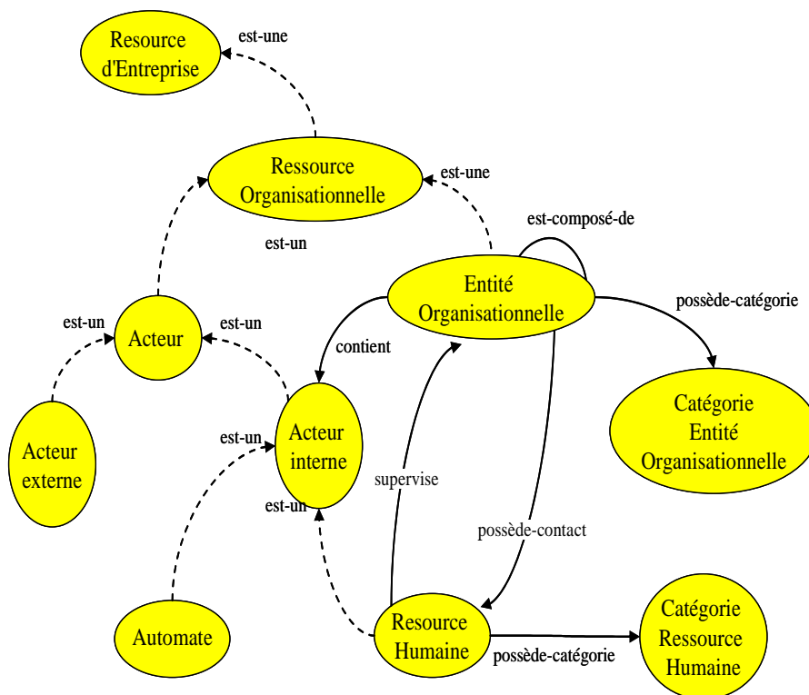
Figure VII.22. Ontologie organisationnelle d'entreprise (OEE)
