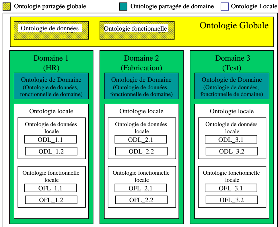
Figure VII.32. Urbanisation sémantique typique
