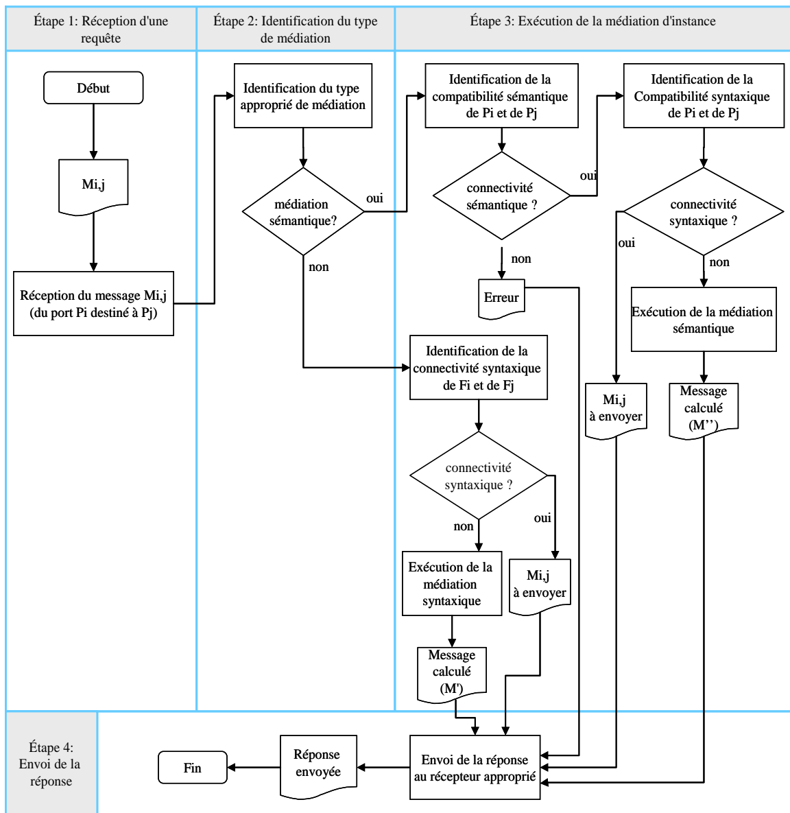
Figure VIII.26. Processus global du service de médiation de données
