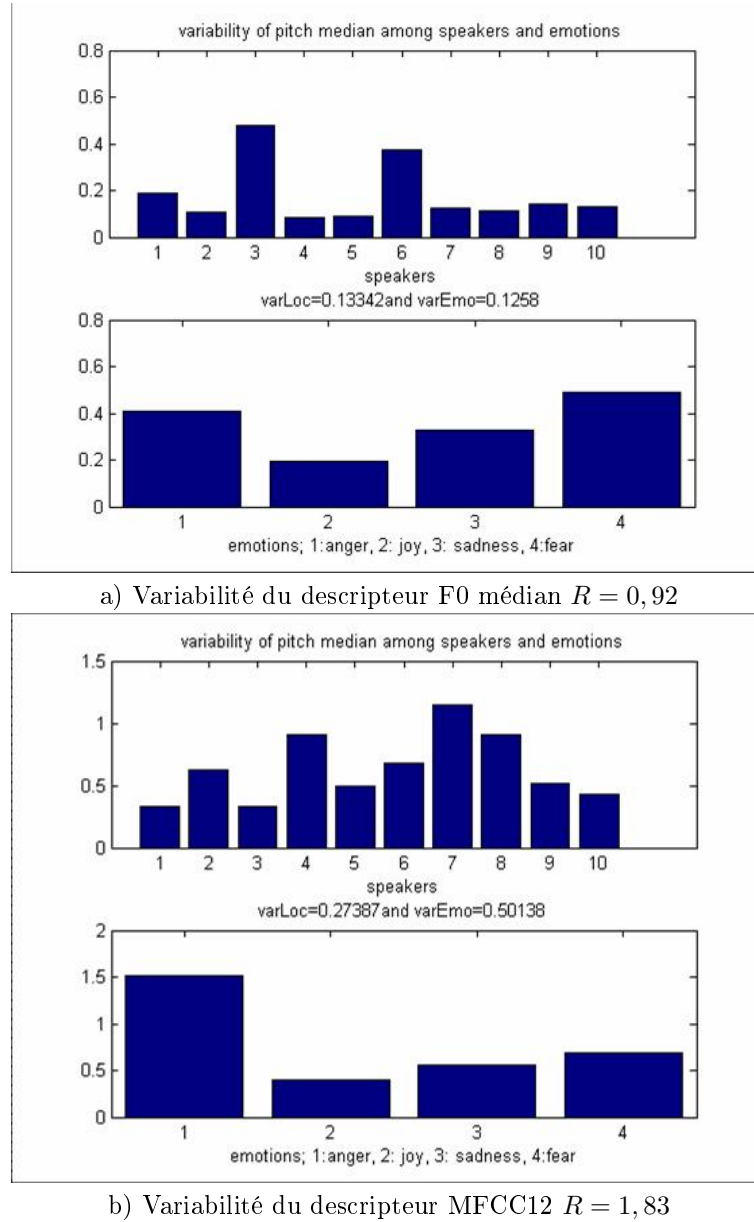
FIGURE 4.5 – Exemple de mesure de variabilité locuteur et émotion sur le corpus NAO-HR1 (10 locuteurs, 5 états émotionnels dont neutre) pour la F0 médiane (a) et le coefficient MFCC12 (b)
