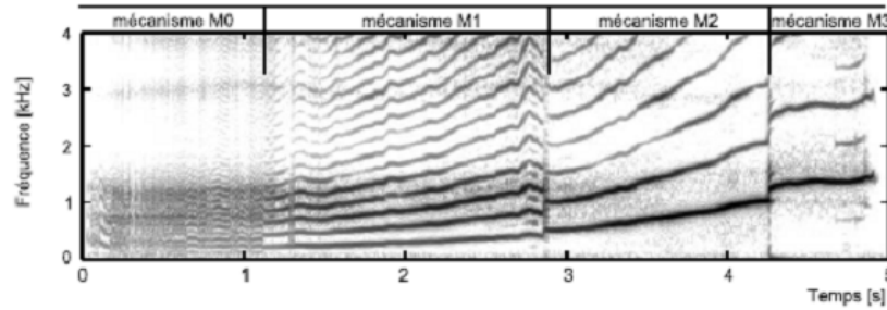
FIGURE 3.2 – Spectrogramme d'un glissando réalisée par une femme dans les 4 mécanismes vibratoires (adapté de [Roubeau et al. 09])
