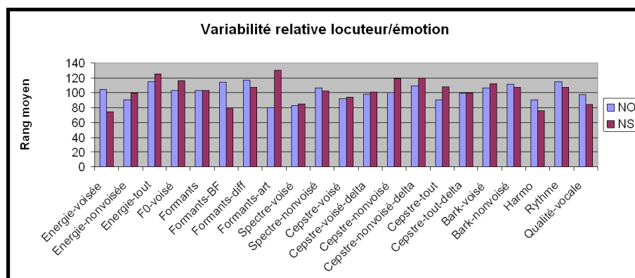
FIGURE 4.6 – Variabilité relative locuteur/émotion, influence de la normalisation locuteur et rang moyen par famille de descripteurs (NO : sans normalisation, NS : normalisation locuteur) sur l’ensemble des corpus Romeo (tableaux B1, B2).
