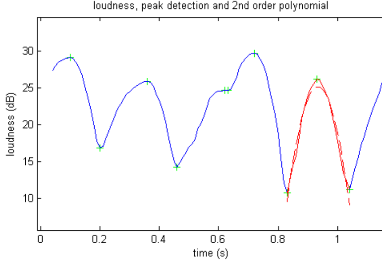
FIGURE 4.1 – Courbe de loudness et sa modélisation au niveau d'un noyau syllabique par un polynôme d'ordre 2.
