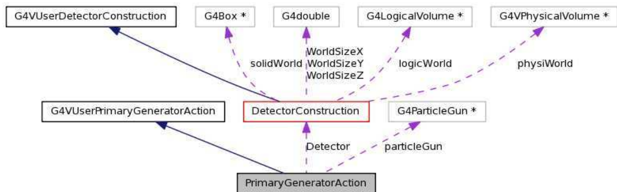
Figure 4 : Diagramme de la classe PrimaryGeneratorAction qui dérive de la classe G4UserPrimaryGeneratorAction et utilise la classe la classe DetectorConstruction , qui dérive de G4UserDetectorConstruction .
