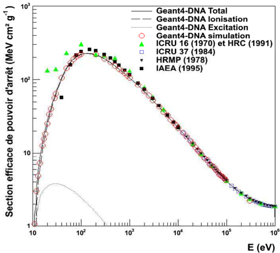
Figure 8: Pouvoirs d'arrêt massiques calculés à partir des sections efficaces d'ionisation et d'excitation de Geant4-DNA représentés par les courbes. La courbe pleine est la somme du pouvoir d'arrêt dû au processus d'ionisation (courbe en tirets) et du pouvoir d'arrêt dû à l'excitation (courbe en pointillés). Les valeurs du pouvoir d'arrêt résultant de la simulation en utilisant la méthode du régime stationnaire avec Geant4-DNA sont représentées par les cercles. Elles sont comparées aux recommandations pour l'eau liquide données par les rapports ICRU 16 [ICRU 16, 1970], ICRU 37 [ICRU 37, 1984], par le Handbook of Radiation Chemistry [HRC, 1991], par le Handbook of Radiation Measurement and Protection [HRMP, 1978], et par le rapport IAEA-TECDOC-0799 [IAEA, 1995].
