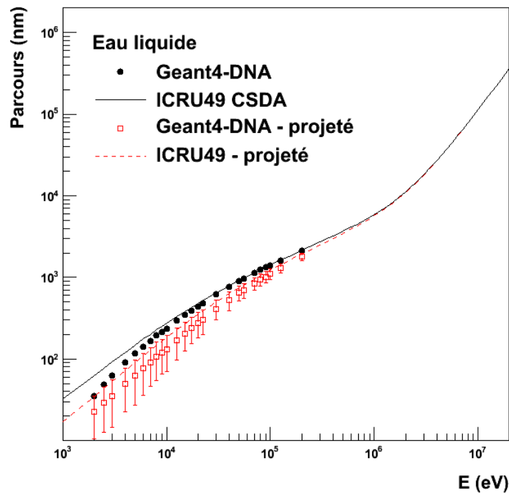
Figure 27 : Comparaison des valeurs du parcours et du parcours projeté de l'hélium et de ses états de charge obtenus avec le processus de diffusion élastique donné par Geant4-DNA pour l'eau liquide et les données de l'ICRU 49 [ICRU 49, 1993] pour l'eau liquide. Nous avons indiqué les barres d'erreur RMS des valeurs projetées simulées.
