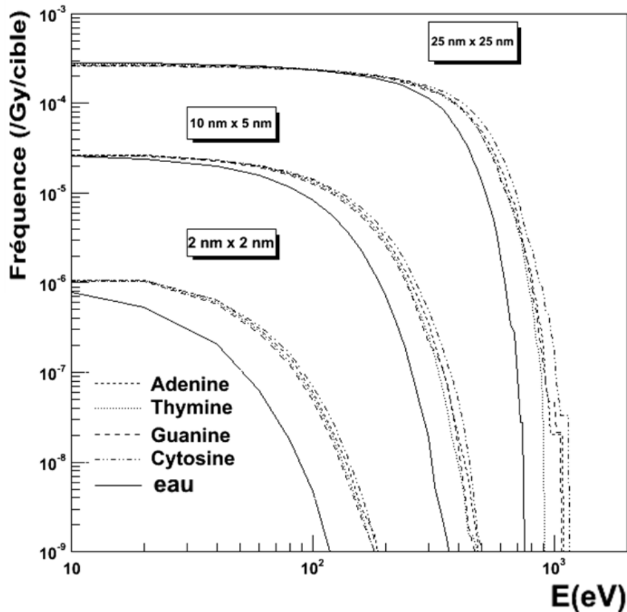
Figure 21 : Fréquences des dépôts d'énergie par cible cylindrique et par Gray dans les géométries cylindriques de dimensions 25\text{ nm} \times 25\text{ nm} , 10\text{ nm} \times 5\text{ nm} et 2\text{ nm} \times 2\text{ nm} , remplis d'eau liquide ou de base d'ADN (A, T, G, C).
