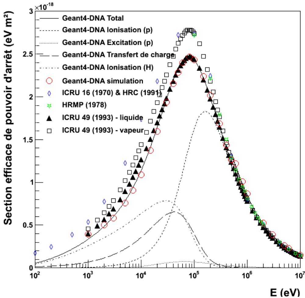
Figure 13: Section efficace de pouvoir d'arrêt calculée à partir des sections efficaces d'ionisation, d'excitation et de changement de charge du proton et de l'hydrogène (trait plein). Les valeurs de la section efficace de pouvoir d'arrêt résultant de la simulation du suivi des protons et atomes d'hydrogène avec Geant4-DNA sont représentées par les cercles. Ces valeurs sont comparées aux recommandations pour l'eau liquide données par le rapport ICRU 16 [ICRU 16, 1970] et par le Handbook of Radiation Chemistry [HRC, 1991], par le Handbook of Radiation Measurement and Protection [HRMP, 1978] et par le rapport ICRU 49 [ICRU49, 1993].
