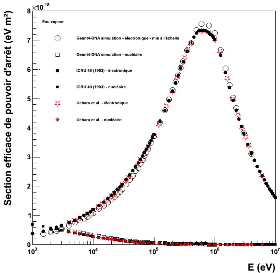
Figure 25 : Sections efficaces de pouvoir d'arrêt électronique mises à l'échelle pour l'eau en phase vapeur et nucléaire résultant de la simulation du suivi des atomes d'hélium et de leurs états de charge avec Geant4-DNA ; carrés ouverts (pour le seul processus de diffusion élastique) et cercles ouverts (pour tous les autres processus de Geant4-DNA). Ces valeurs sont comparées à la section efficace de pouvoir d'arrêt nucléaire (carrés pleins) et à la section efficace de pouvoir d'arrêt électronique (cercles pleins) de l'ICRU 49 [ICRU 49, 1993] pour l'eau de vapeur et aux calculs de [Uehara et al. , 2002].
