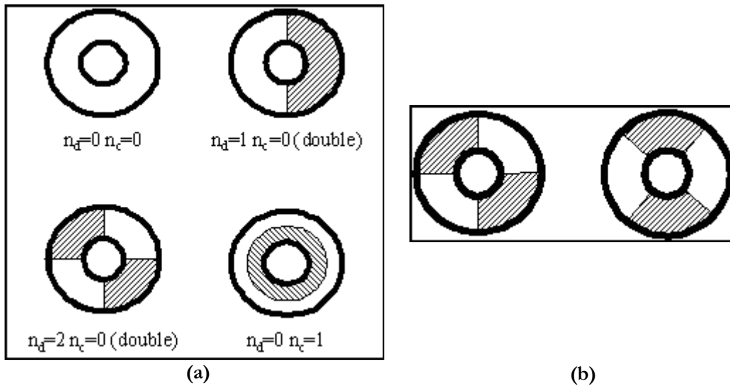
Figure I- 8 : (a) Modes normaux théoriques d'une plaque circulaire encadrée en son rayon intérieur. n_d représente le nombre de diamètres nodaux et n_c le nombre de cercles nodaux. (b) Représentation des modes doubles n_d=2 et n_c=0 . Ces deux modes sont déphasés spatialement de 45^\circ . Les modes possédant un nombre de diamètres nodaux non nuls sont doubles (théoriquement).
