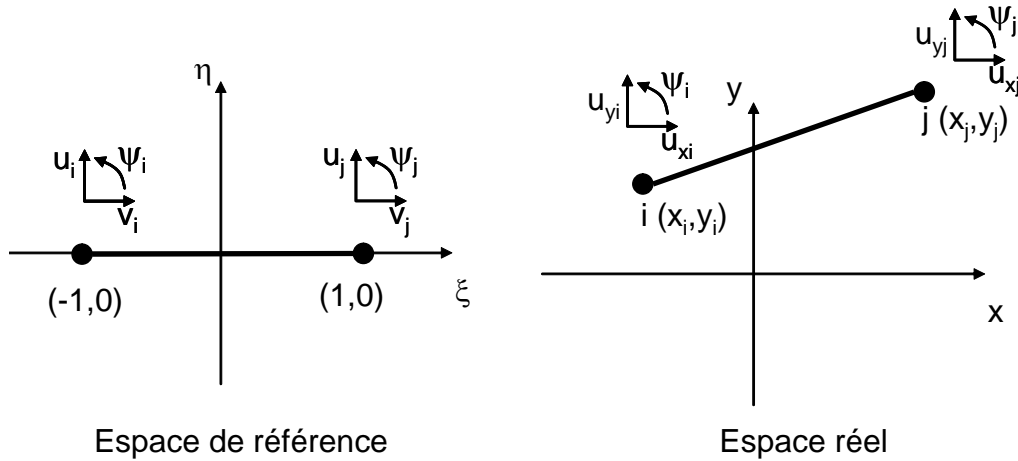
Figure II - 3 : Elément fini choisi pour la discrétisation spatiale de \Omega_1 et \Omega_2 . L'élément fini est présenté dans l'espace de référence et dans l'espace réel.
