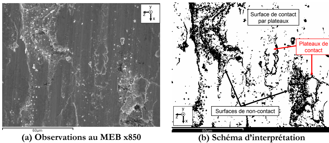
(a) Observations au MEB x850 (b) Schéma d'interprétation Figure IV- 20 : Surface de contact de la poutre \Omega_2 dans la zone de frottement.
