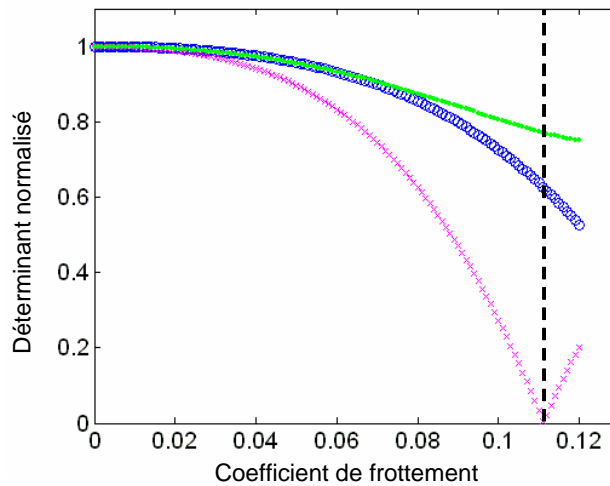
Figure B- 6: Déterminant (normée par rapport à la trace) de la sous-matrice 2x2 de K_g en fonction du coefficient de frottement correspondant aux modes ② et ③ (○), aux mode ⑤ et ⑥ (×) et aux modes ⑧ et ⑩ (●)
