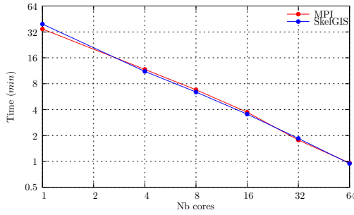
(a) Test 1 - temps d'exécution
