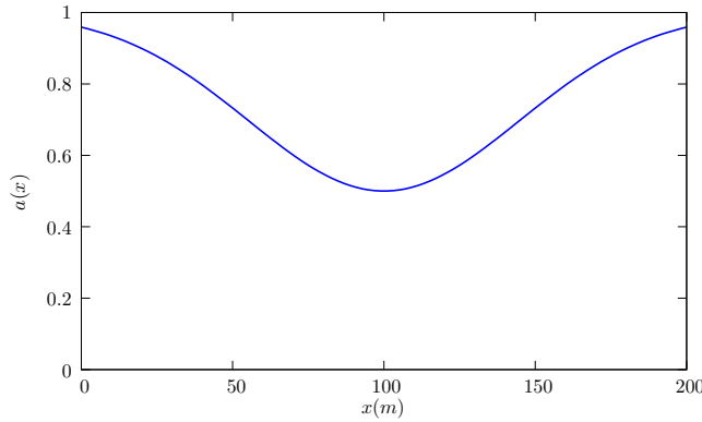
(a) La fonction a(h) = a(x) associée
