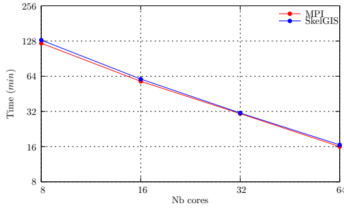
(e) Test 3 - temps d'exécution
