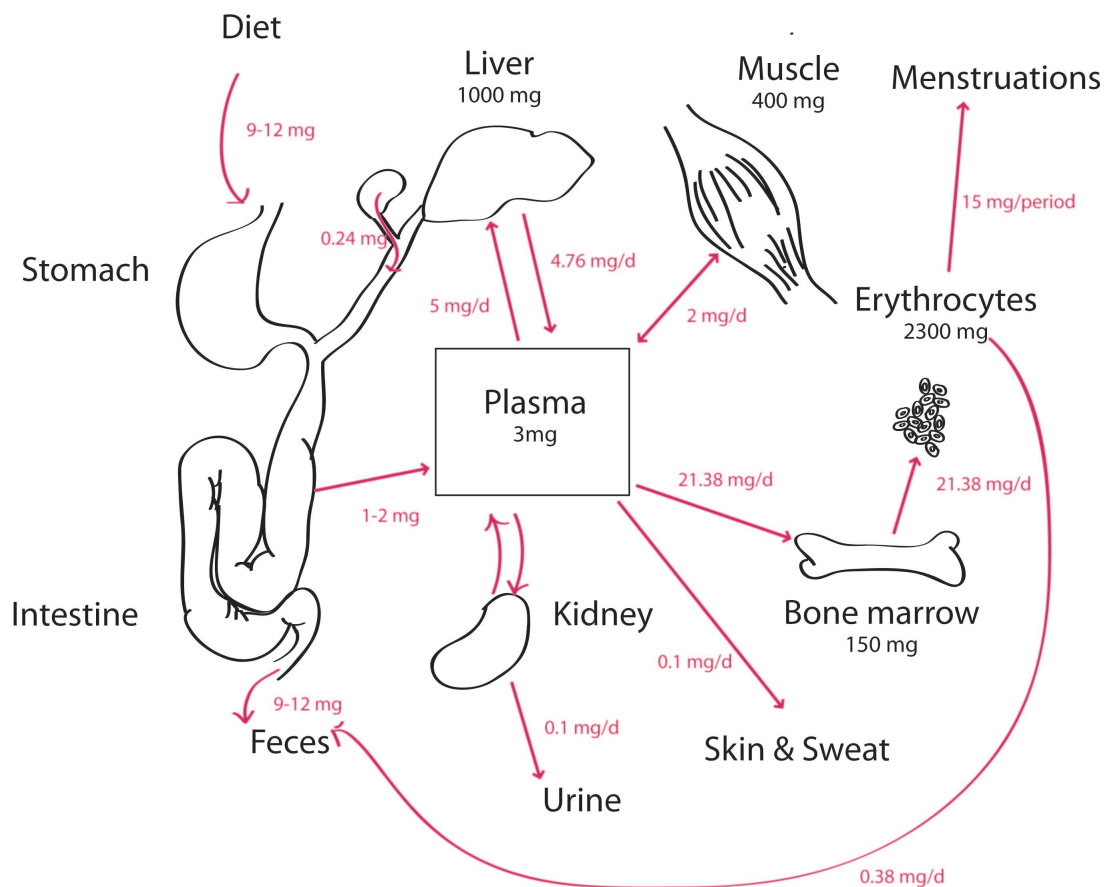
FIGURE 3.2.1: Cycle métabolique du fer. Diet=Bol alimentaire, Stomach=Estomac, Kidney=Rein, Liver=Foie, Intestine=Intestin, Bone marrow=moëlle osseuse.
