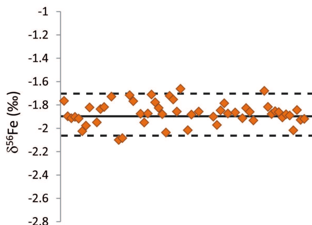
FIGURE 9.1.1: Reproductibilité externe « machine » d'un échantillon de sang de mouton (3H, n=53 ). La ligne noire représente la valeur moyenne. Les lignes pointillées délimitent la zone des échantillons compris entre la moyenne \pm deux écart-types. Les valeurs données ici tiennent compte de celles obtenues lors de mauvais réglages.
