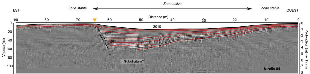
Figure 6-25. Radargramme du tronçon Mirella - 84 au Cirque des Graves.
