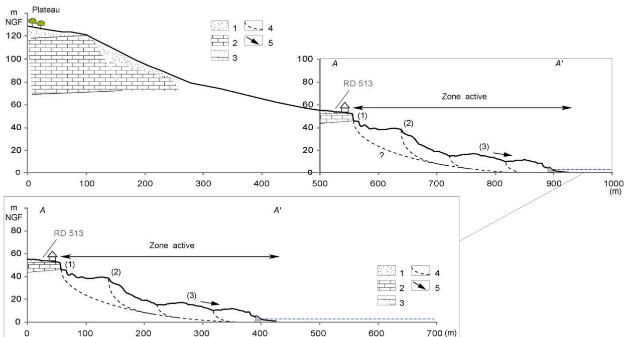
(1) Dépôts de pente, (2) Craie, (3) Calcaire gréseux, (4) Surface de rupture supposée, (5) Vecteur de déplacement.
