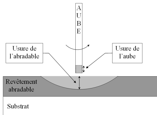
FIGURE 1.9 – Usure de l’aube et du revêtement abradable
