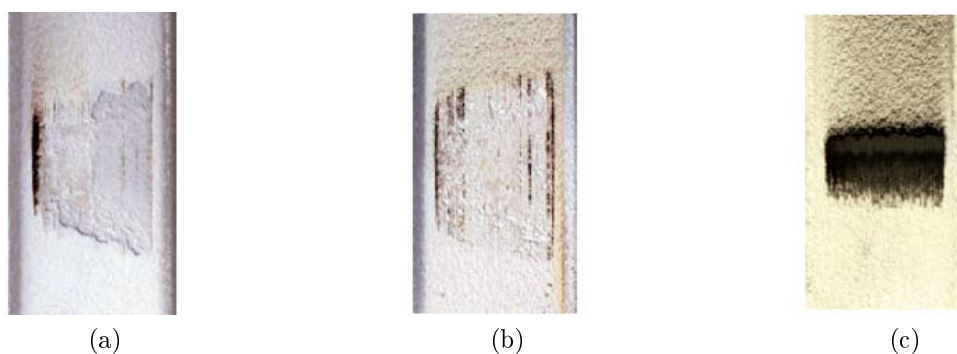
FIGURE 1.10 – Exemple d’échantillon d’abradable post-mortem (a) Décohésion, (b) Décohésion, coupe et léger transfert de matière, (c) Transfert de matière aube→abradable
