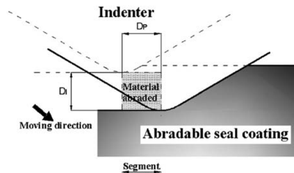
FIGURE 1.12 – Déplacement de l'indenteur lors des essais d'indentation [Ma 09]
