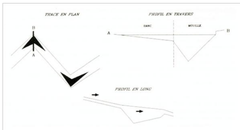
Figure 4.13. Illustration d'une mouille et d'un banc de convexité (Malavoi, 1989).
