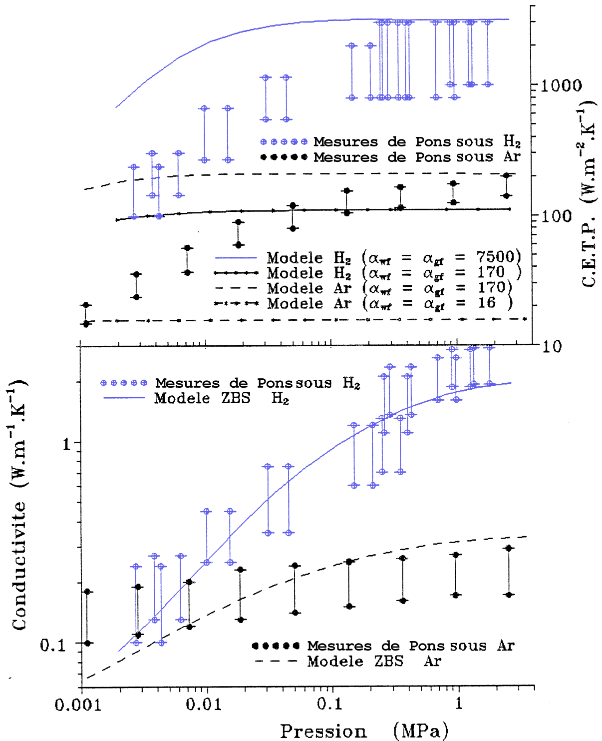
Fig. 8.6: Conductivité thermique effective (CTE) du lit et coefficient d'échange thermique à la paroi (CETP) pour le lit de LaNi 5 sous argon et sous hydrogène [37].
