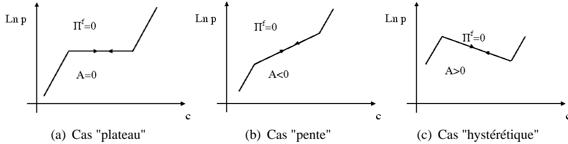
Fig. 6.3: Différentes évolutions de la pression d'équilibre vis-à-vis de la concentration en fonction du terme d'interaction de phase A .
