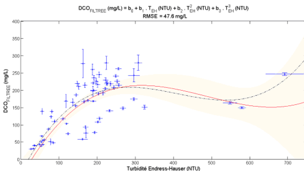
Figure III-18 : Exemple d'un intervalle de confiance à 95 % élargi pour les fortes valeurs
