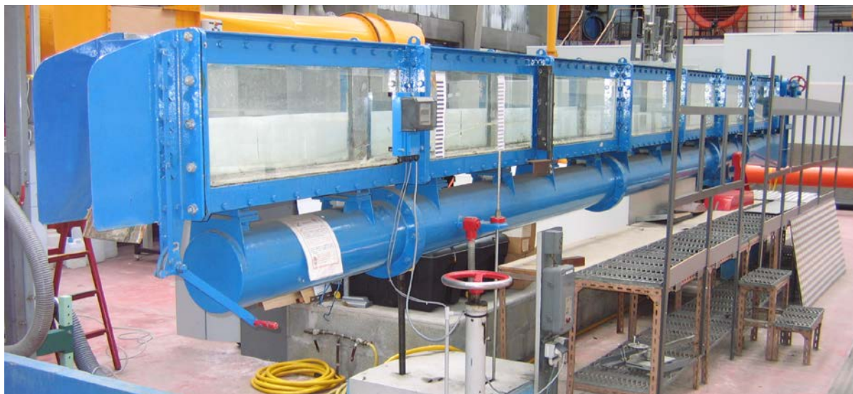
Photo II-1 : Banc hydraulique au LMFA (M. Lepot)
