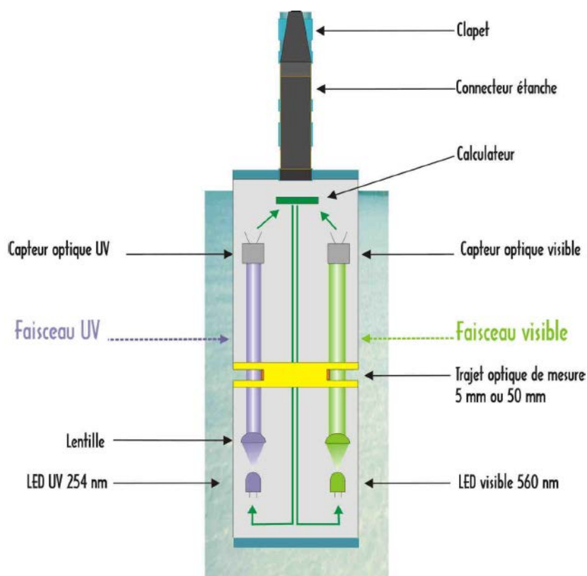
Figure II-6 : Schéma de la sonde EFS (EFS, 2010)
