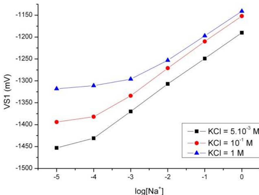
Figure 56: Courbes de calibration pour des concentrations de potassium variant de 5 \cdot 10^{-3} à 1 M
