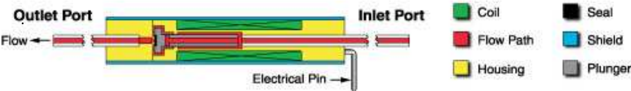
Figure 39: Coupe transversale d'une électrovanne [42]
