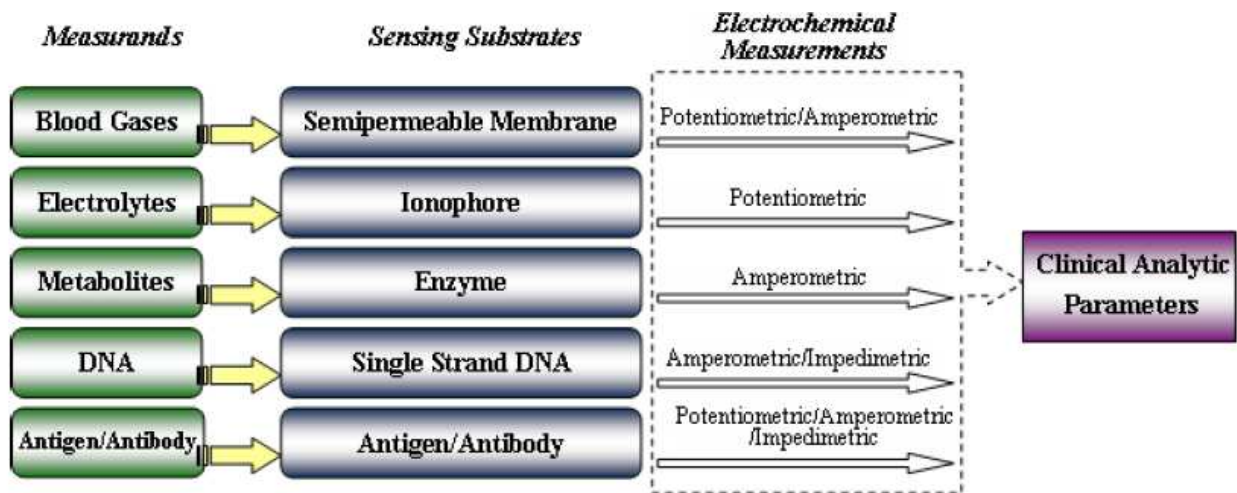
Figure 21: Correspondance entre les différents modes de transduction électrochimique et les mesurands dans le cas d'analyses cliniques [46]
