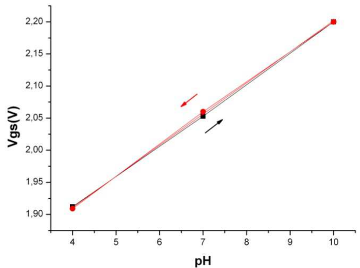
Figure 20: Sensibilité du capteur en fonction du pH
