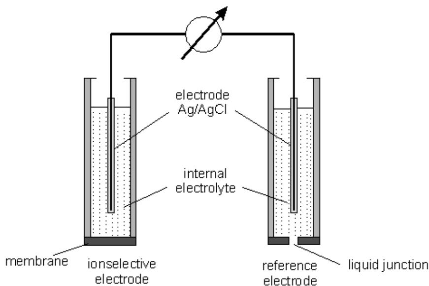
Figure 15: Schéma d'une mesure par électrode sélective ( http://csrg.ch.pw.edu.pl/tutorials/ise/ )
