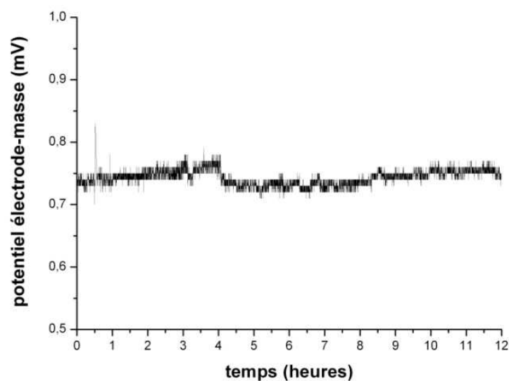
Figure 12: Potentiel électrode-masse
