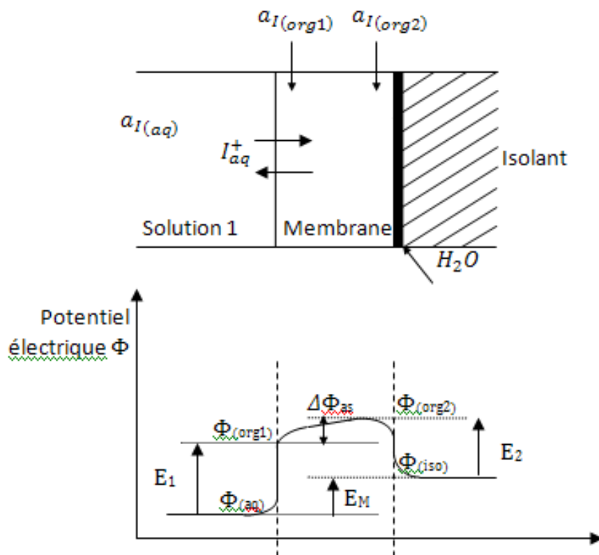
Figure 29: Equilibre dans une structure ChemFET asymétrique ( http://www.techniques-ingenieur.fr )
