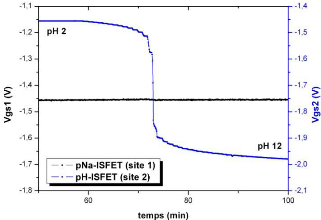
Figure 35: Réponse du pNa-ISFET et du pH-ISFET à une variation de pH de 2 à 12, à concentration en sodium constante (0,1M)
