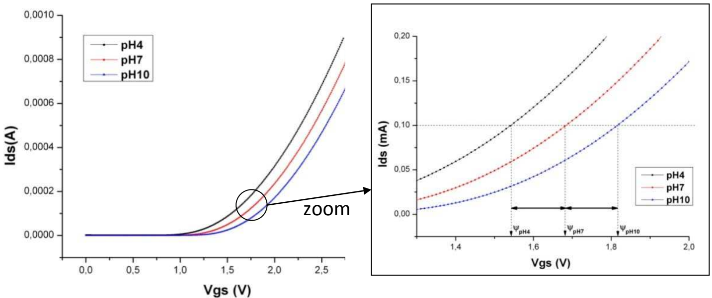
Figure 19: Caractéristiques I_{ds}=f(V_{gs}) de l'ISFET pour trois solutions de pH différents, polarisées par une électrode de référence Ag/AgCl commerciale
