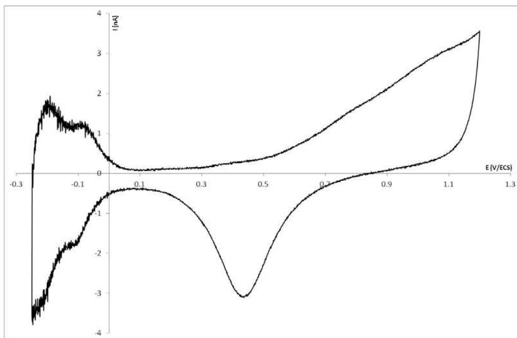
Figure 18: Exemple de voltammogramme effectué sur une électrode de platine [43]
