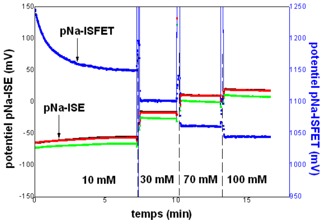
Figure 24: Réponses analytiques des ISE et des pNa-ISFET
