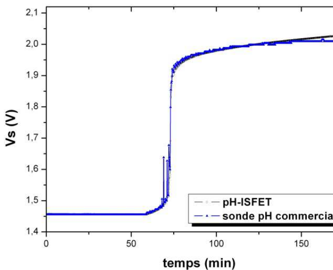
Figure 23: Tension de sortie du capteur pour une solution dont le pH varie de 2 à 12
