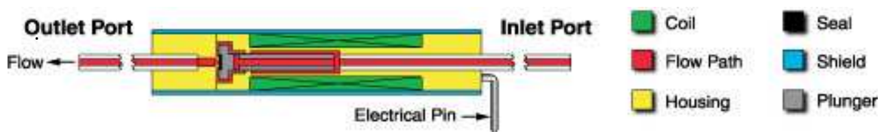
Figure 39: Coupe transversale d'une électrovanne [42]
