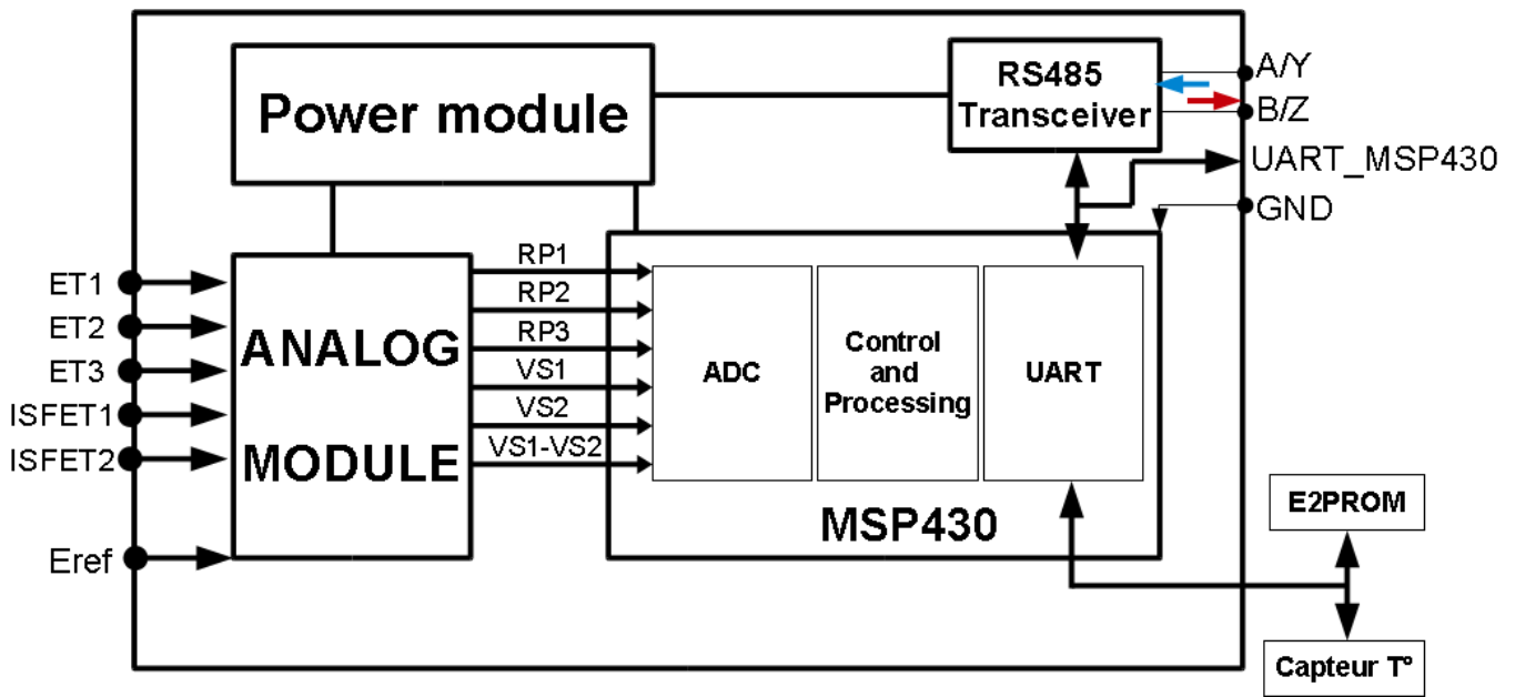
Figure 8: Architecture de la carte électronique embarquée
