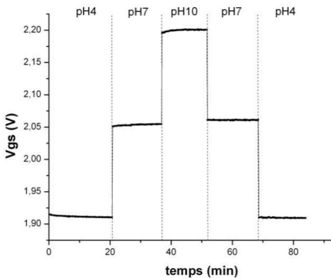
Figure 21: Tension de sortie du capteur en fonction du temps pour différentes valeurs de pH
