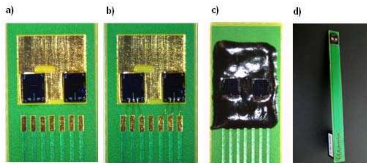
Figure 16: Etape d'encapsulations a) collage, b) microsoudures, c) englobage, d) connectique
