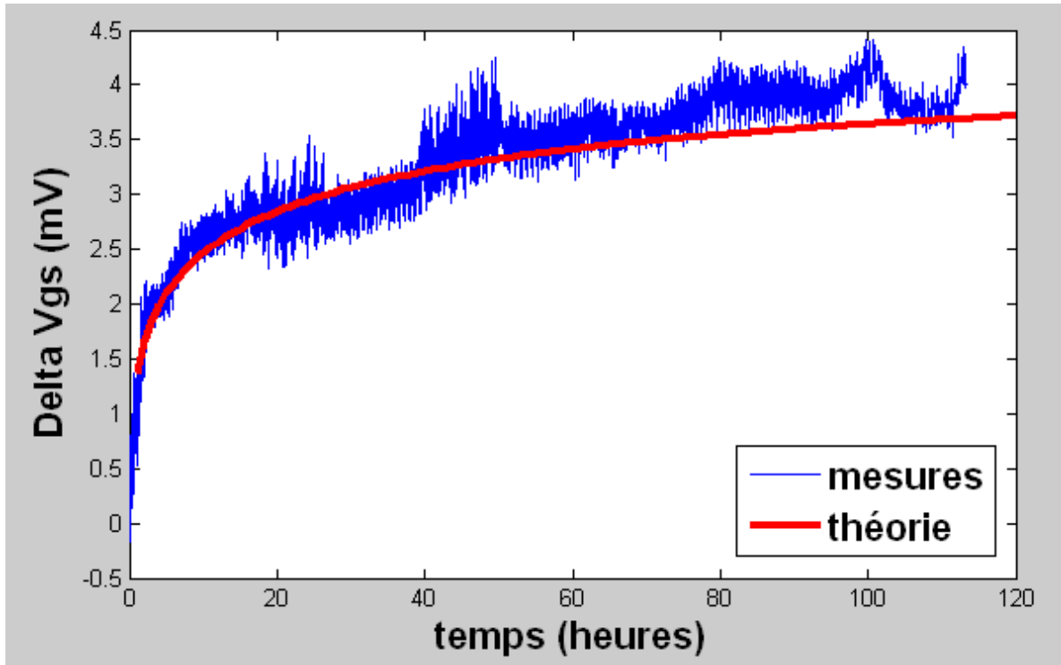
Figure 27: Modélisation de la dérive
