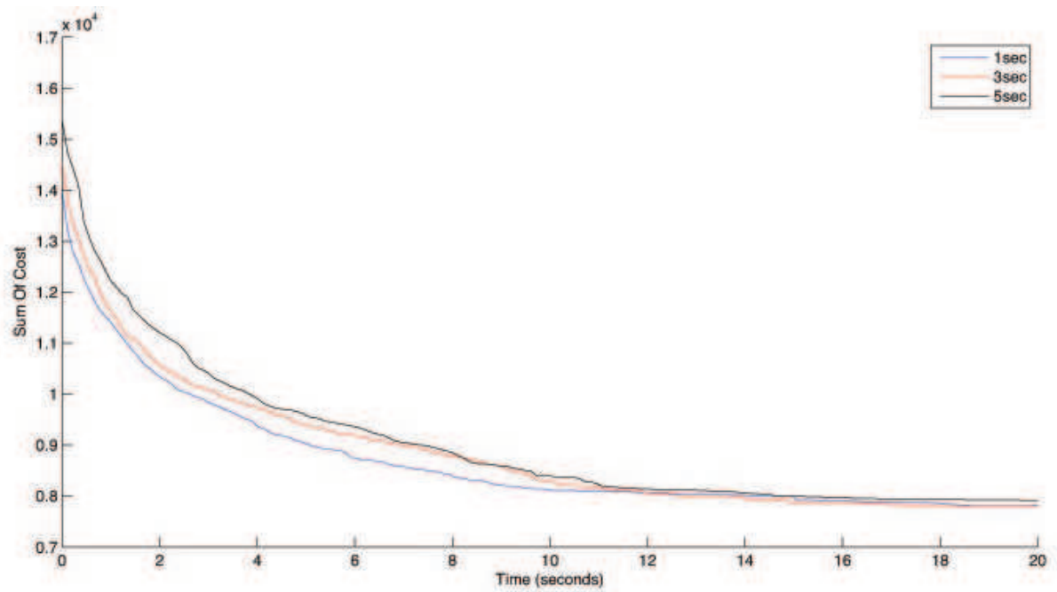
(a) Convergence sur l'exemple PR2 simple
