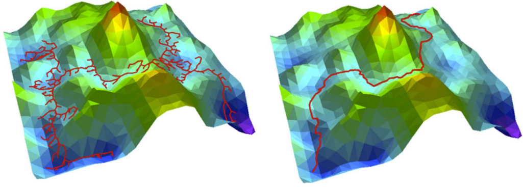
FIGURE 3.2 – T-RRT développé sur une carte de coût 2D (à gauche). Le test de transition favorise l'exploration des régions de bas coût, résultant en un chemin de bonne qualité (à droite).
