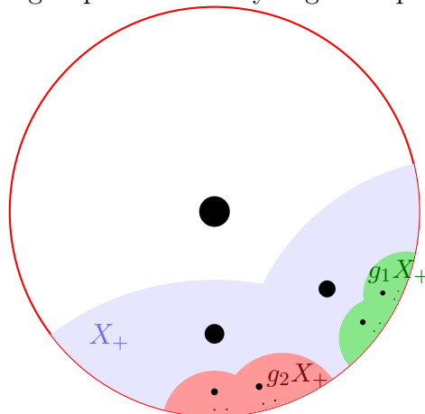
FIGURE II.12 – Un semi-groupe de Schottky engendré par deux isométries g_1 et g_2
