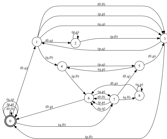
P = 1 et Q = X^2
