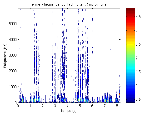
Figure 107 : Représentation temps-fréquence du signal vibratoire obtenu sur un panneau (spectrogramme).
