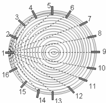
Figure 109 : Schéma d'un essai de tomographie en géométrie éventail.
