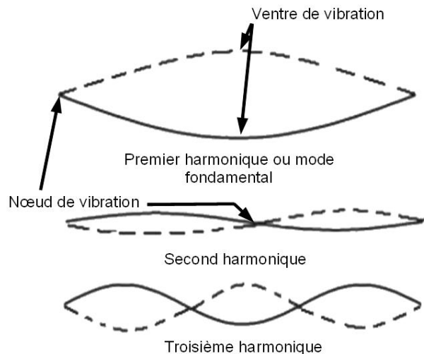
Figure 12 : Déformée d'une poutre en vibration de flexion selon la fréquence de résonance.
