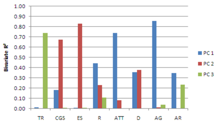
Figure 78 : Coefficient de détermination bivarié entre paramètres et CPs (N=300).
