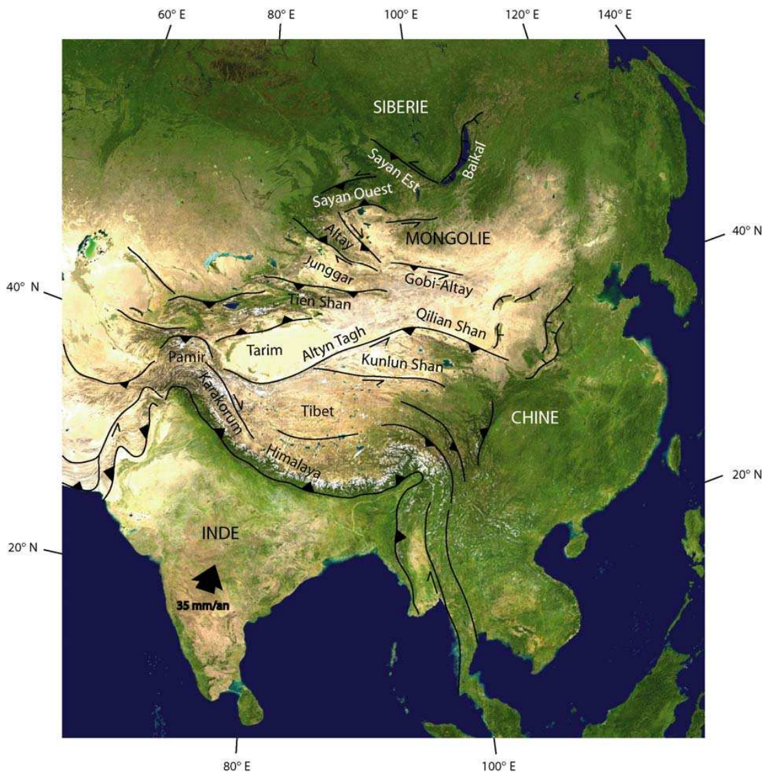
FIG. 4.1: Carte tectonique simplifiée, tirée de Vassalo (2006), avec les principales failles et chaînes de montagnes associées à la collision Inde - Asie. La convergence entre l'Inde et la Sibirie est donnée par le GPS (Bettinelli et al. , 2006).
