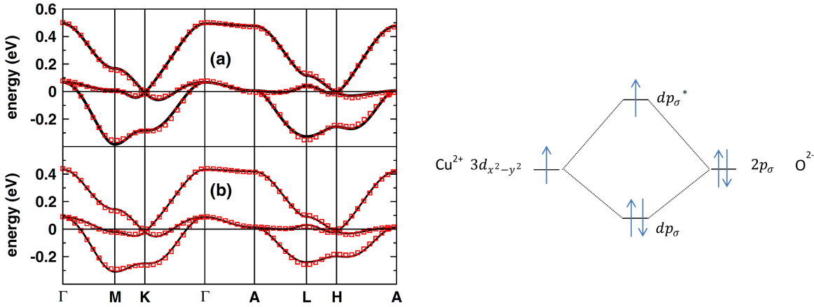
FIGURE 6.7 – Gauche : Structure de bandes (lignes) établie par DFT de la kapellasite (a) et de l’haydéite (b), extrait de [178]. Les carrés rouges représentent l’ajustement des bandes d’énergie obtenues dans le cadre d’un modèle de liaisons fortes. Droite : Diagramme de liaison moléculaire entre un ion \text{Cu}^{2+} et un ion \text{O}^{2-} . Les bandes qui croisent le niveau de Fermi sont notées dp_{\sigma}^* .
