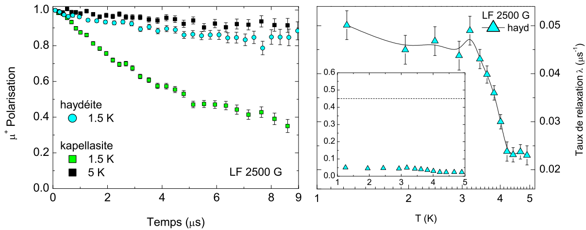
FIGURE 9.12 – Gauche : Comparaison de la relaxation pour la kapellasite et l'haydéite sous 2500 G. Pour T \geq 4 K, les relaxations sont similaires alors qu'à T = 1.5 K celle dans la kapellasite est nettement supérieure. Droite : Dépendance en température du taux de relaxation de l'haydéite pour H_{LF} = 2500 G. Insert : Comparaison entre le taux de relaxation de la kapellasite dans le régime basse température (ligne pointillée) et celui de l'haydéite (triangles bleus).
