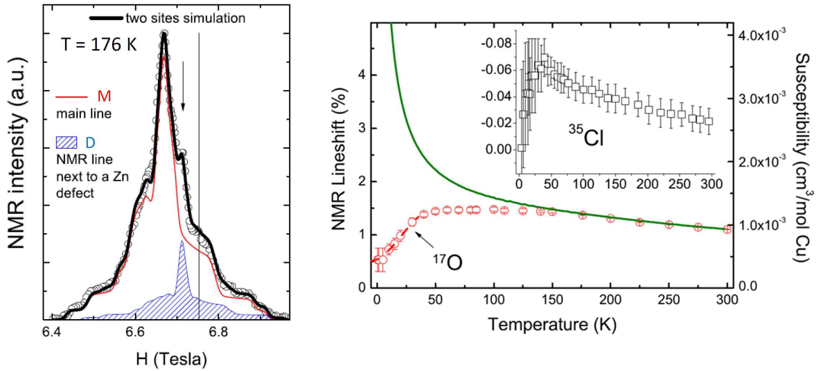
FIGURE 2.4 – Gauche : Spectre RMN d' ^{17}\text{O} dans l'herbertsmithite à T = 176 K. Il peut être simulé par deux contributions, une majoritaire M (rouge) et une minoritaire D (bleue). Droite : Comparaison de la dépendance en température de la susceptibilité locale RMN (points rouges) et macroscopique SQUID (ligne verte). Insert : Susceptibilité locale RMN mesurée à partir de la sonde ^{35}\text{Cl} .
