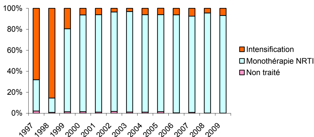
Figure 3.5 : Evolution des traitements prophylactiques administrés aux nouveau-nés entre 1997 et 2009 (EPF)
